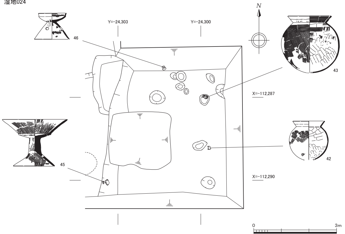
图10 湿地023·024遺物出土狀況图 (1 : 80)
