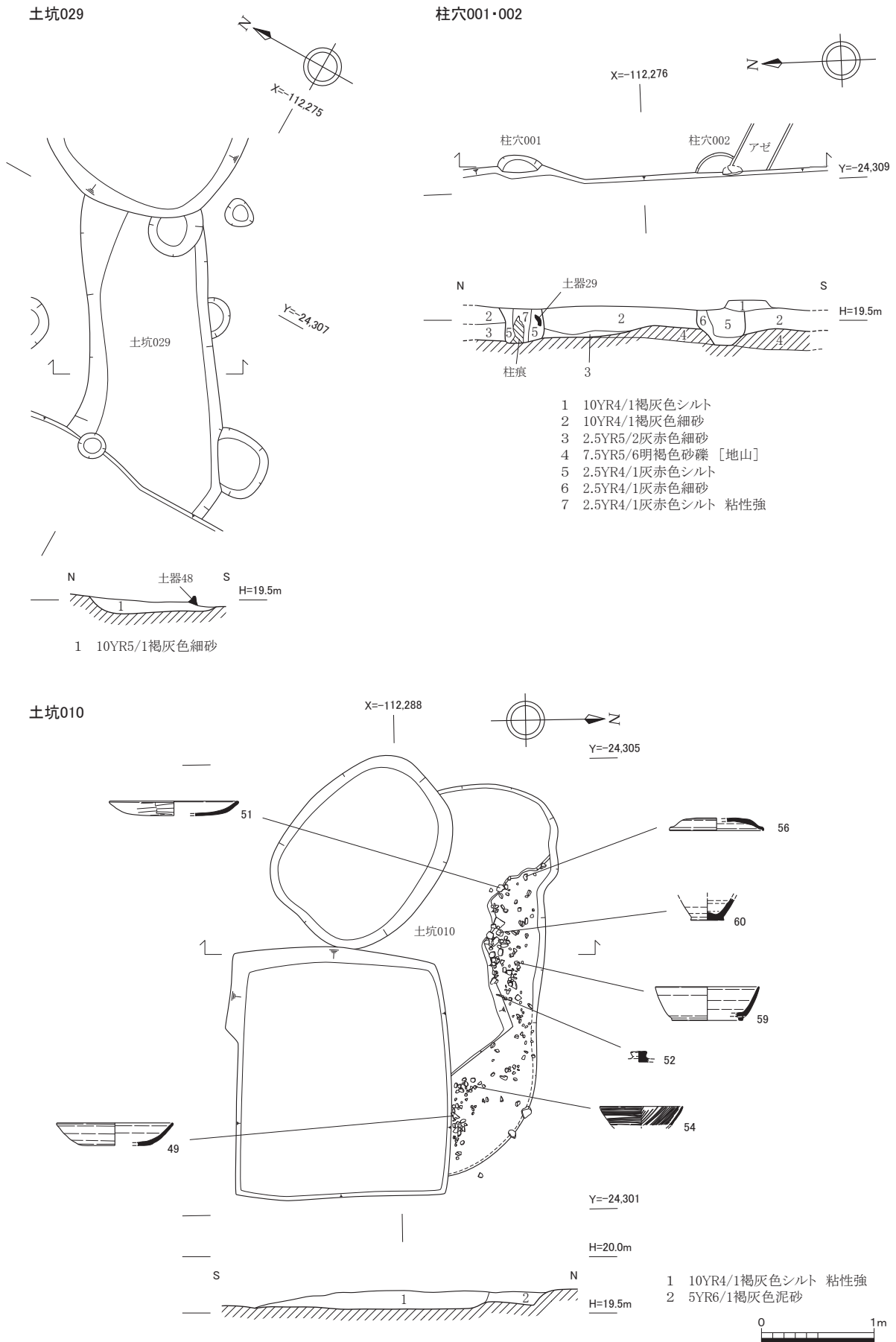
図14 土坑029、柱穴001・002、土坑010平面・断面図（1：50）
