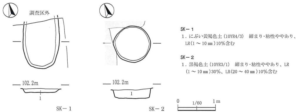
第10図 SK-1・SK-2遺構平・断面図
