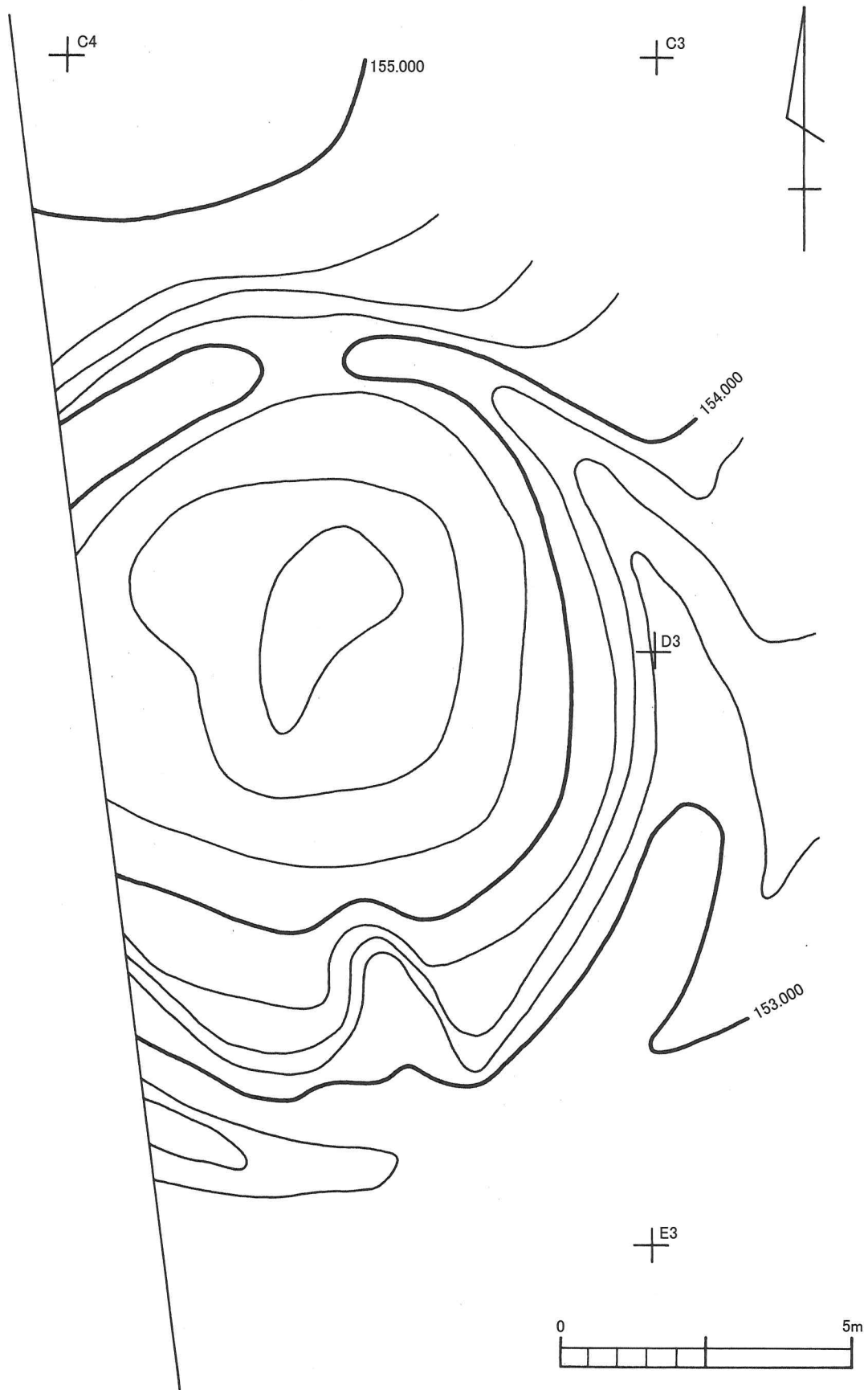
第12図 大塚古墳群 2号墳測量図
