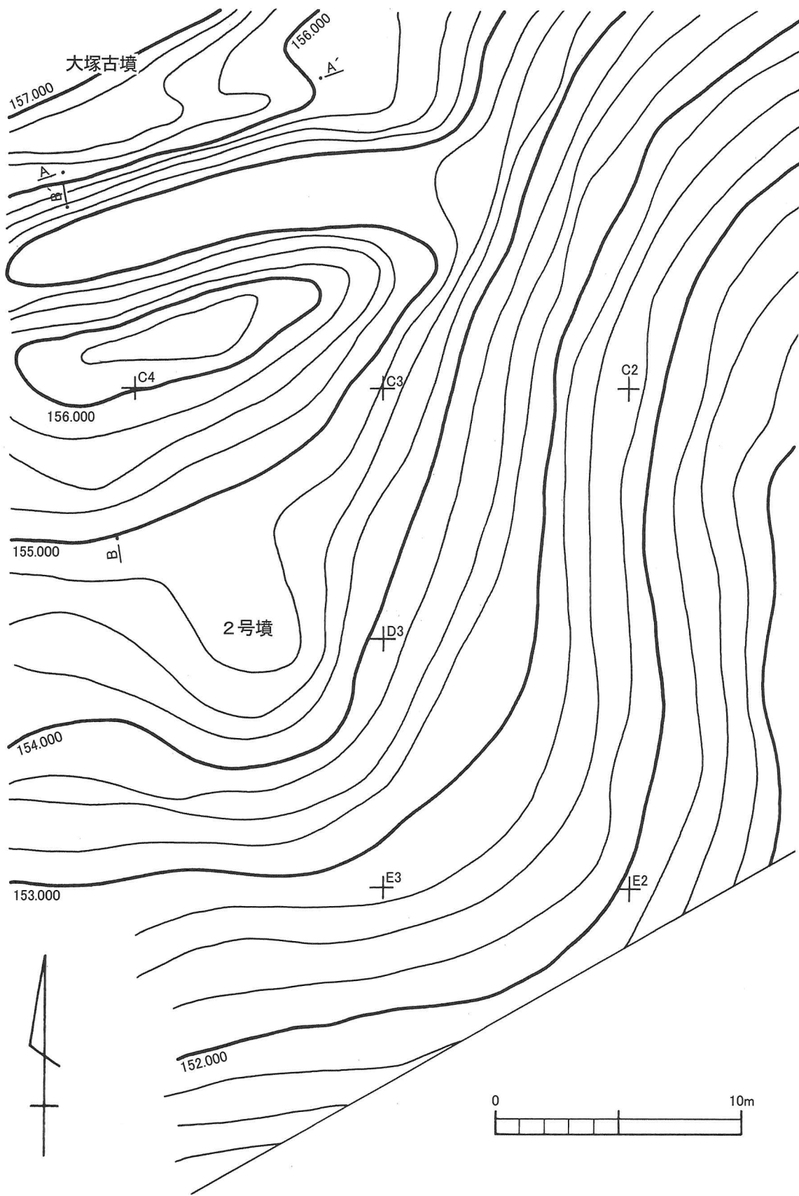
第10図 大塚古墳群測量図
