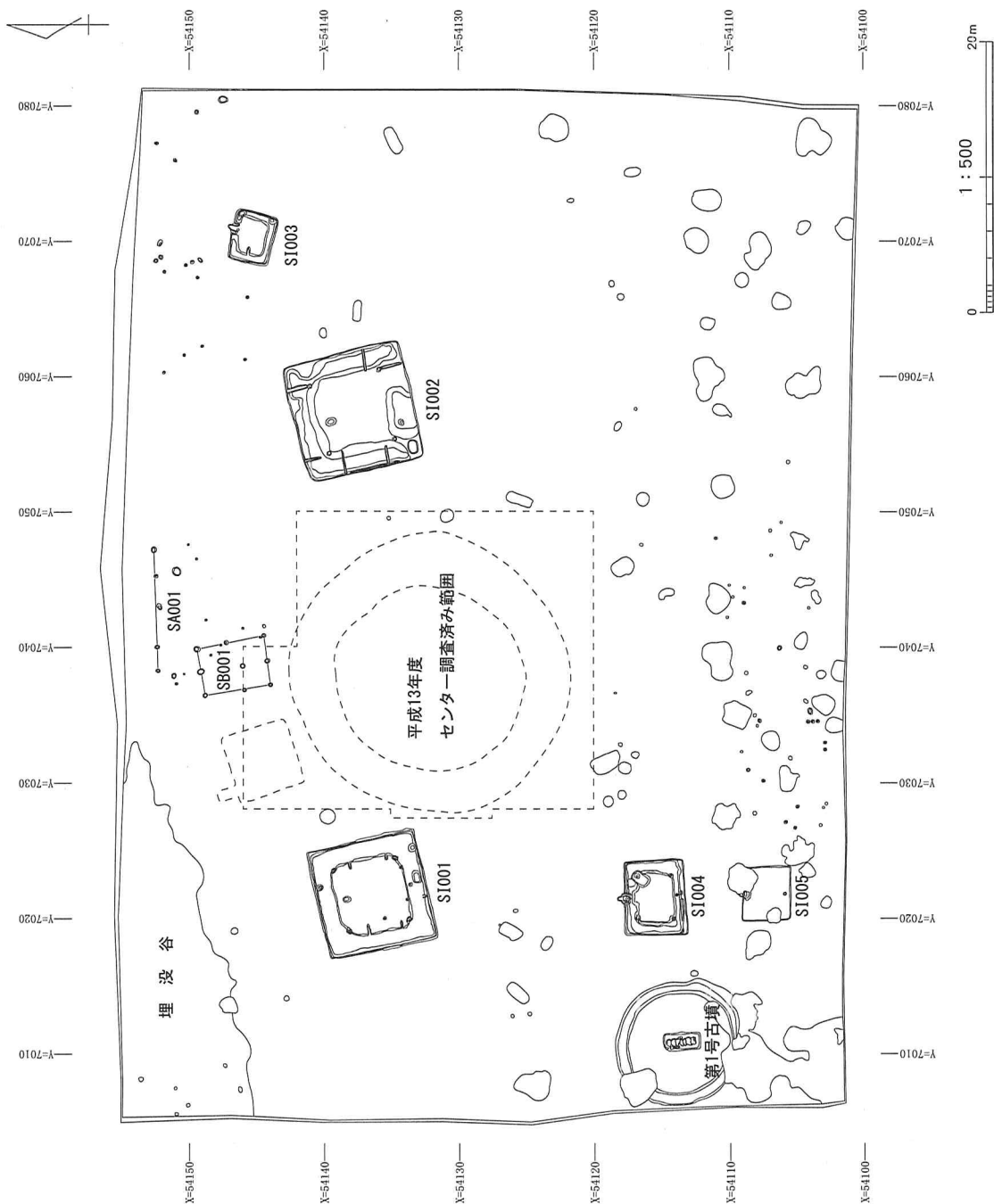
図4 遺構配置図
