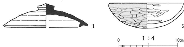
図21 第5号竪穴住居SI005遺物実測図
