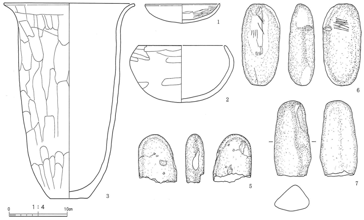
図16 第3号竖穴住居SI003遺物実測図
