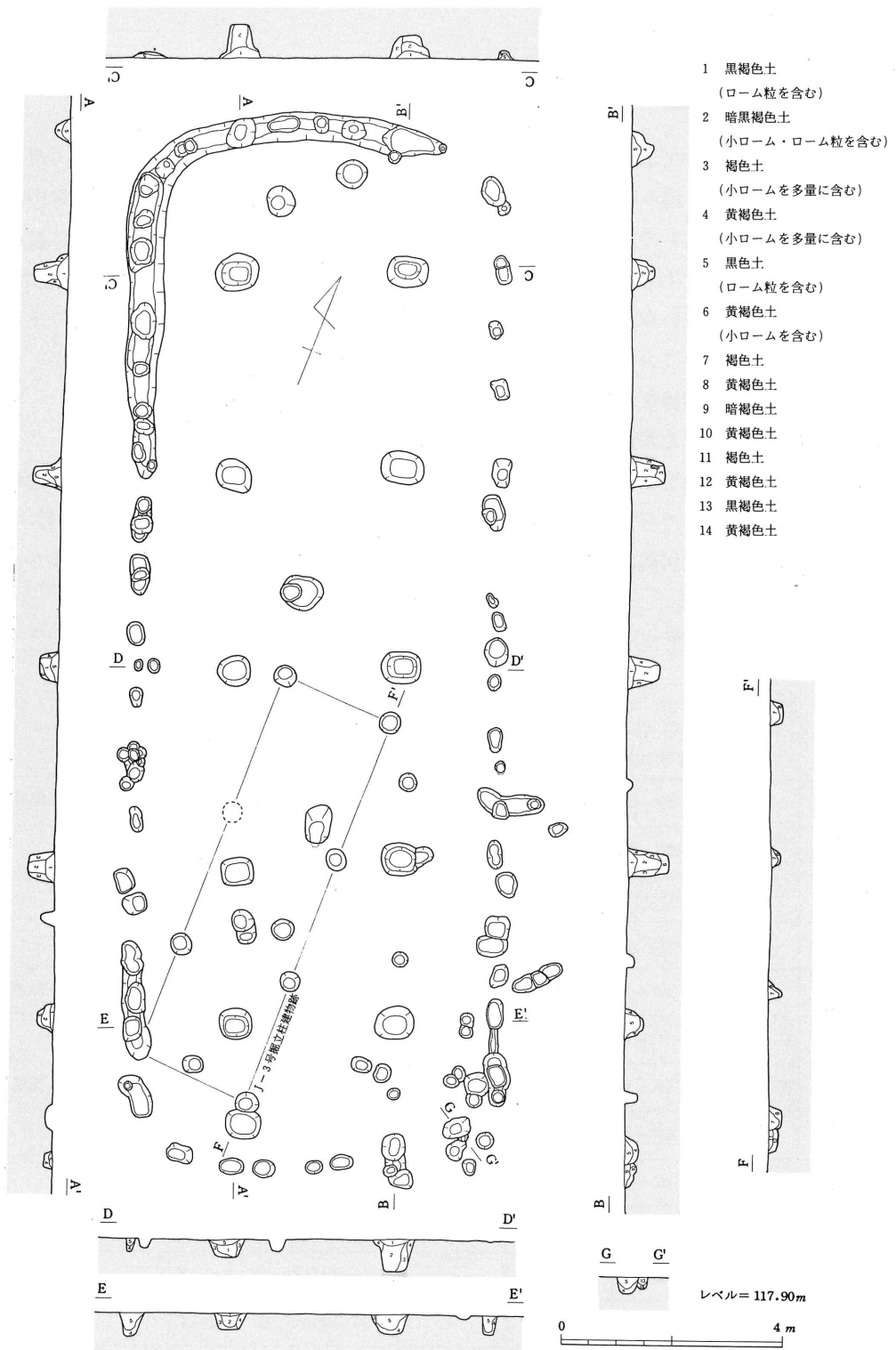
第9図 3号長方形大型建物跡実測図
