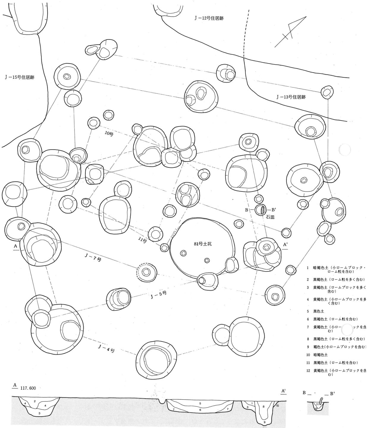
第11図 J-4～7号掘立柱建物跡実測図
