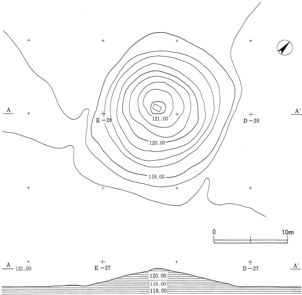
第4図 將軍塚古墳墳丘測量図
