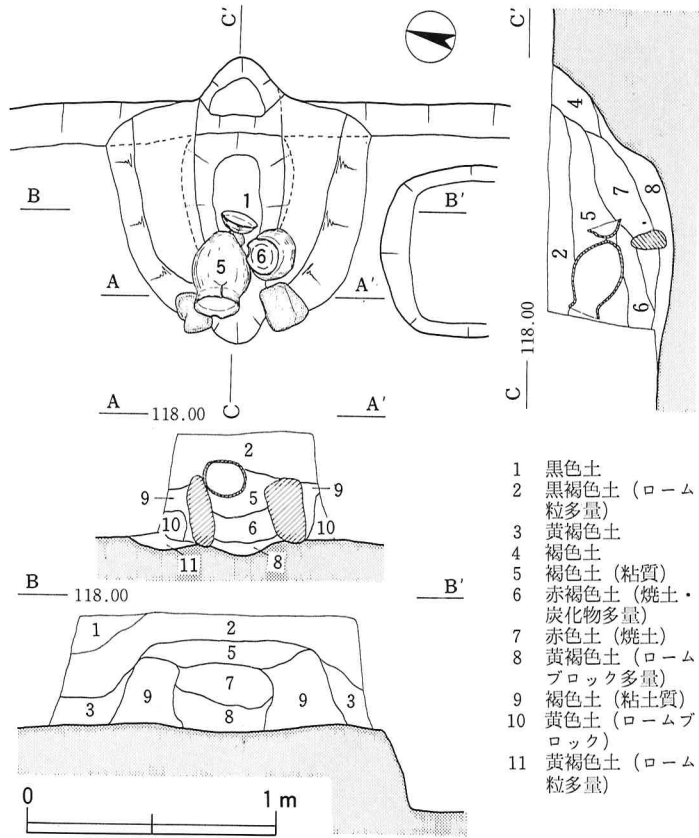
第17図 30号住居跡カマド実測図
