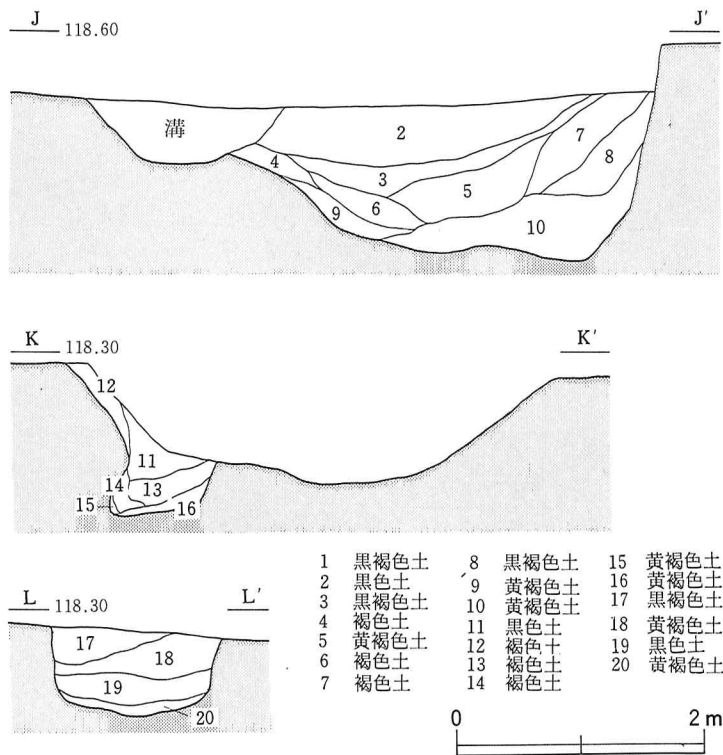
第9図 將軍塚古墳土坑断面図(上 土坑6, 中 土坑5, 下 土坑9)
