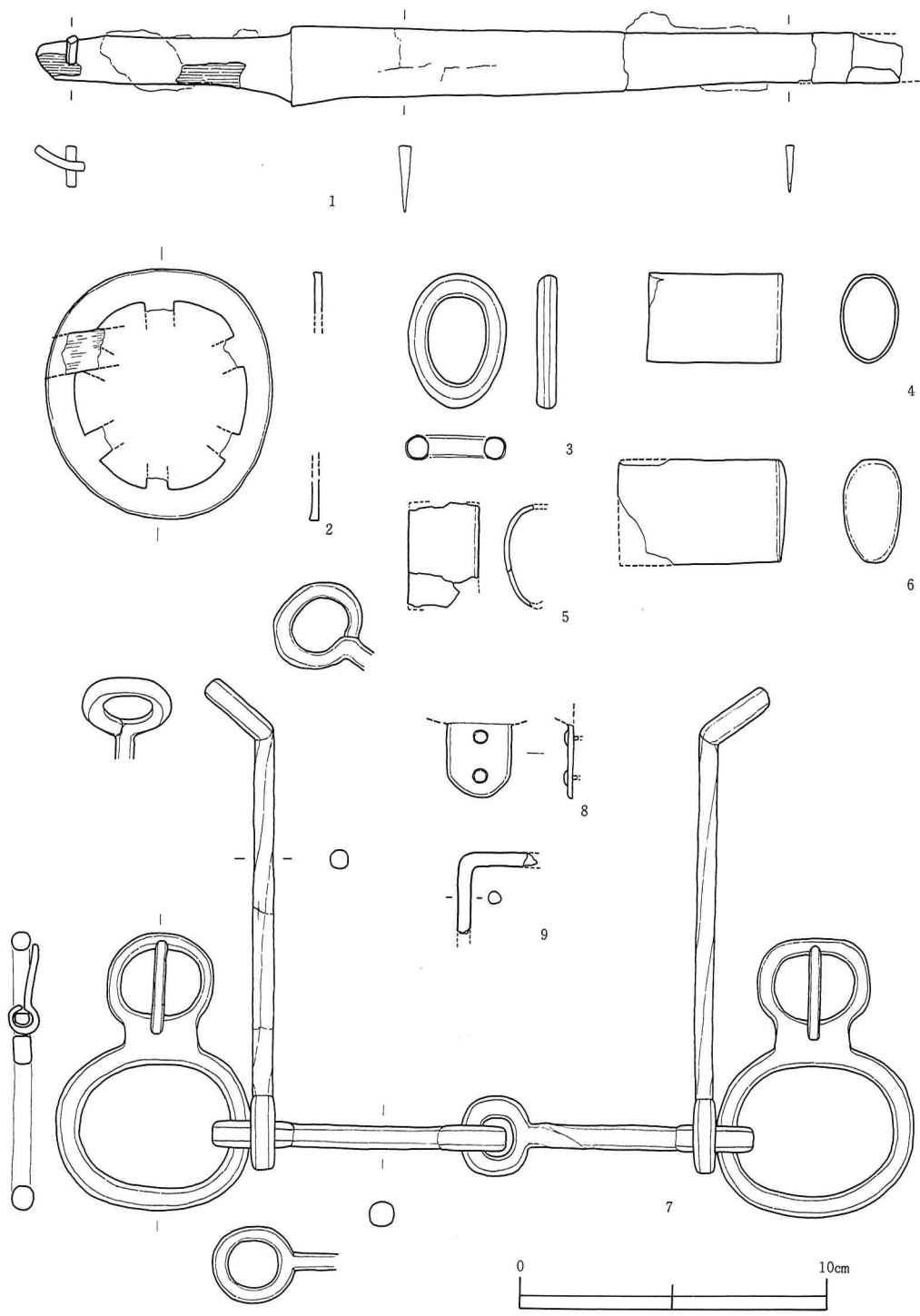
第16图 聖山公園6号墳出土鉄器実測図(1)
