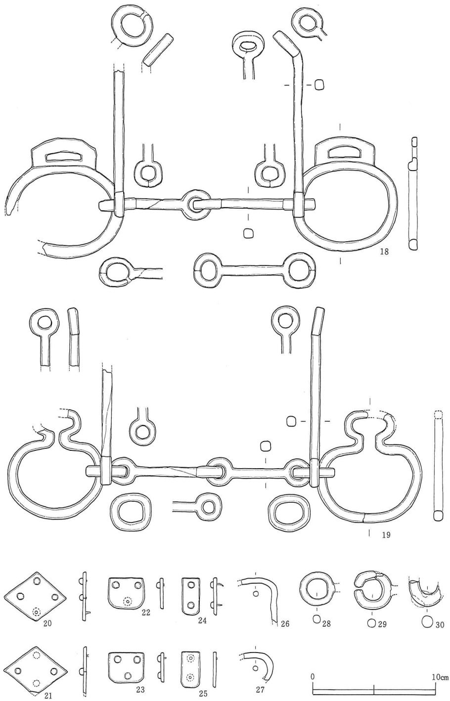
第20图 瓦塚古墳群中出土鉄器実測図(2)
