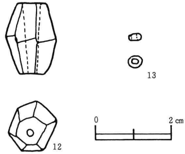
第18図 聖山公園 6号墳出土玉類実測図
