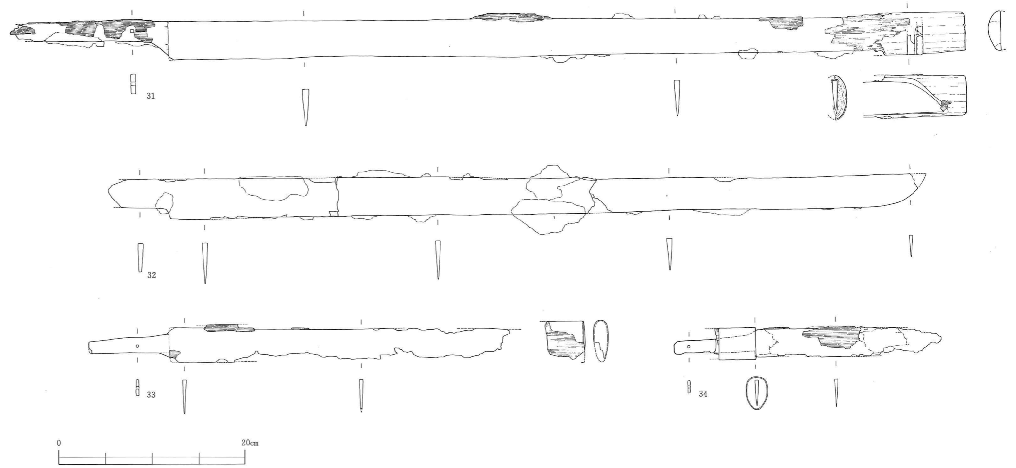
第21图 瓦塚古墳群中出土鉄器実測図(3)
