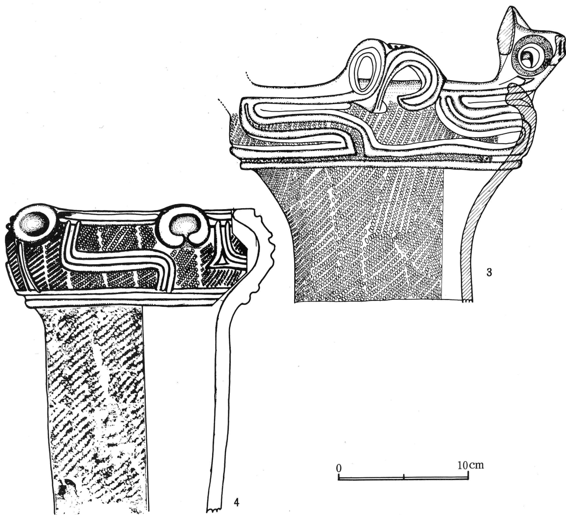
2号土器ブロック実測図 No.2
