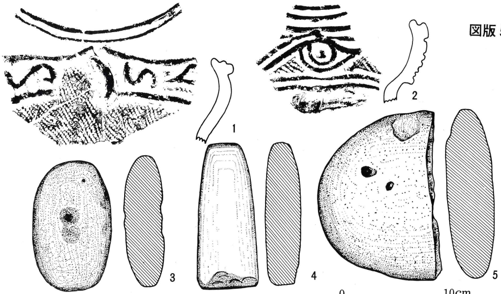
0 10cm P-1 実測図 No.3
