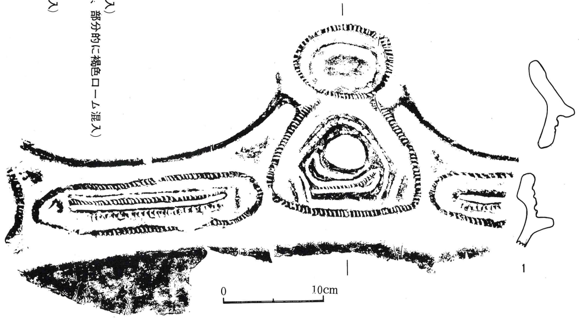
P-16実測図 No.1
