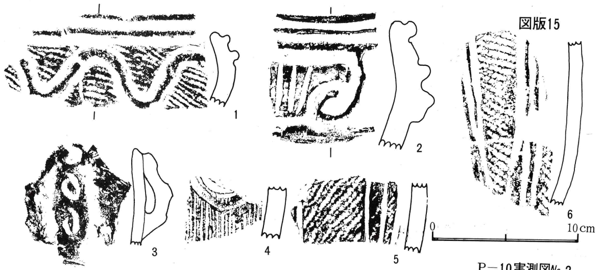
P-10実測図No. 2
