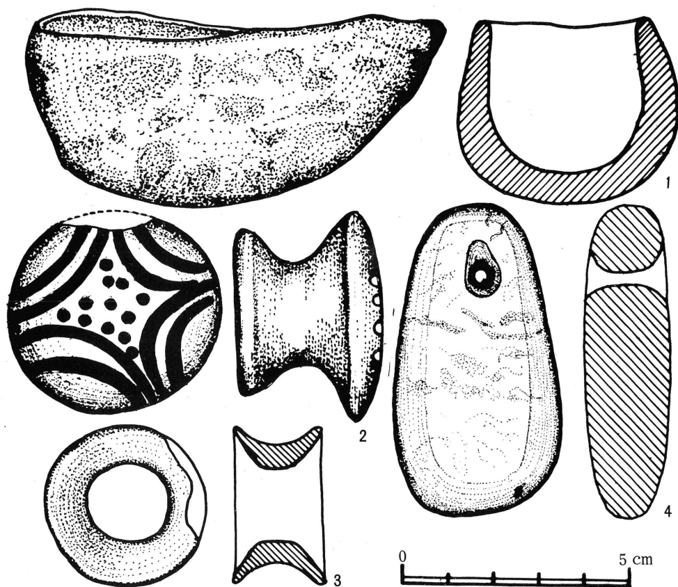
A区出土遗物实测图
