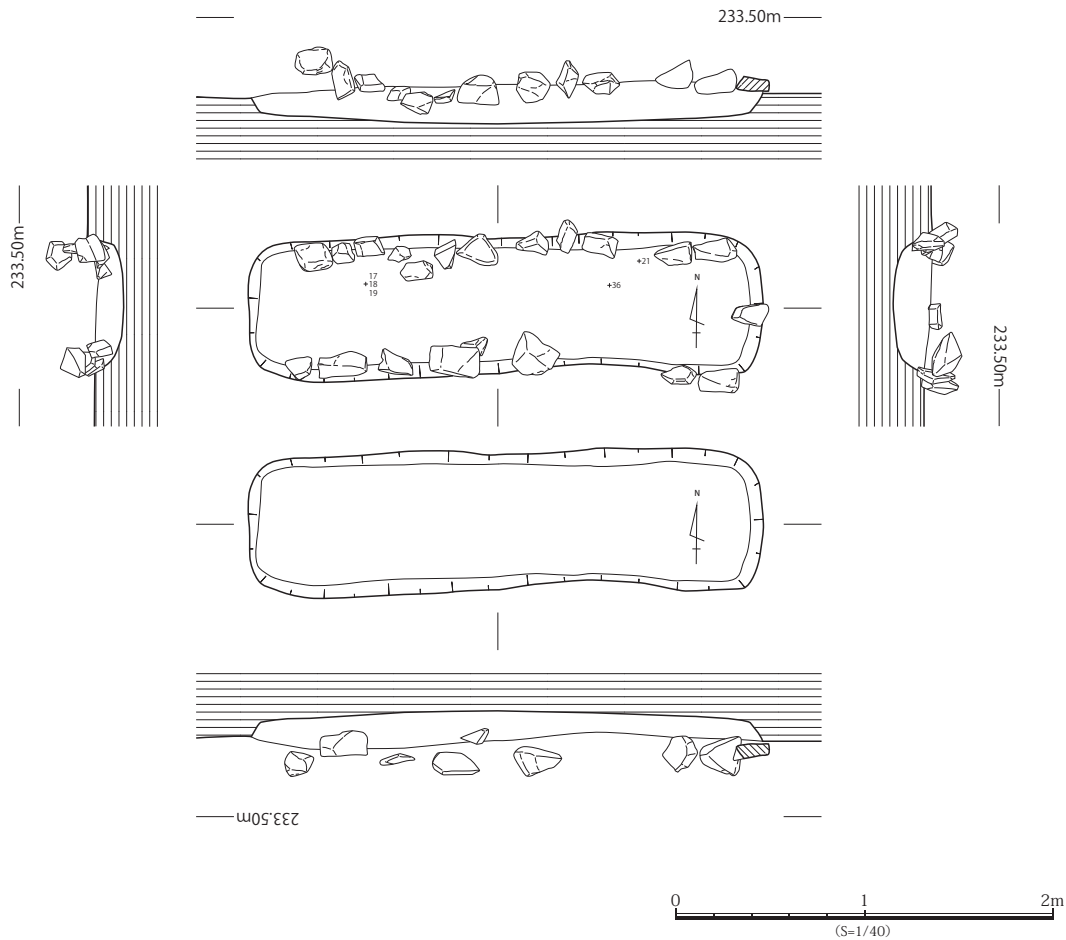
第14図 第8号古墳第2主体部実測図(1:40)
