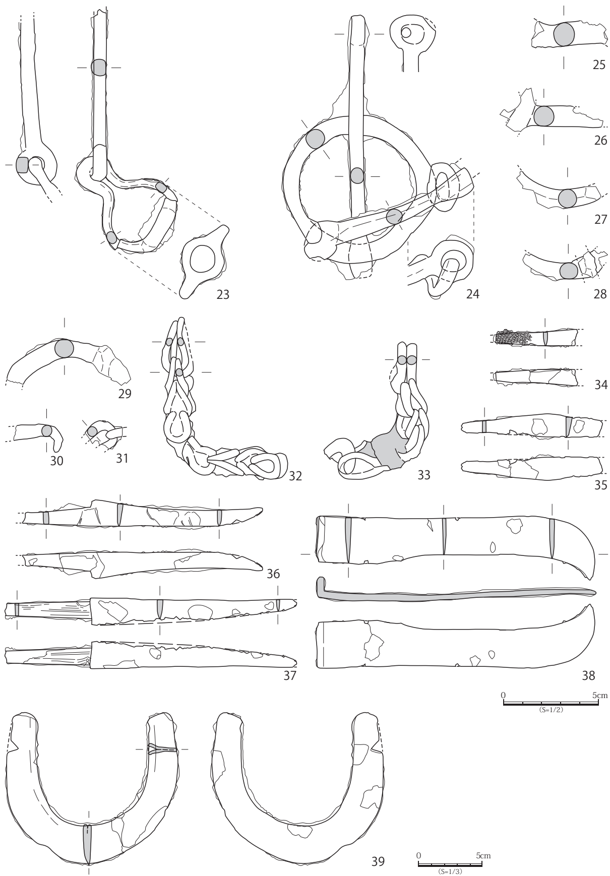
第16图 第8号古墳出土遺物実測図(2)(1:2、1:3)
