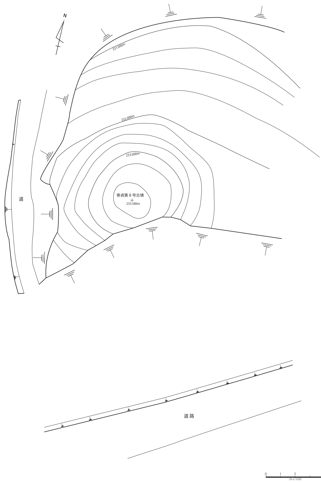
第10図 第8号古墳調査前地形測量図(1:150)
