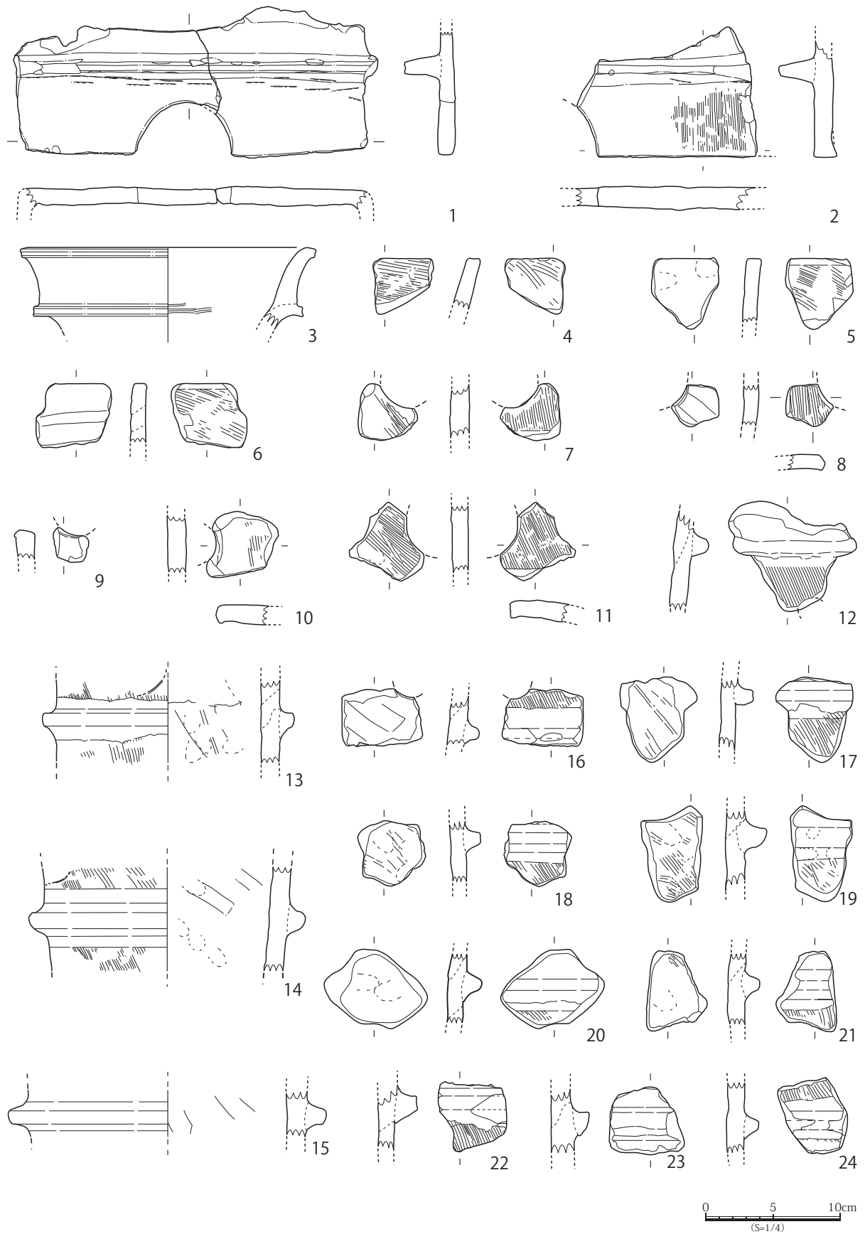
第8图 第7号古墳出土遺物実測図(1)(1:4)
