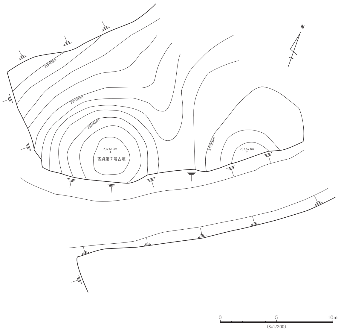
第4図 第7号古墳調査前地形測量図(1:200)
