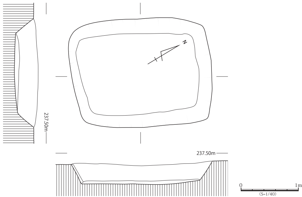
第7図 第7号古墳主体部実測図(1:40)
