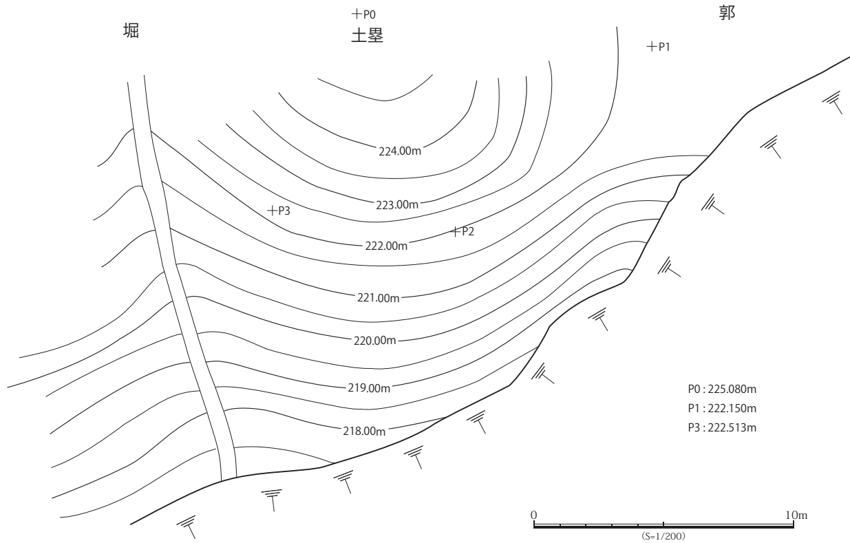
第17図 寄貞城跡地形測量図(1:200)
