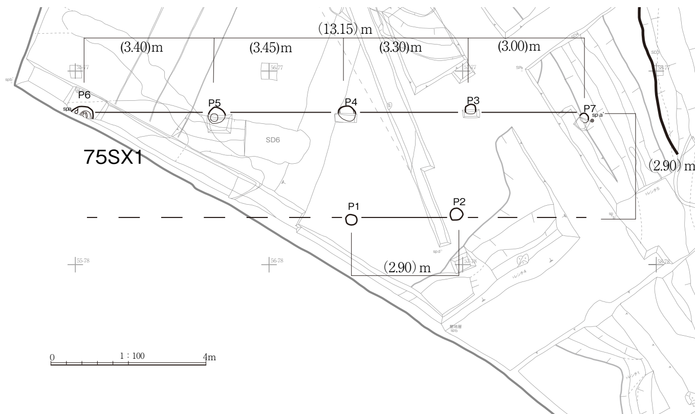
図43 75SX1平面図
