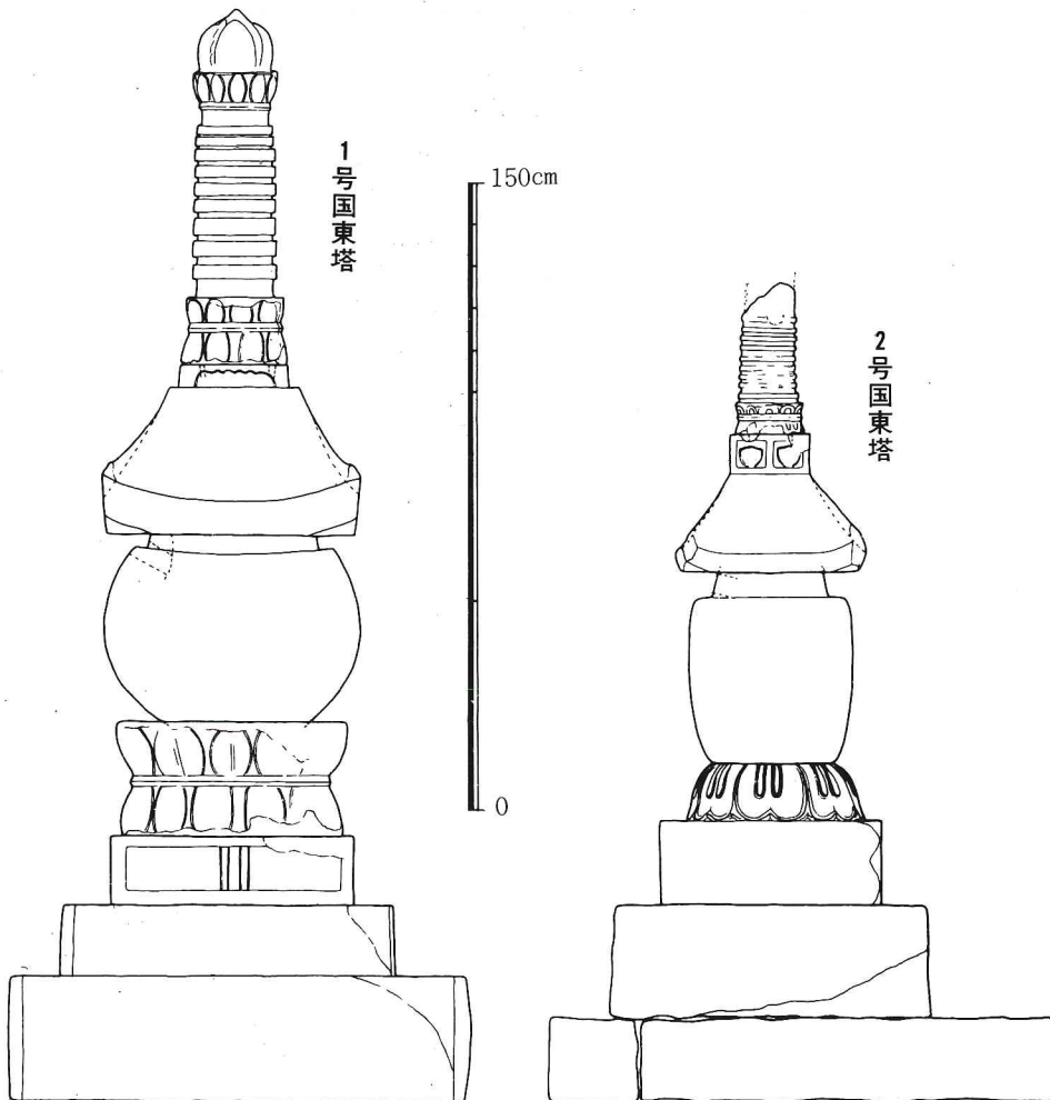
第8図 万福寺国東塔実測図
