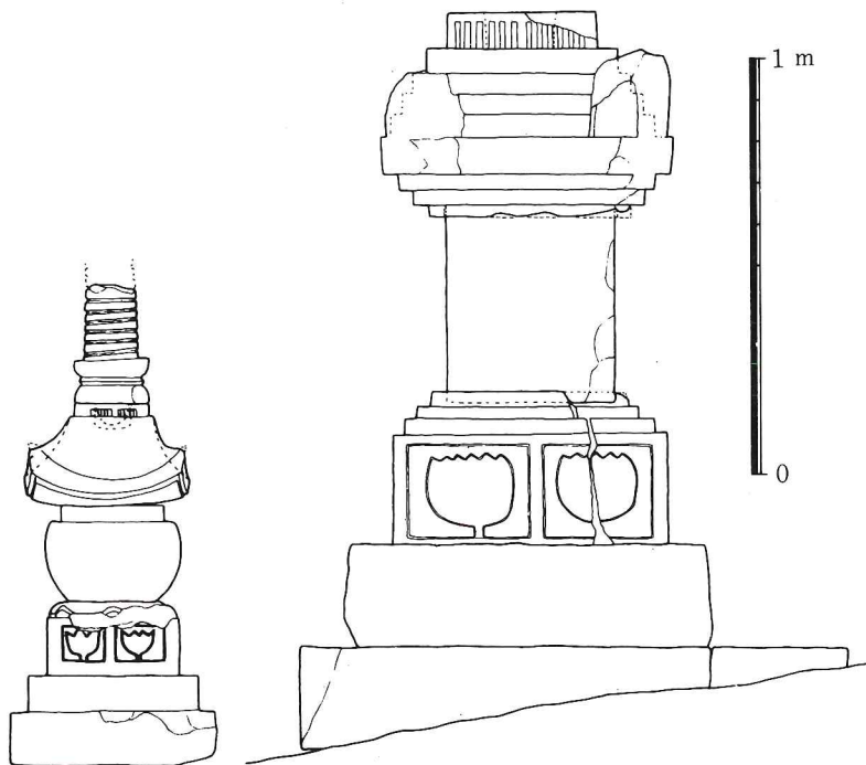
第11図 成仏寺阿弥陀堂周辺石塔実測図
