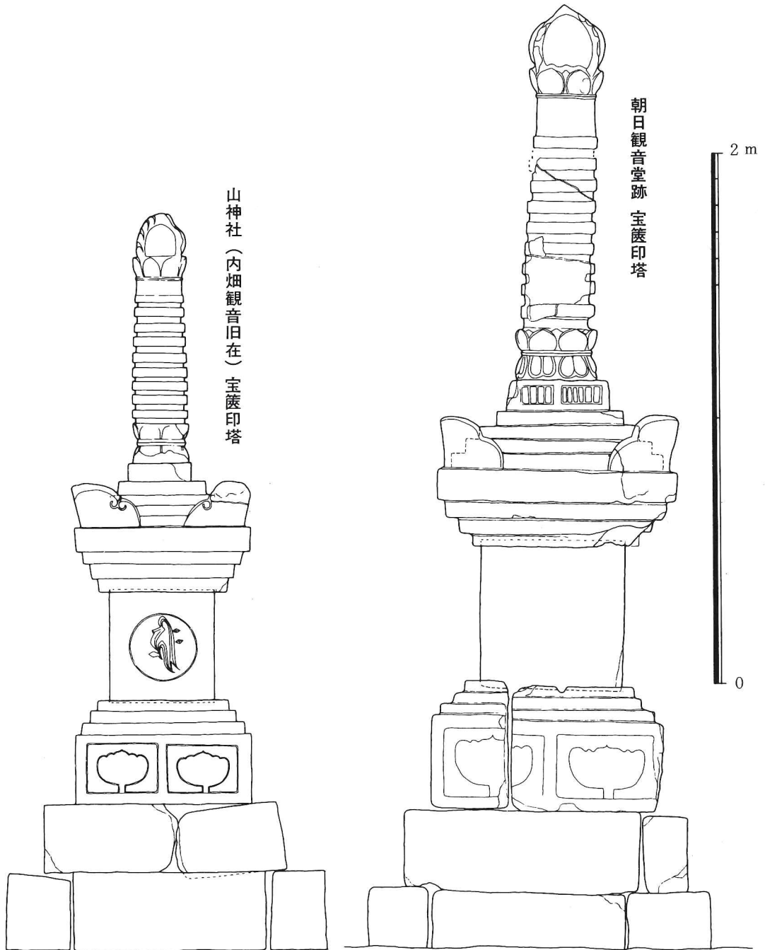
第12図 成仏寺周辺宝篋印塔実測図
