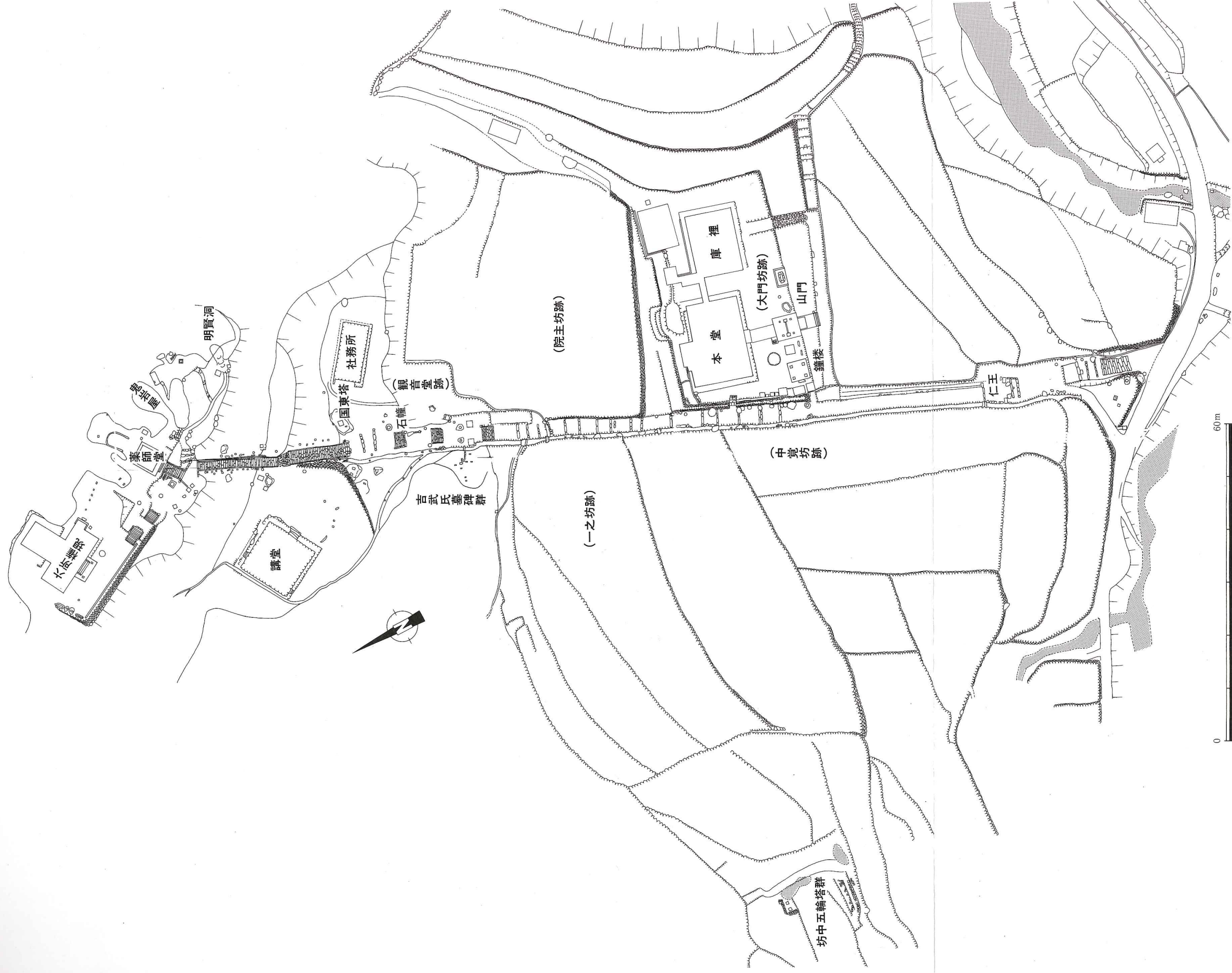
第17図 石立山岩戸寺周辺地形測量図
