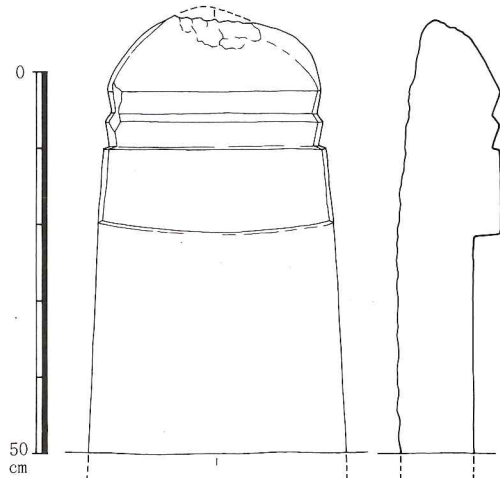
第7図 真木大堂古代公園円板碑実測図
