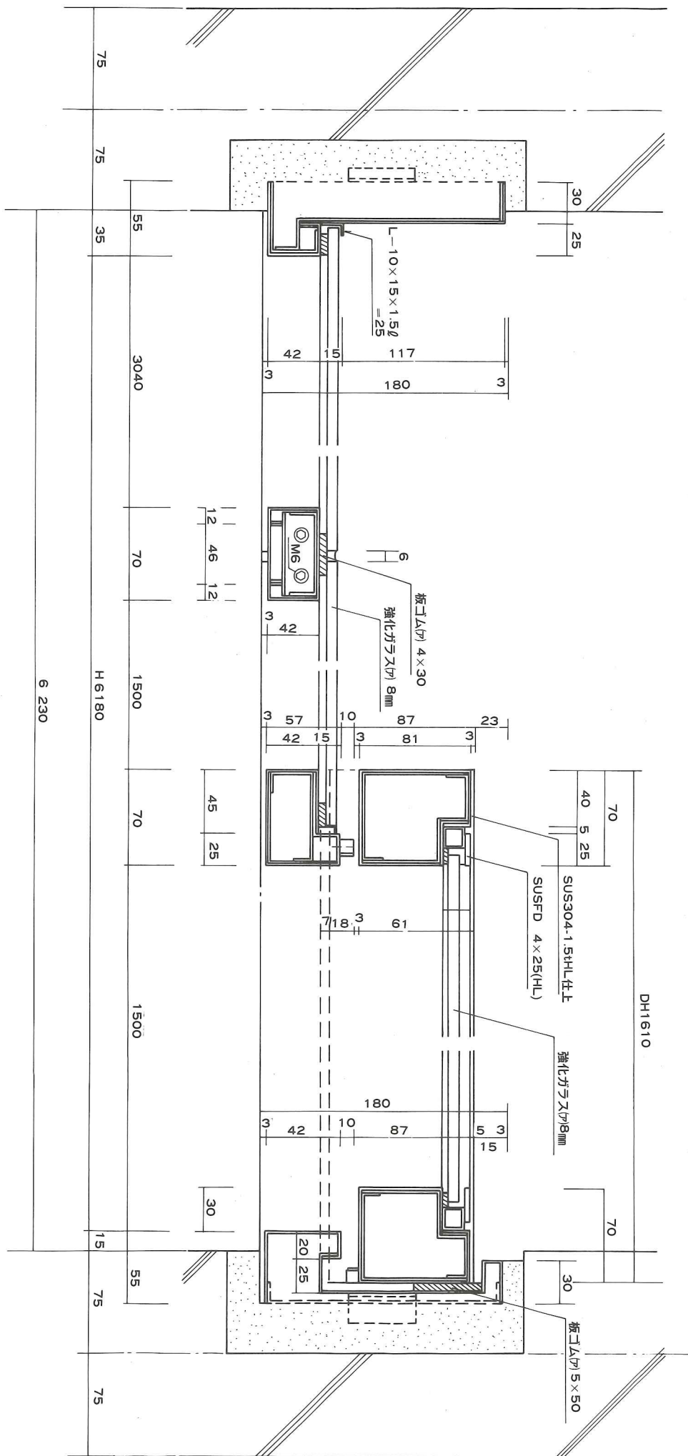
第38図 覆屋建具詳細図 (1)
