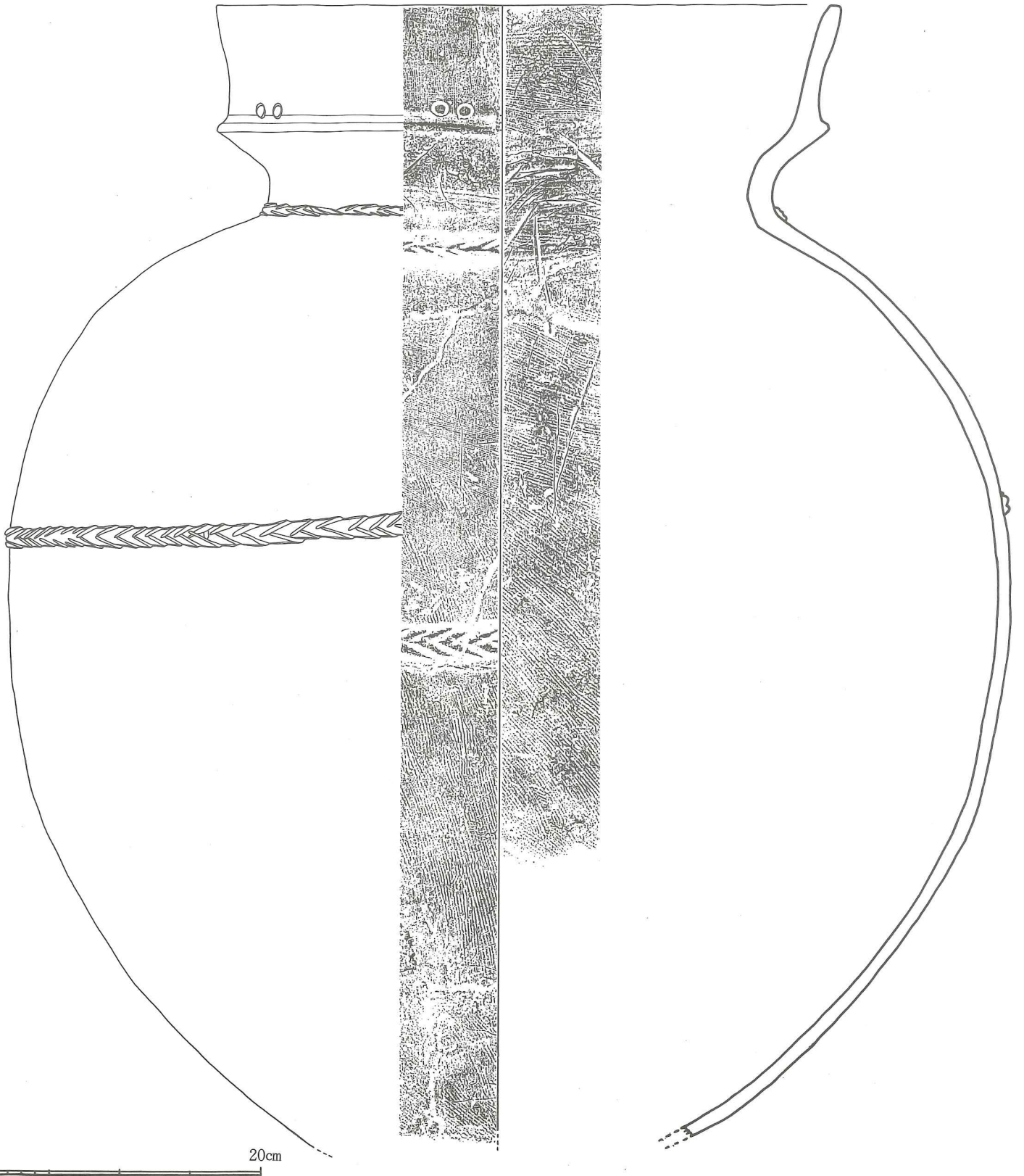
第27图 壺棺实测图
