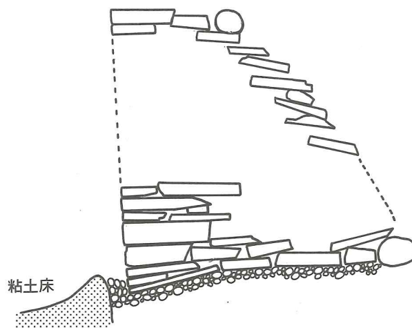
第12図 竪穴式石室構造模式図
