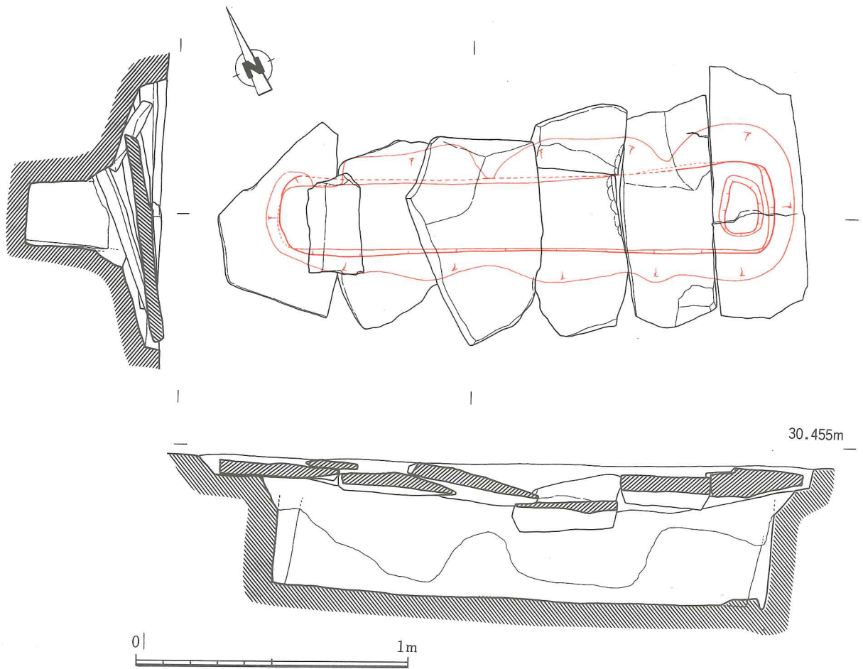
第24図 方形周溝墓主体部 (石蓋土塚墓)
