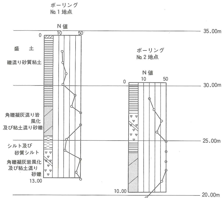
第32図 地層想定図・標準貫入N値
