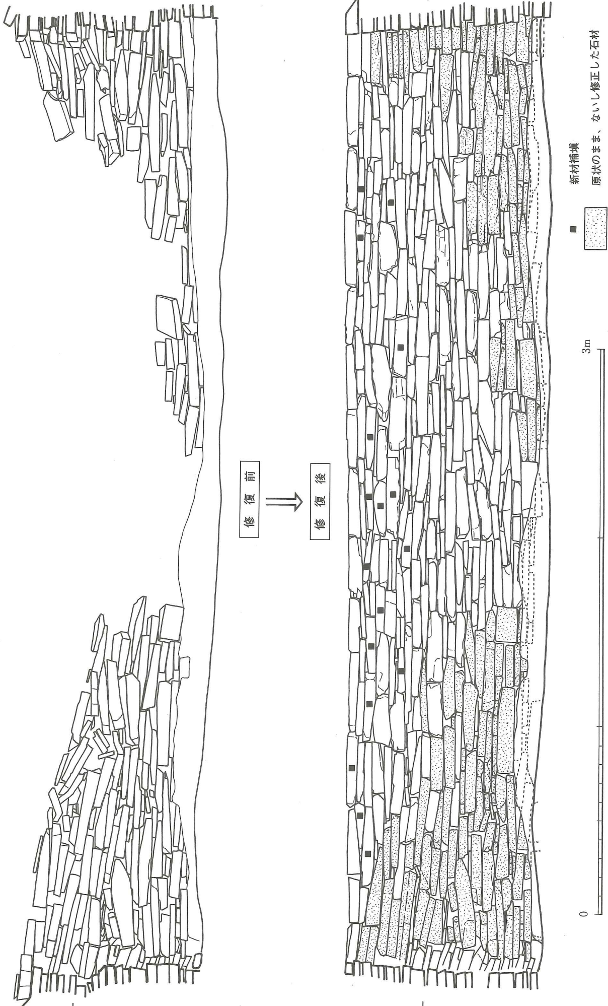
第45図 竪穴式石室の修復（1）北長側壁
