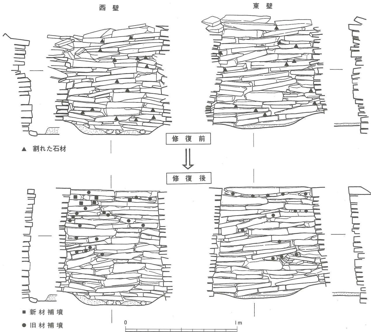
第47図 竪穴式石室の修復（3）短側壁
