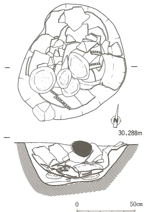
第26図 壺棺出土状態
