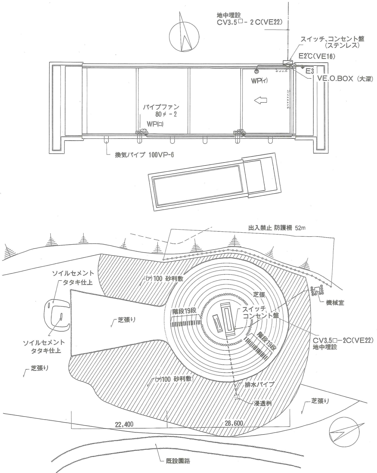
第40図 電気設備
