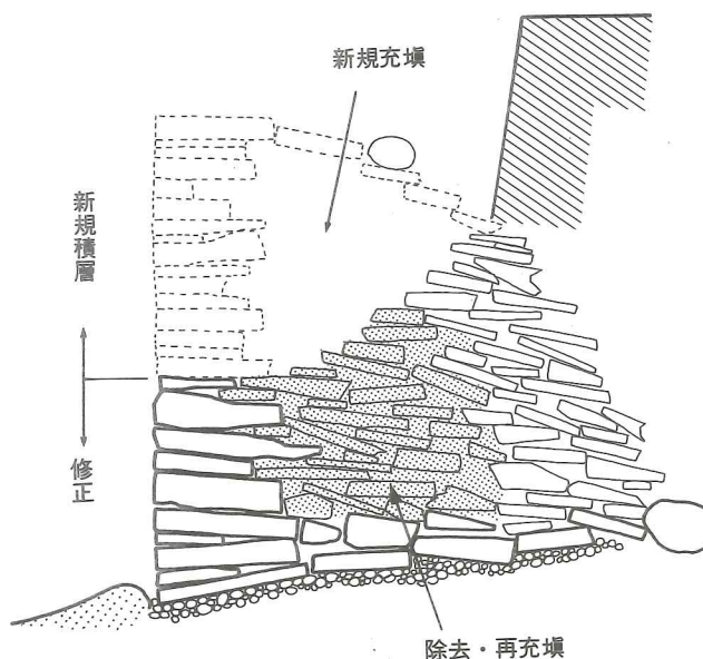
第41図 石室の修復模式図
