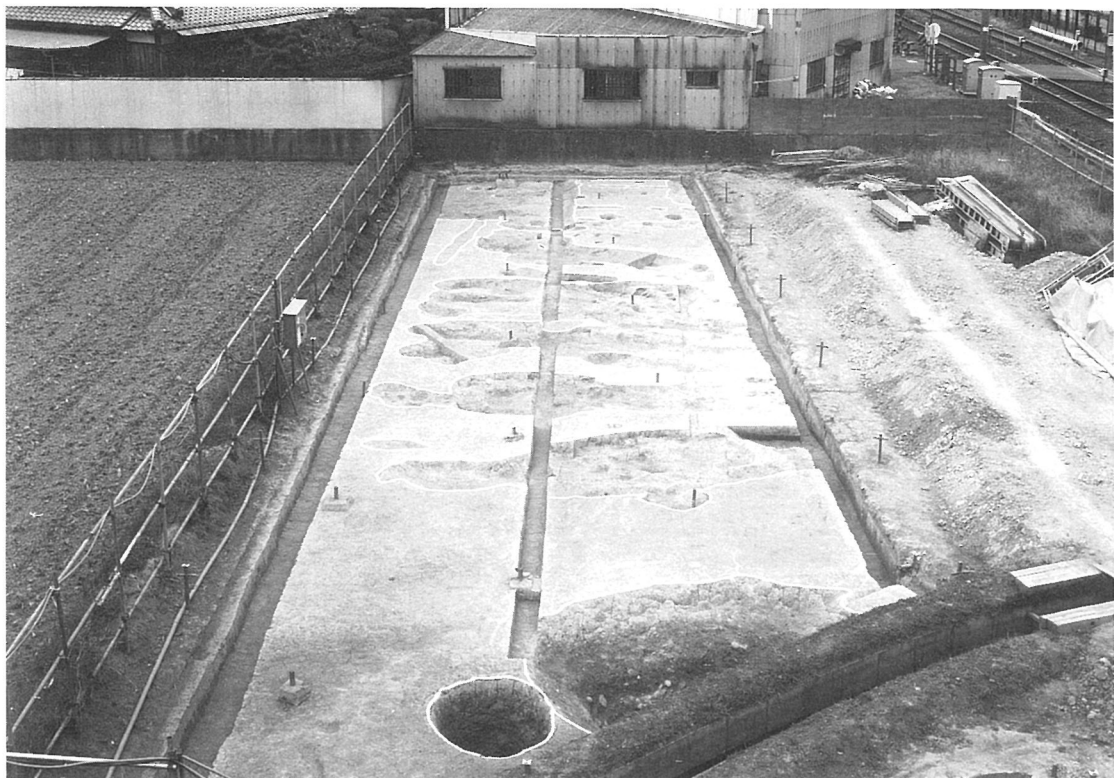
A-1区遺構検出状況（南西から）
