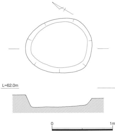
第16図 土壙3平・断面図 (S=1/30)
