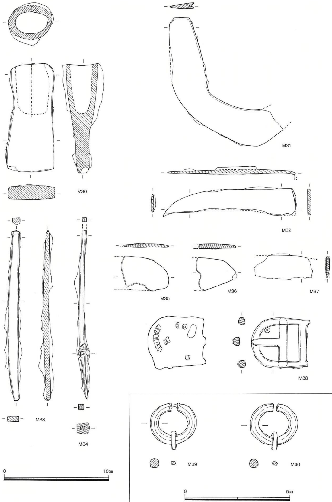
第53图 3号墳第1主体部出土遺物2 (S=1/2・1/1)
