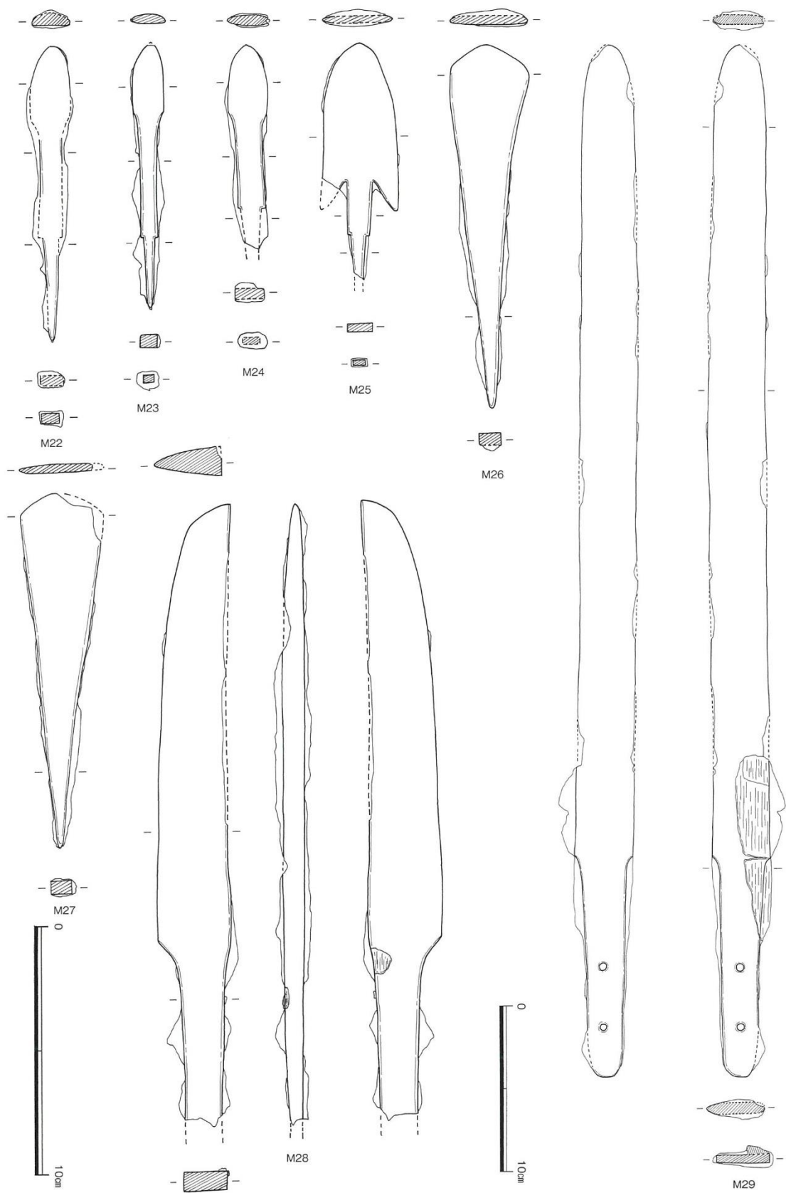
第52図 3号墳第1主体部出土遺物1 (S=1/2・1/3)
