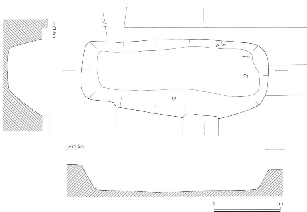
第45図 2号墳主体部平・断面図 (S=1/30)
