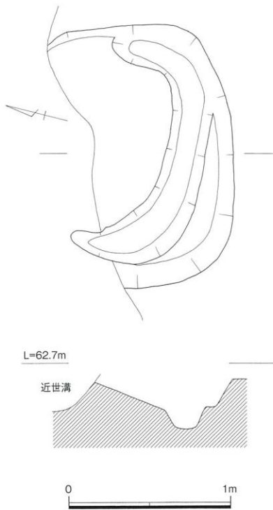
第17図 土壙4平・断面図 (S=1/30)
