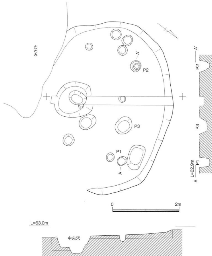
第13図 住居址4平・断面図 (S=1/60)
