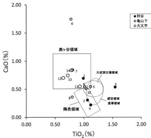
第5図 各遺跡出土須恵器の比較(TiO 2 -CaO)
