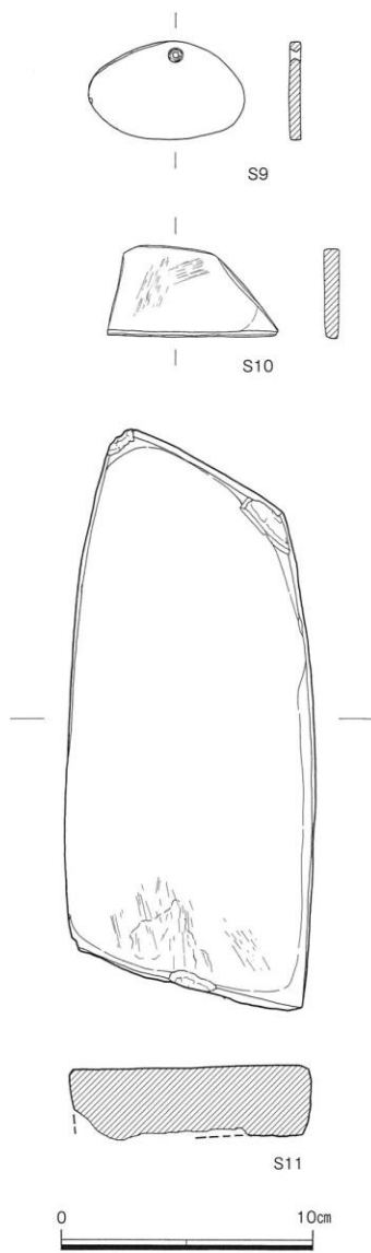
第7図 住居址1出土遺物2 (S=1/3)
