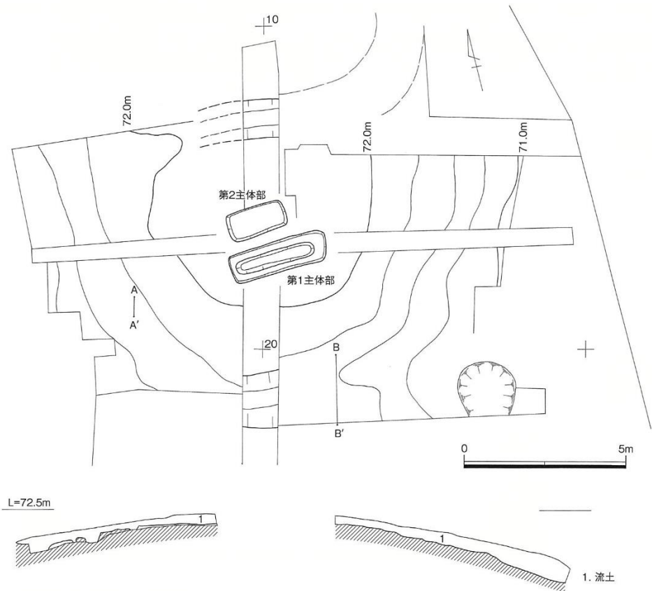
第47図 3号墳平・断面図 (S=1/150)
