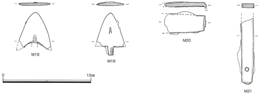
第46図 2号墳主体部出土遺物 (S=1/2)
