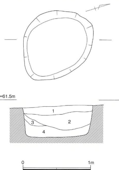
第20図 土壌6 平・断面図 (S=1/30)
