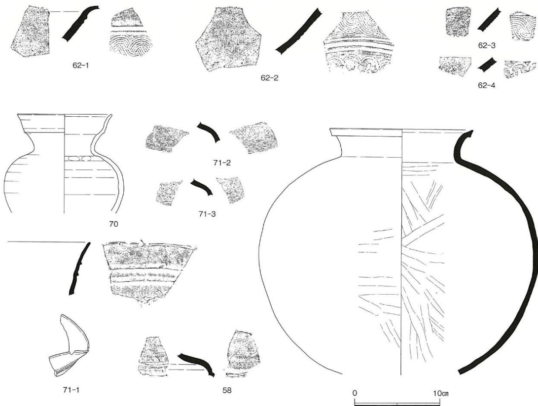
第63図 狩谷遺跡・狩谷古墳群出土初期須恵器（S=1/4）
