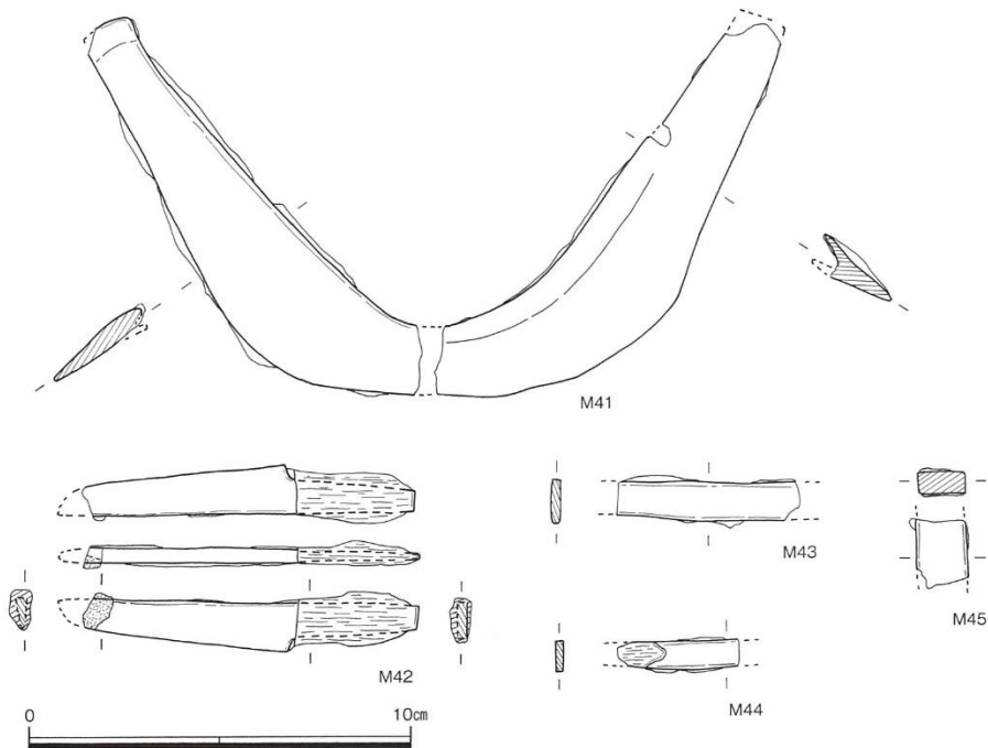
第56図 3号墳第2主体部出土遺物1 (S=1/2)
