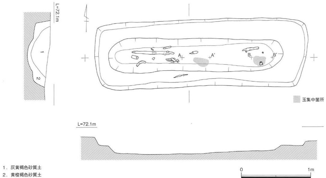
第51図 3号墳第1主体部平・断面図 (S=1/30)
