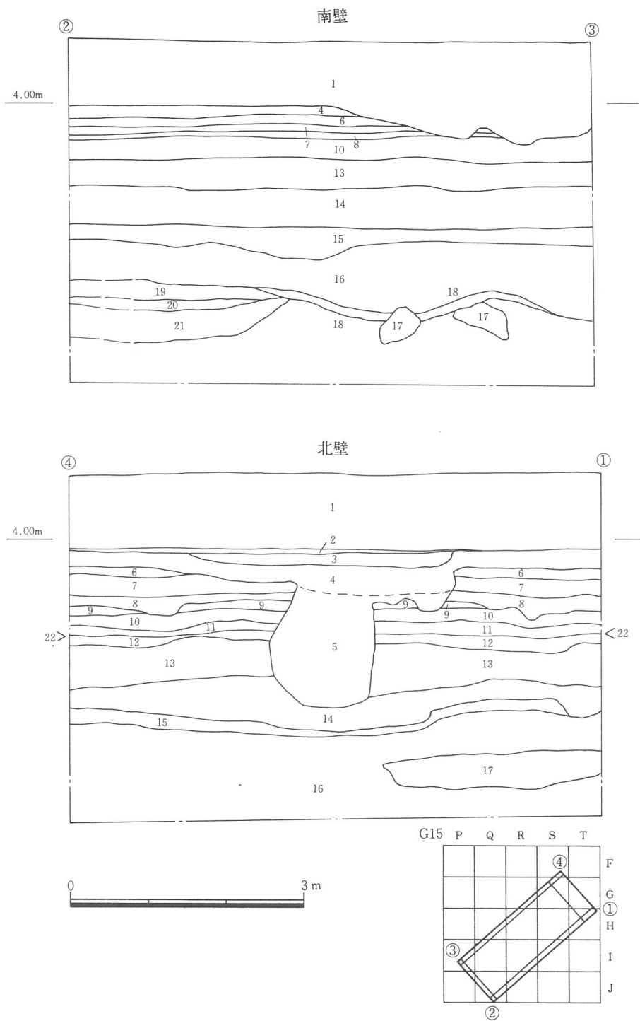
第7图 II区土层断面图(2)
