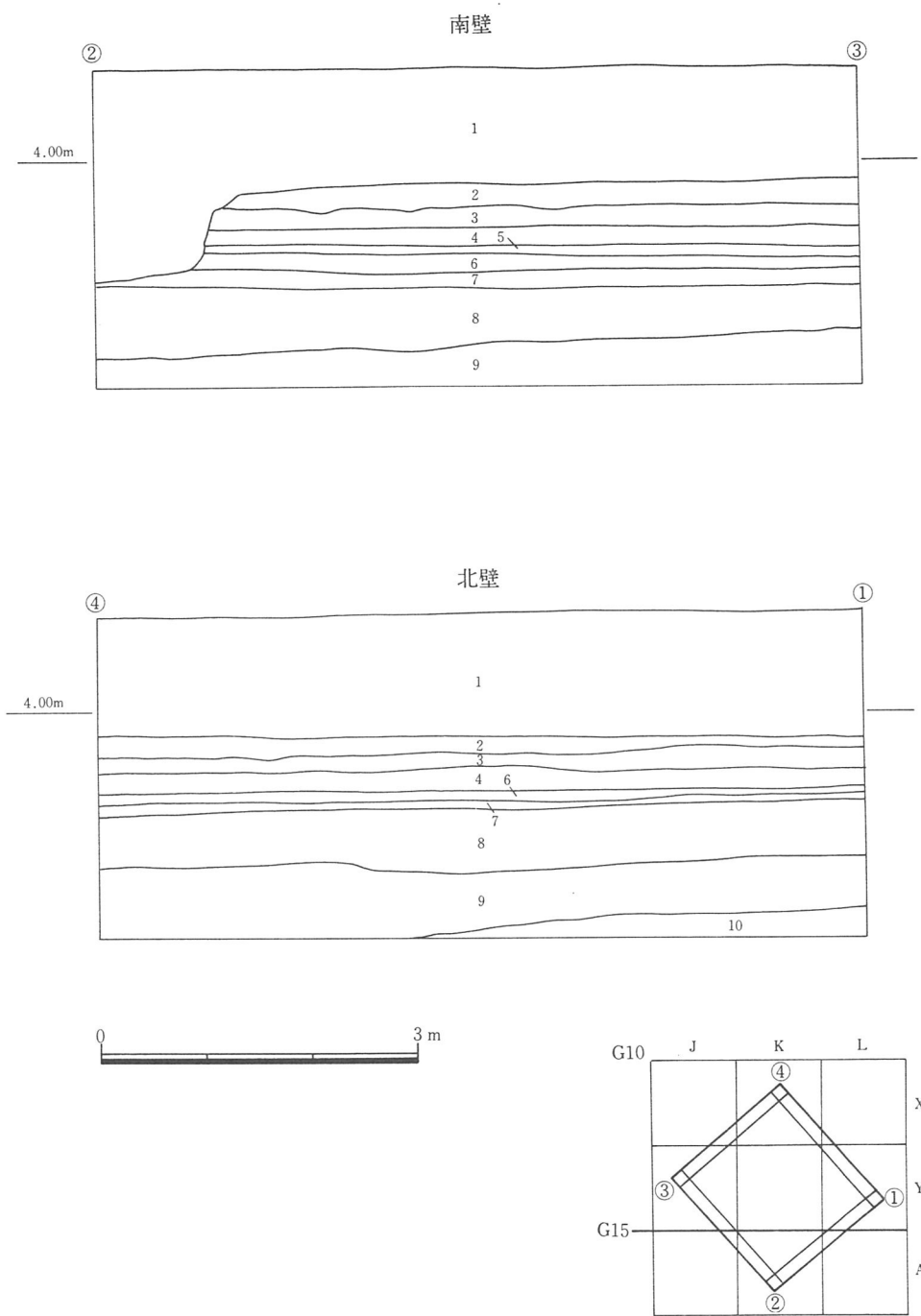
第9图 III区土层断面图(2)
