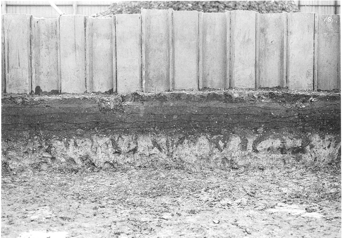
I区東壁断面（西から）
