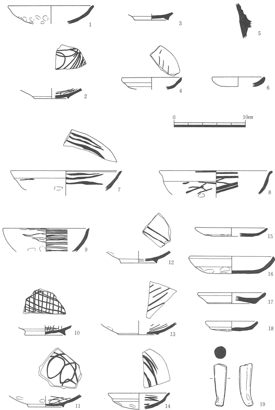
第11图 出土遺物実測図(1)
