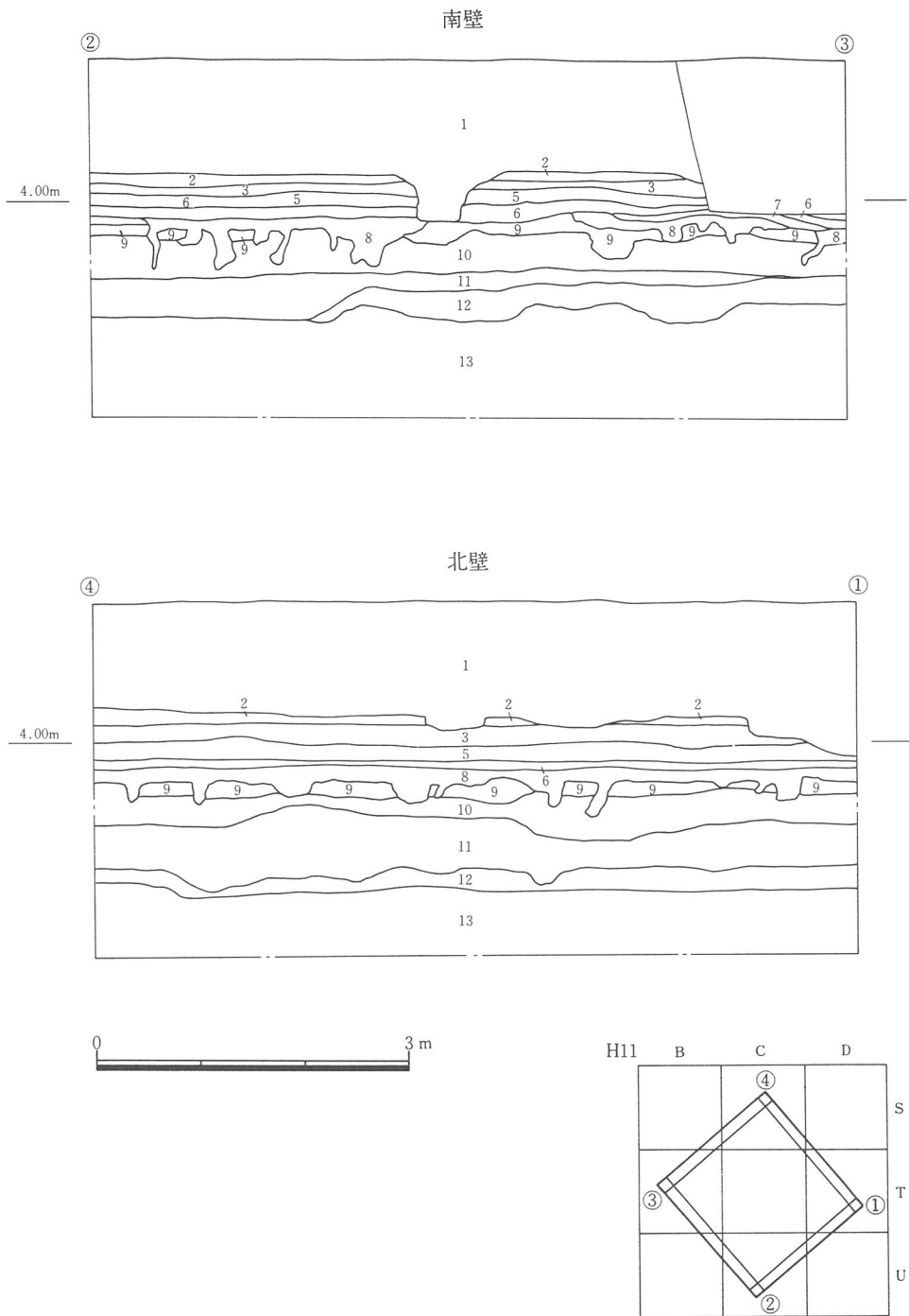
第5图 I区土层断面图(2)
