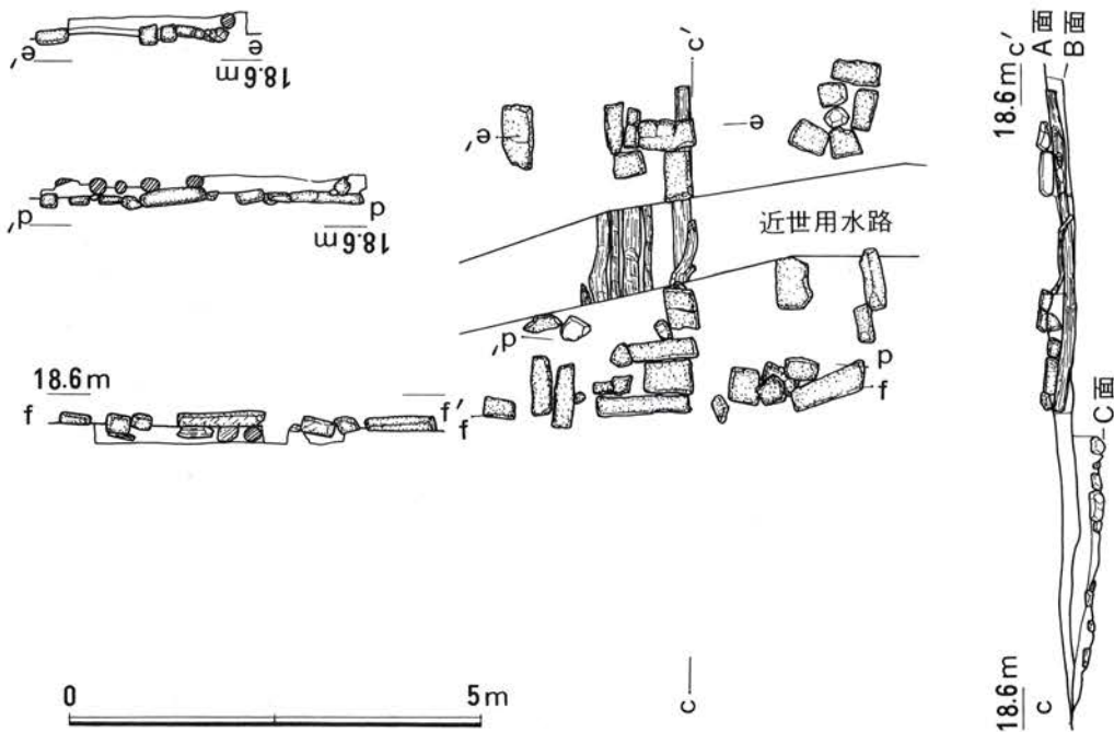
図5 石列下の木材検出状況図
