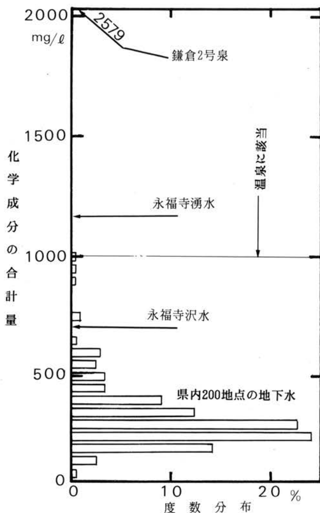
図18 化学成分の合計量の度数分布—— 県内200地点の地下水および永福寺湧水、周辺の地下水等 永福寺湧水、鎌倉2号泉、永福寺沢水は、県内の地下水と比較して化学成分の合計量が多いことが判る。
