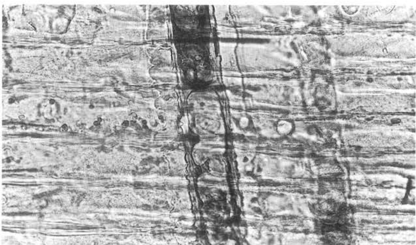
c. クロマツ (放射断面) bar:0.1mm
