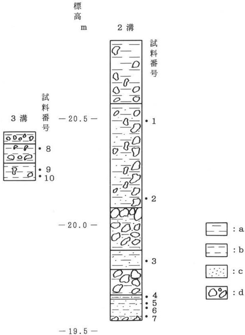
図12 永福寺の溝内堆積物の地質柱状図
