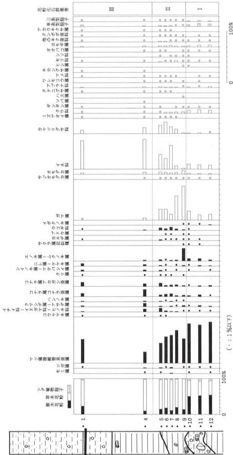
図16 永福寺苑池堆積物の主要花粉化石分布図
