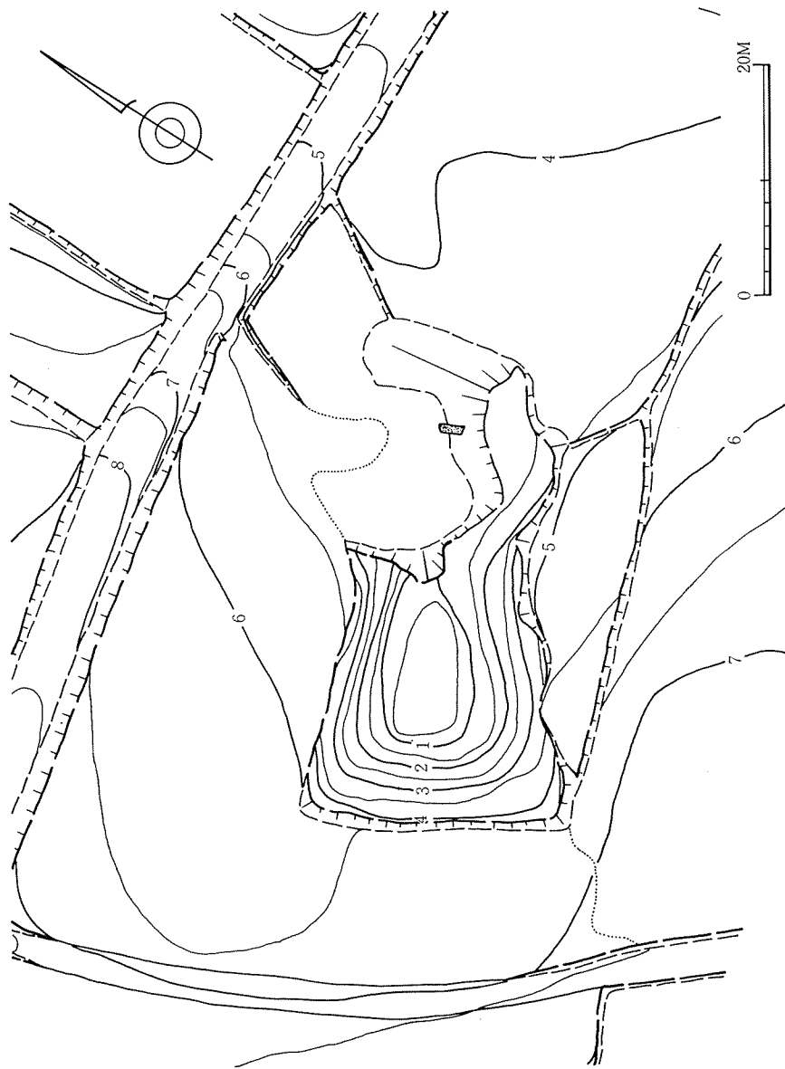
第15図 男塚古墳地形測量図 (1 / 600)
