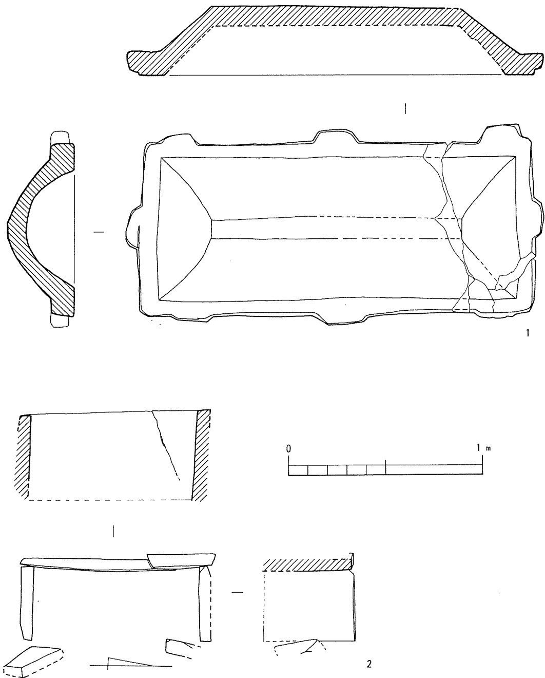
第6図 西潤野古墳石蓋土壇(1), 西潤野箱式石棺(2)実測図
