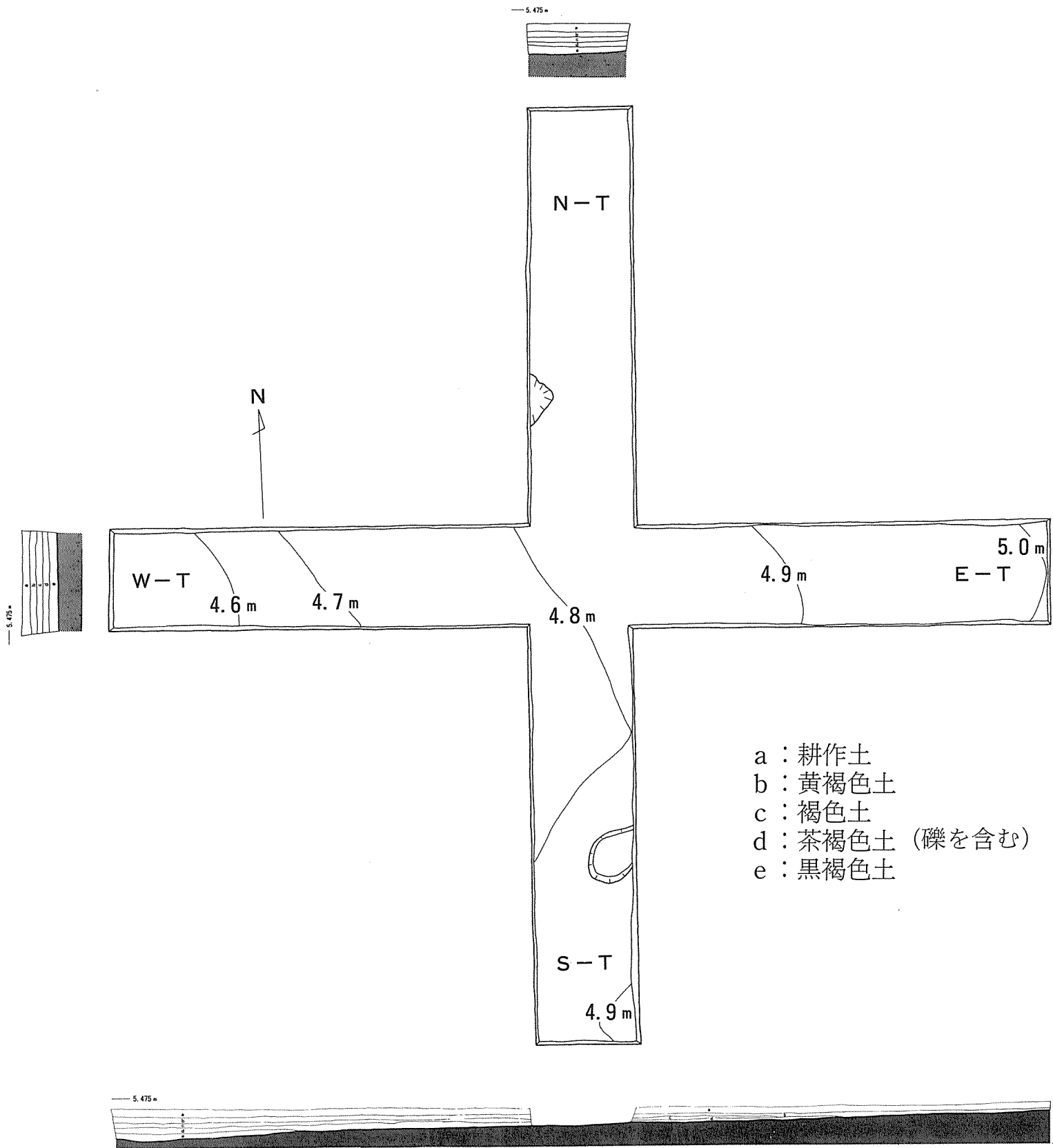
Fig 3 トレンチ実測図及び土層断面図 1 / 100
