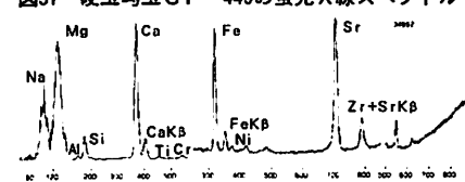
図38 硬玉製勾玉 G P-462-11の蛍光X線スペクトル
