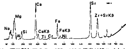
図32 硬玉製勾玉 G P-355-133の蛍光X線スペクトル
