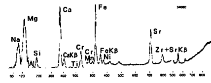
図36 硬玉製勾玉 G P-433-14の蛍光X線スペクトル
