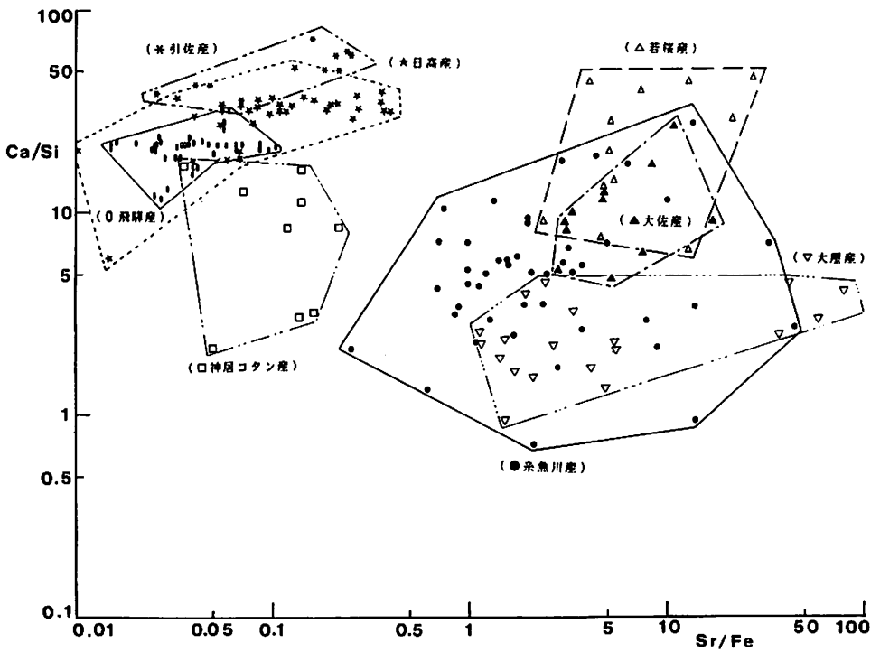
図25 ヒスイ原石の元素比值Ca/Si対Sr/Feの分布および分布範囲
