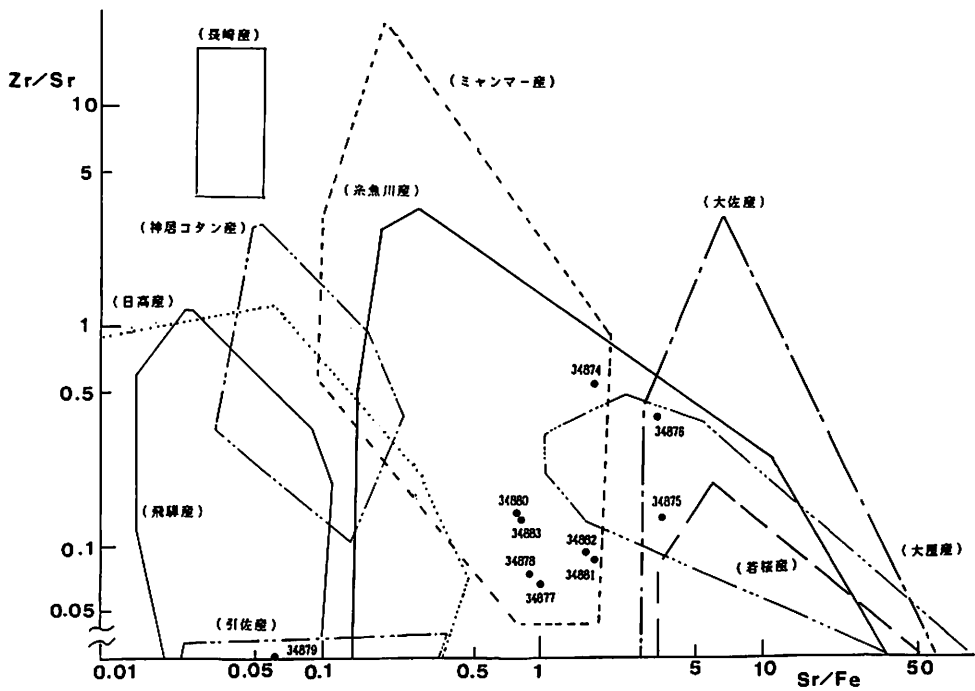
図27 大川遺跡出土の硬玉製勾玉のZr/Sr対Sr/Feの分布
