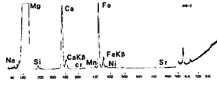
図35 軟玉製勾玉 G P-432-2の蛍光X線スペクトル
