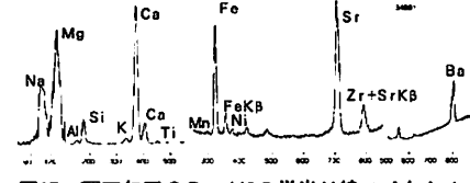
図37 硬玉製勾玉 G P-449の蛍光X線スペクトル
