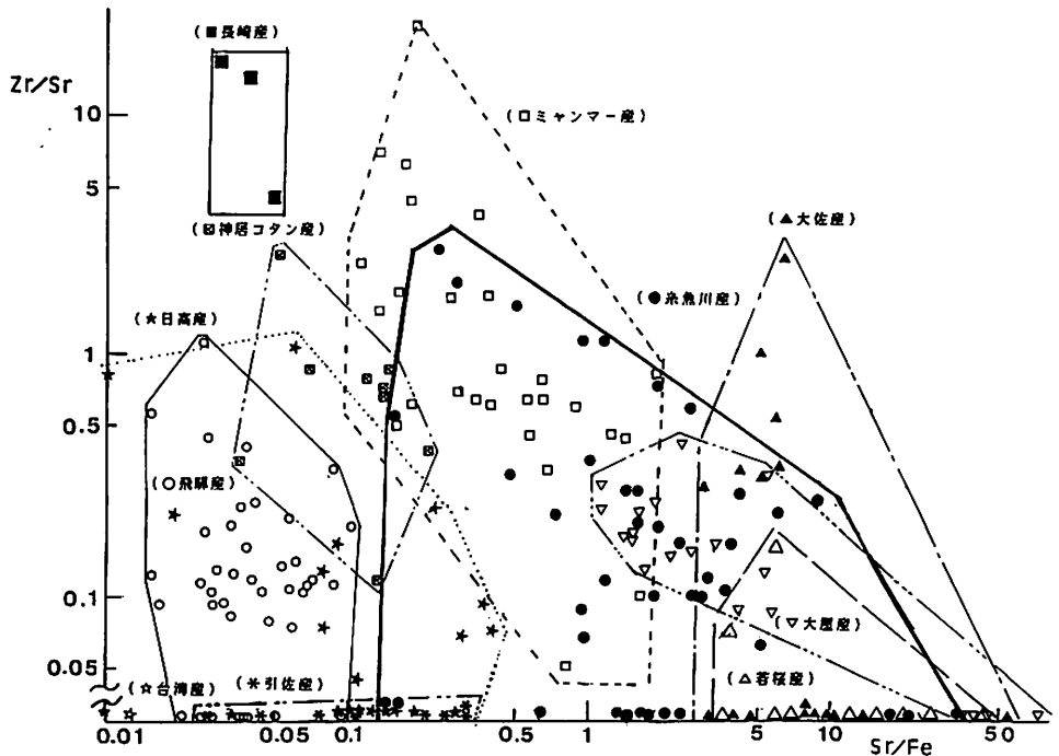
図24 ヒスイ原石の元素比值Zr/Sr対Sr/Feの分布および分布範囲
