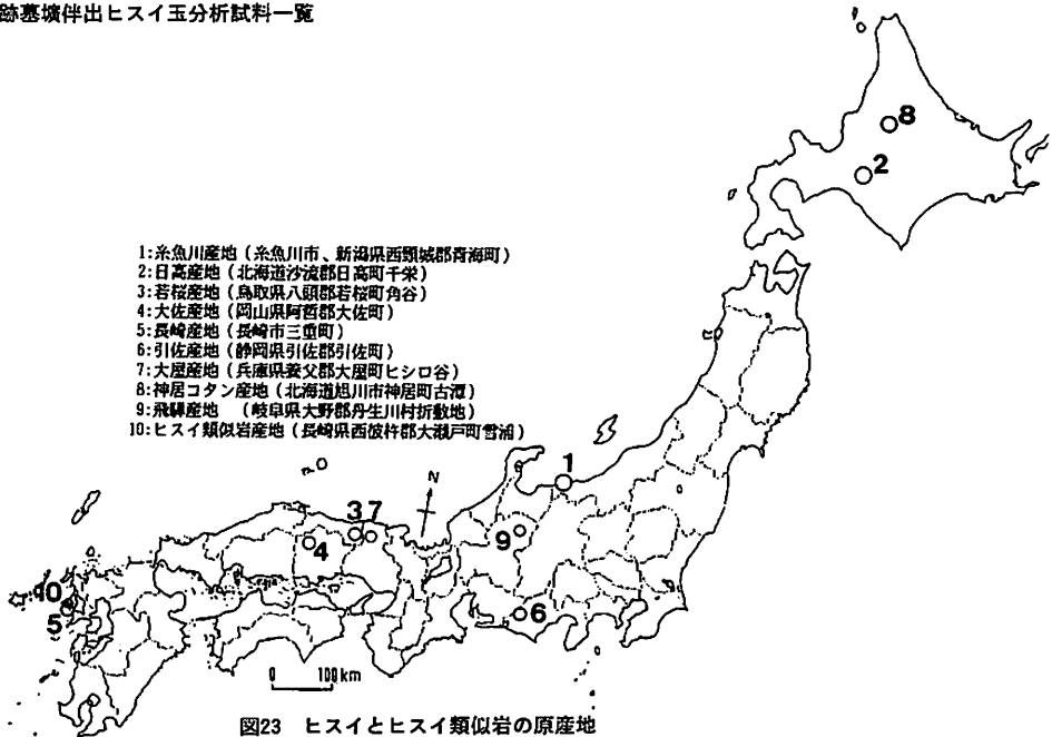
図23 ヒスイとヒスイ類似岩の原産地
