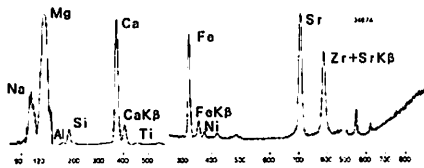
図30 硬玉製勾玉 G P-105の蛍光X線スペクトル
