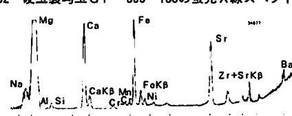
図33 硬玉製勾玉 G P-355-141の蛍光X線スペクトル
