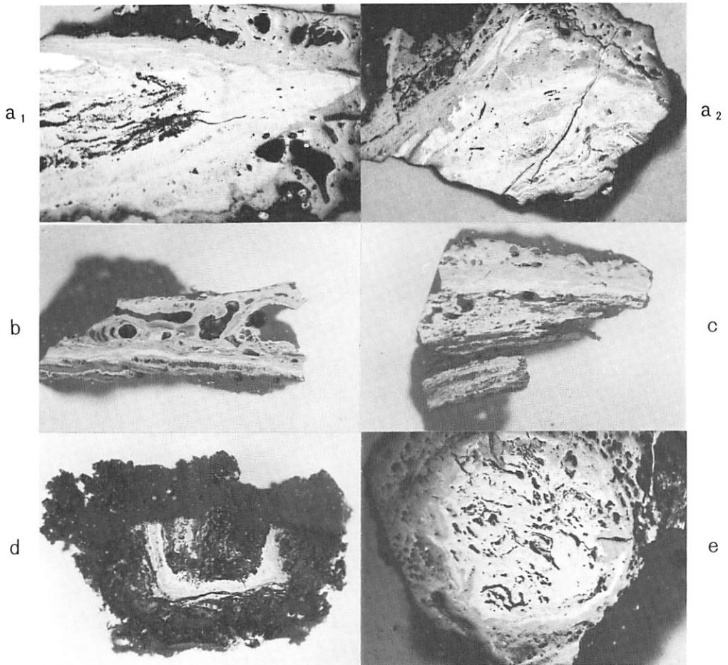
写真33 錆試料片のマクロ組織
