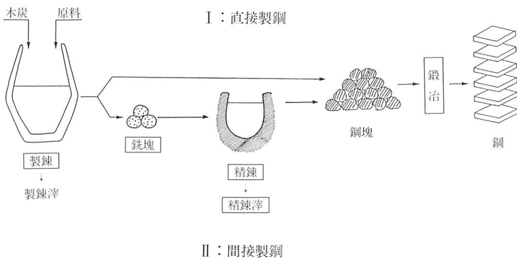
図10 推定される古代の製鉄フロー
