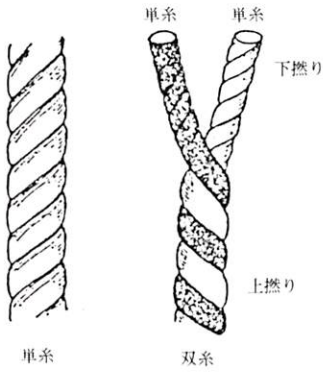
図8 単糸と双糸
