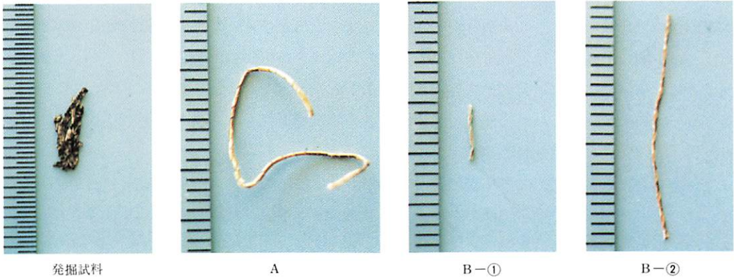
図8 単糸と双糸
