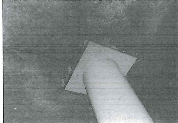
写真4 最終設備以前の横穴式石室内補強状況その2 [1977(昭和52)年]
