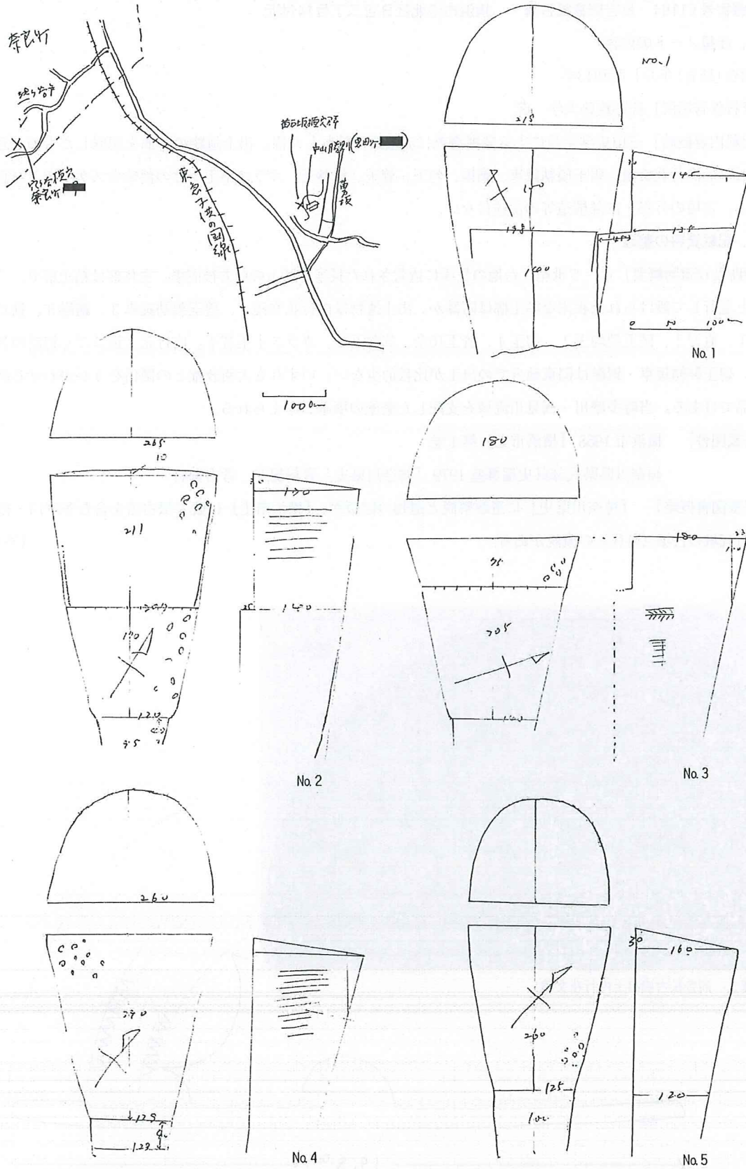
第5図 苗万坂横穴墓群の位置と各横穴墓断面概略図
