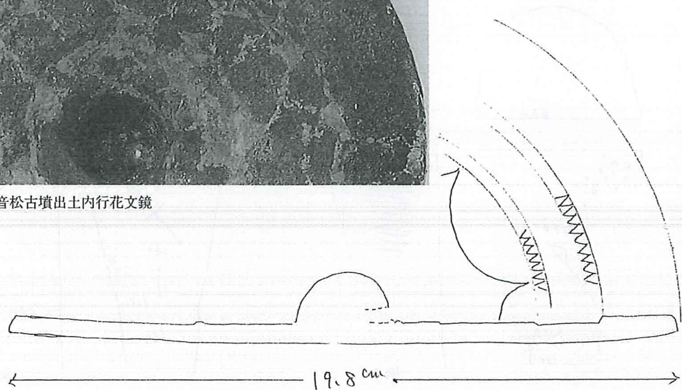
第6図 観音松古墳出土内行花文鏡平・断面図
