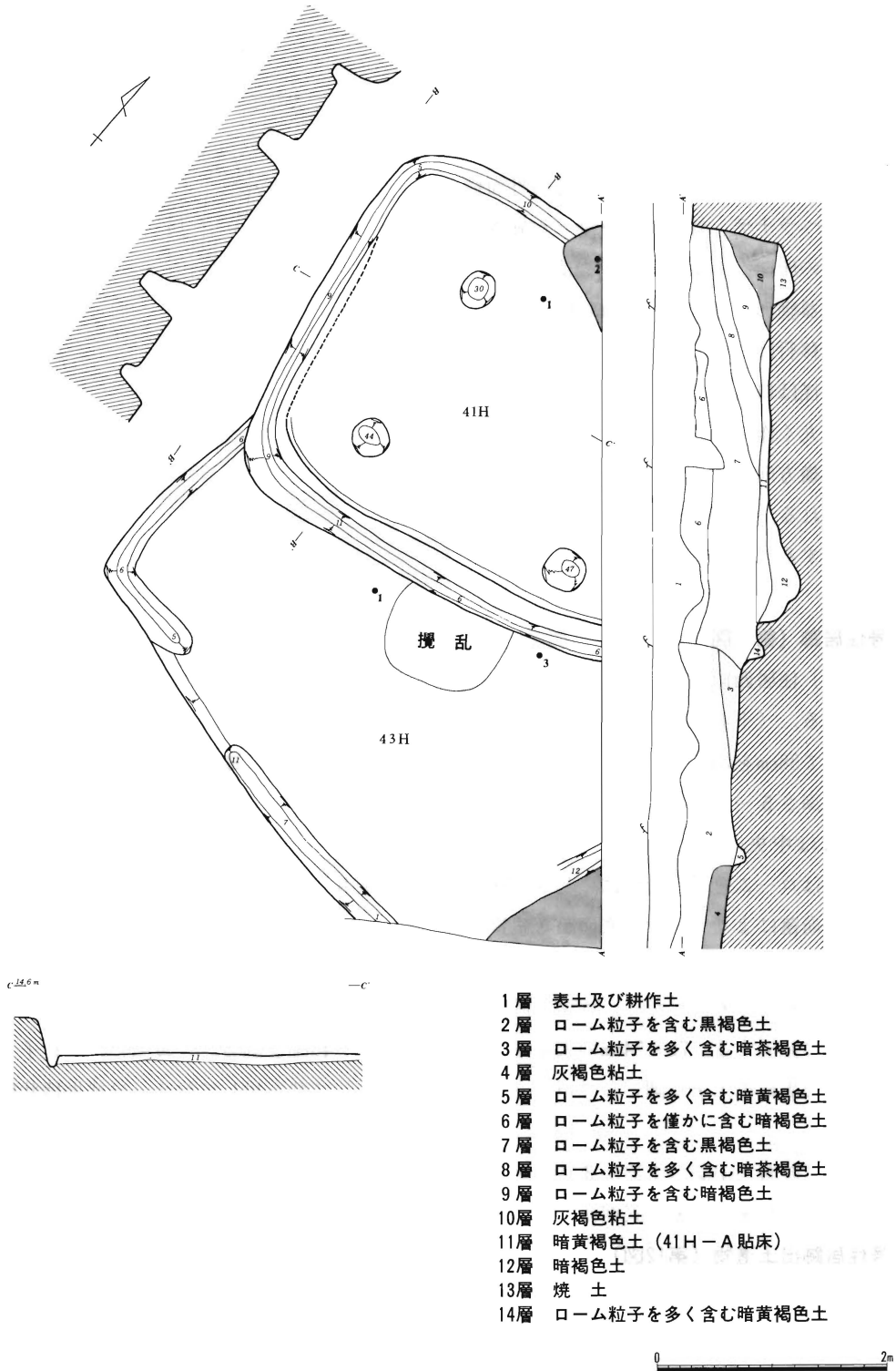
第9図 41・43号住居跡 (1/60)
