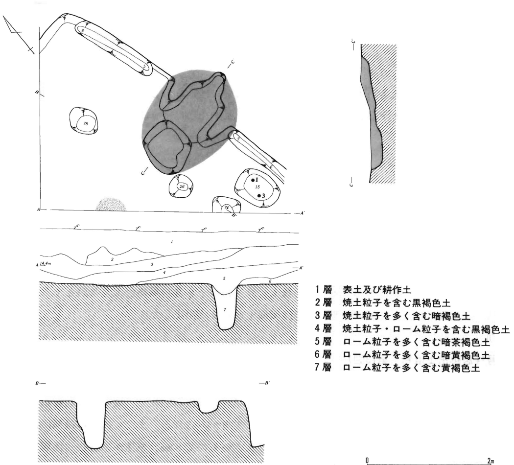
第11図 42号住居跡 (1/60)
