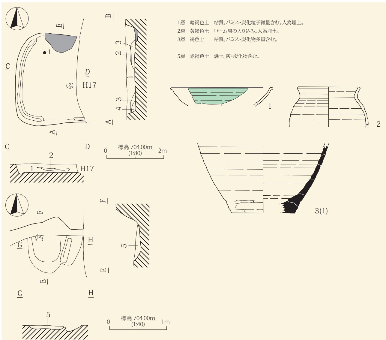
H16号住居址
