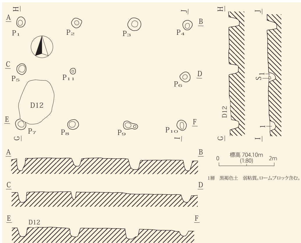
F1号掘立柱建物
