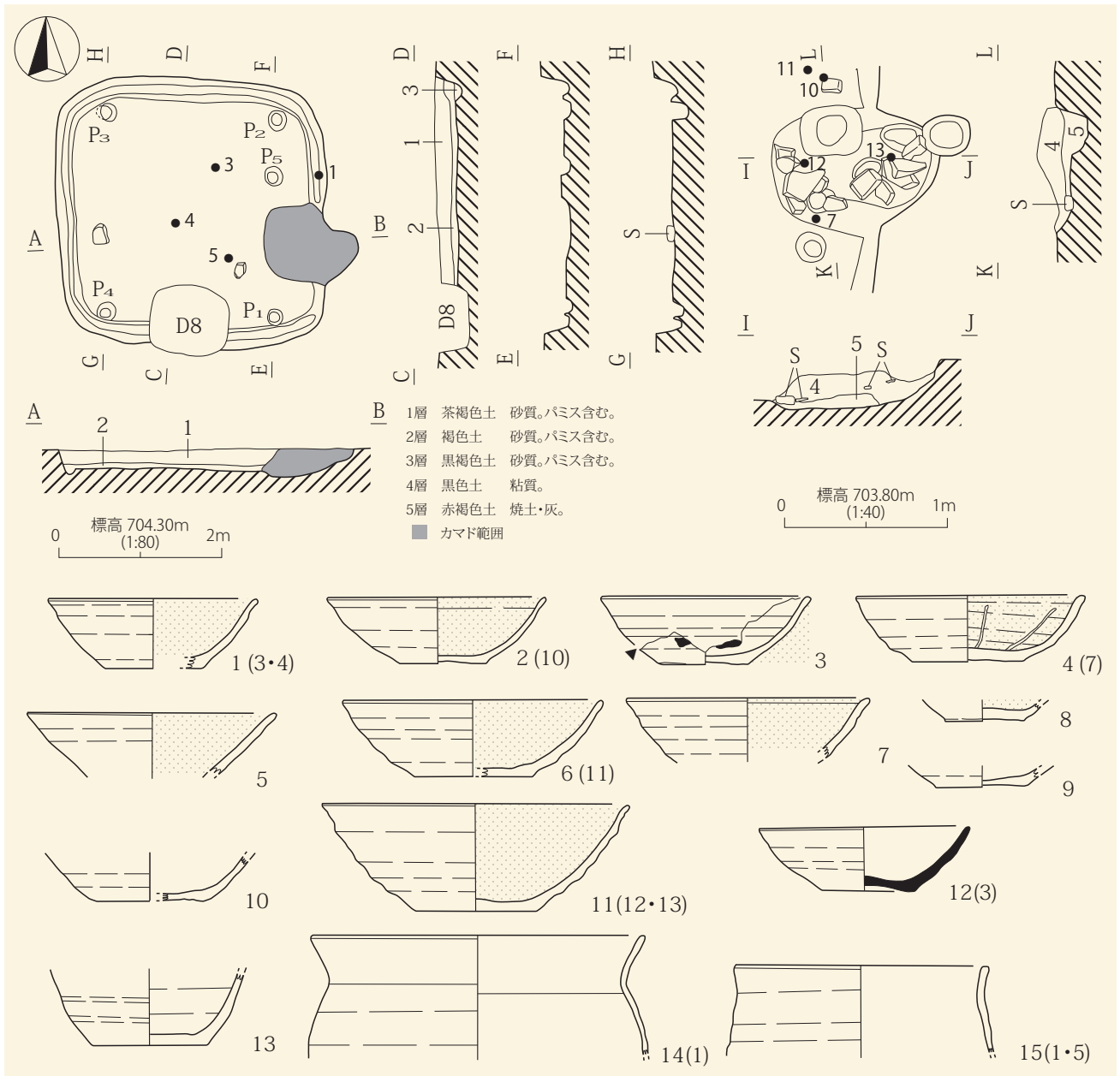
H20号住居址
