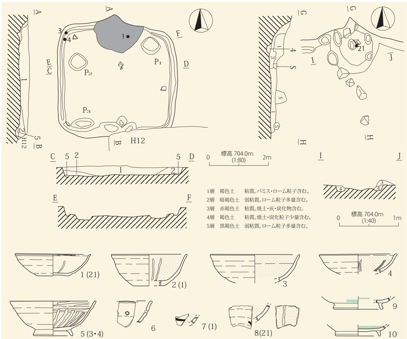
H11号住居址
