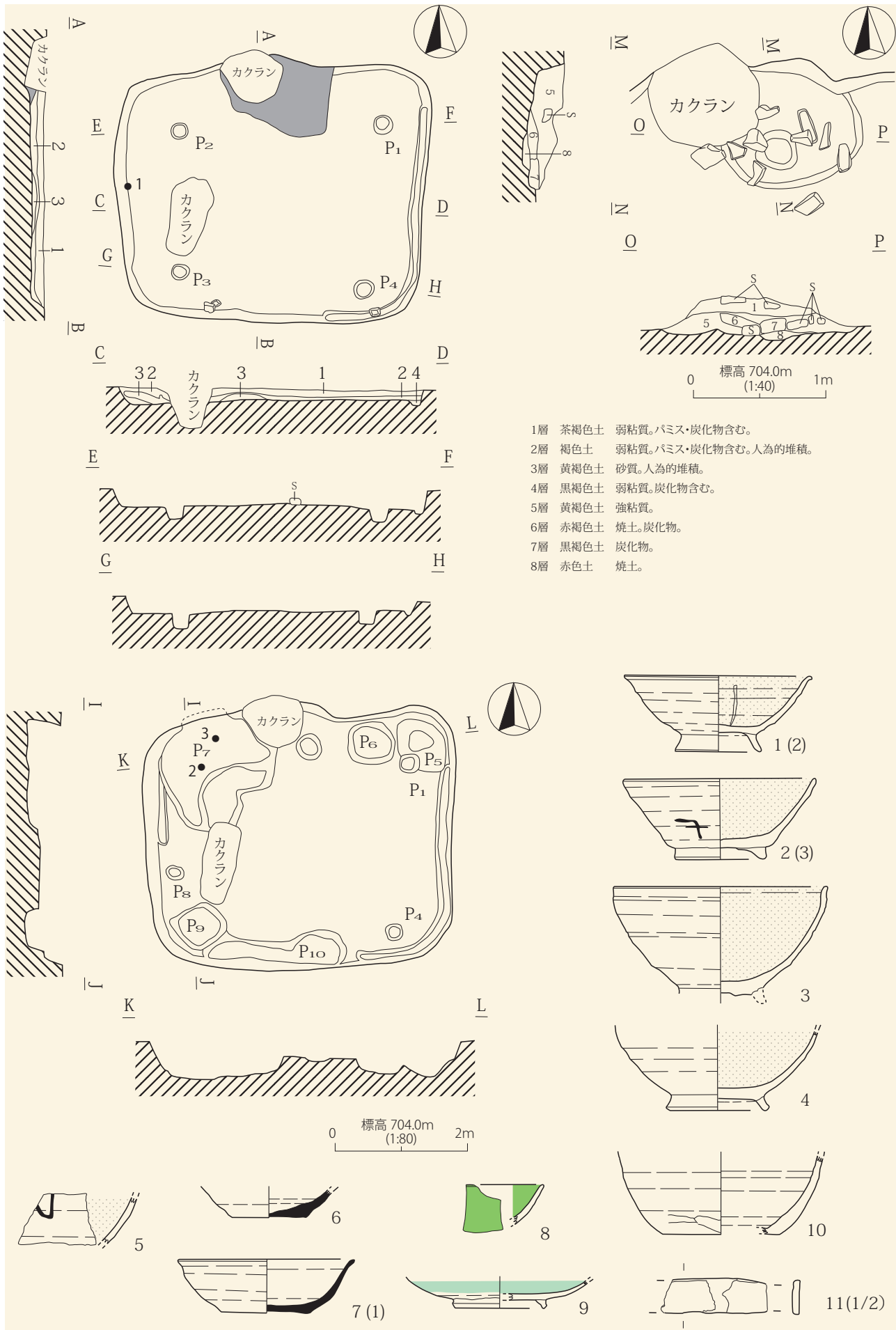
H10号住居址
