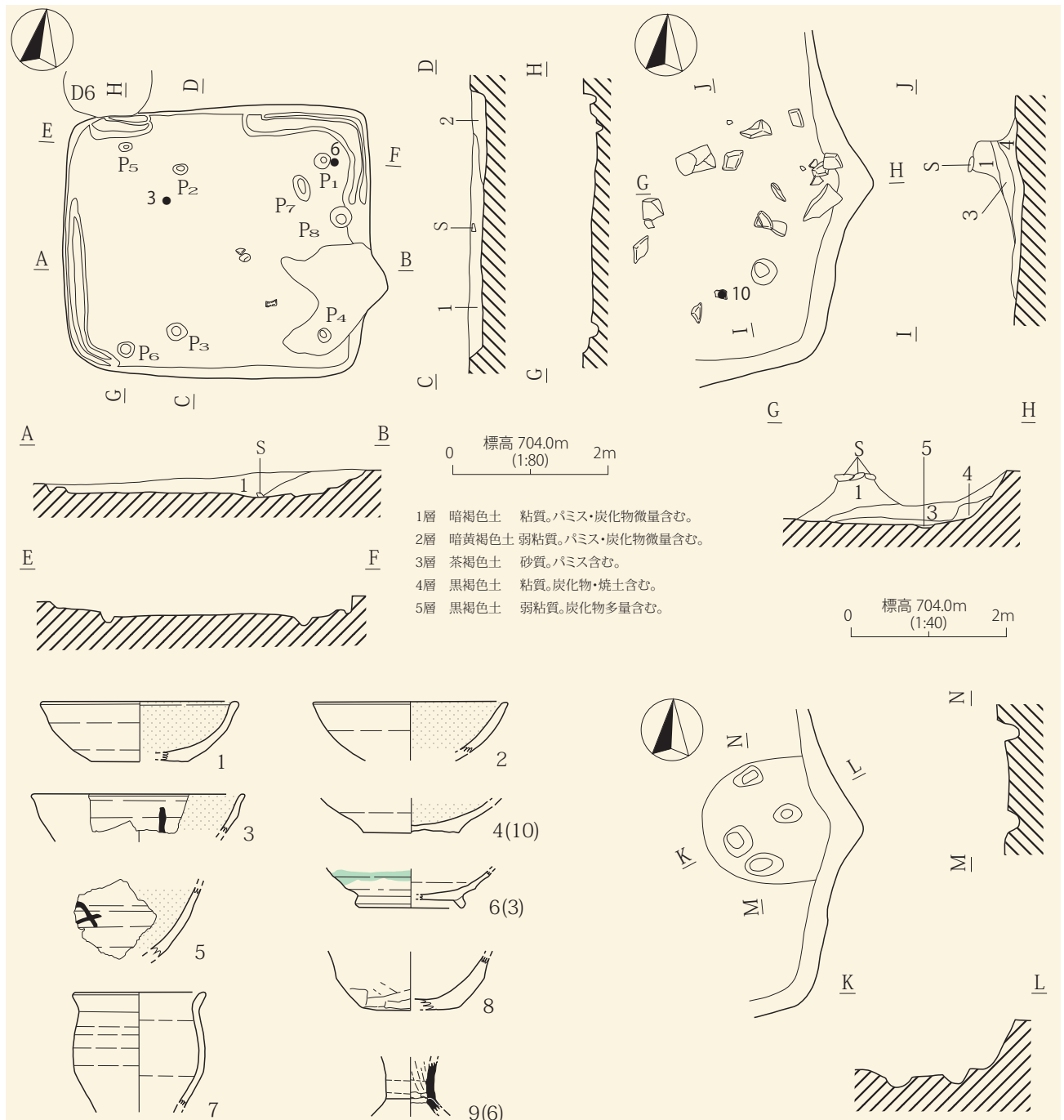
H8号住居址
