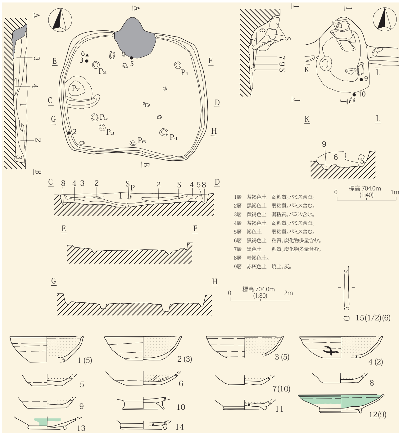
H9号住居址
