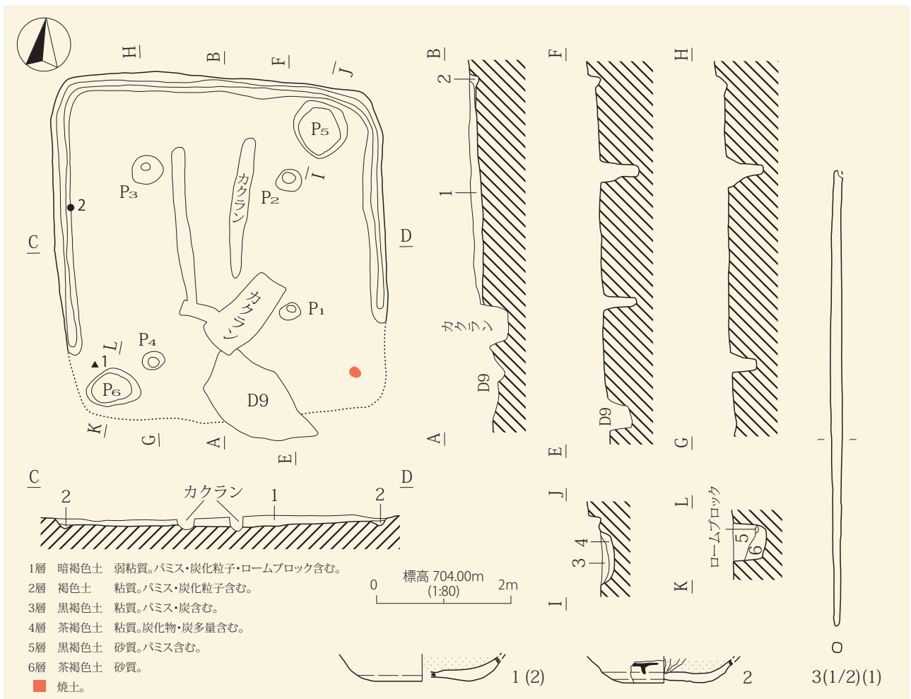
H18号住居址
