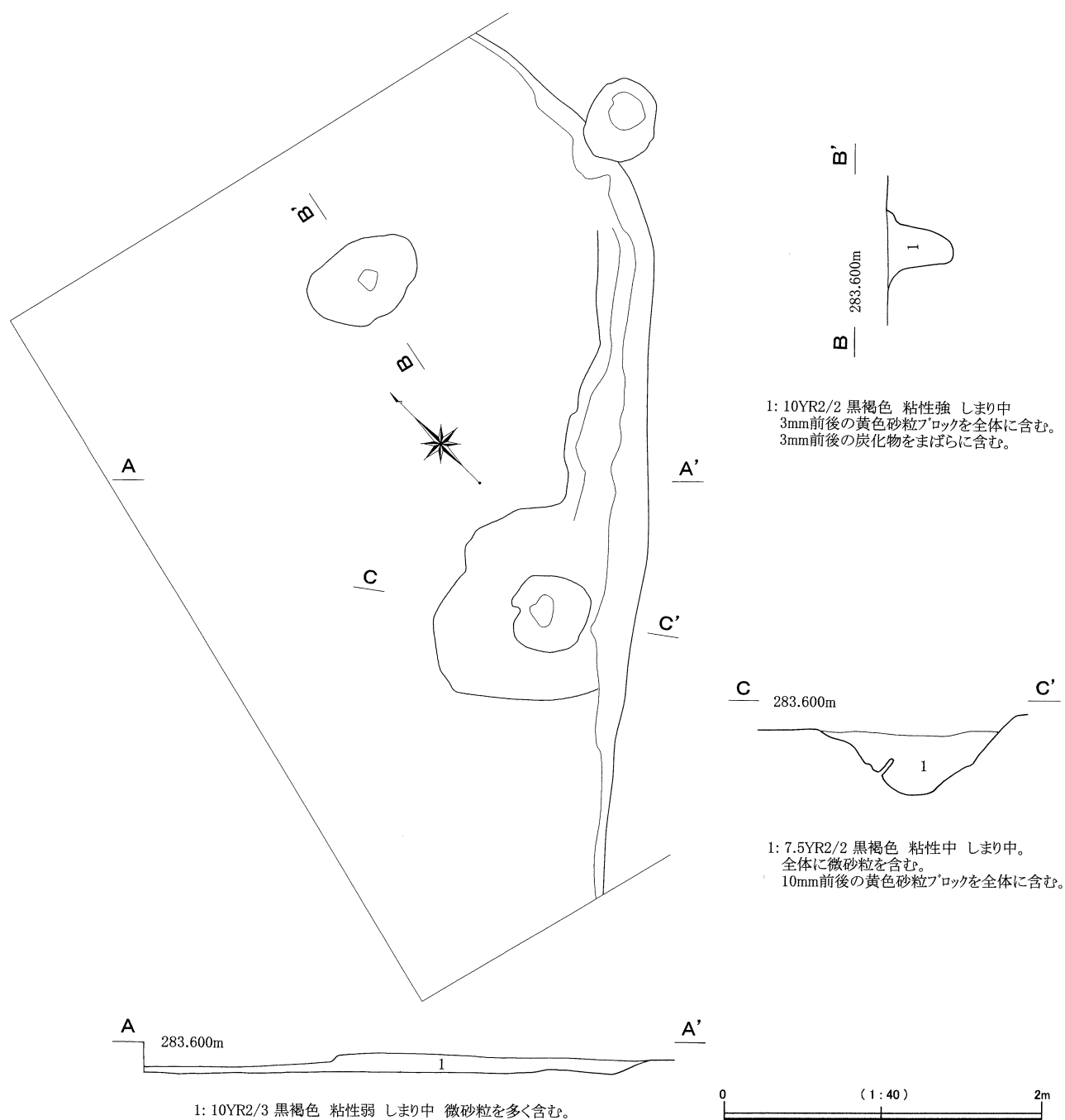
第4図 第5次1号住居跡
