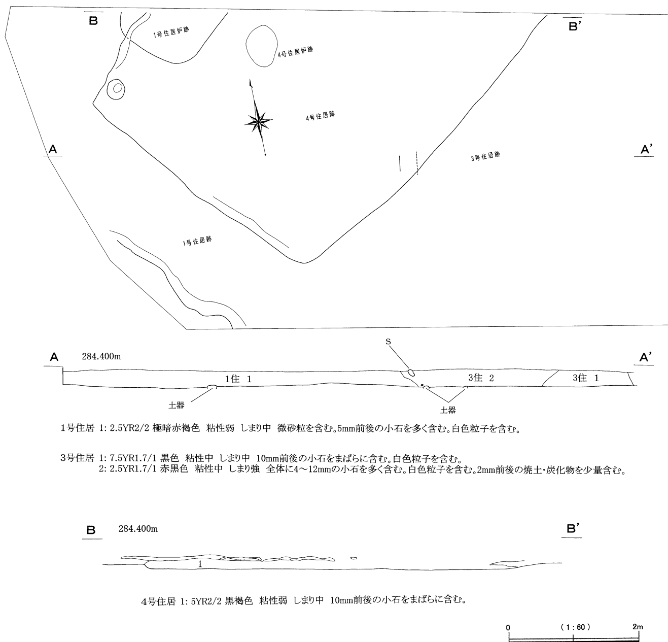
第14図 第6次1・3・4号住居跡
