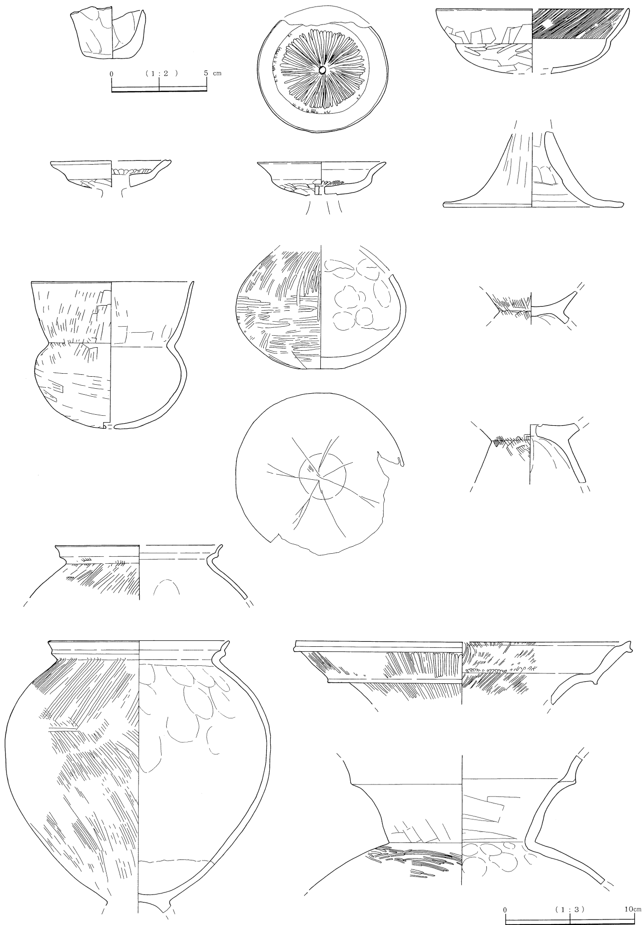
第24図 第2次1号住居跡出土遺物
