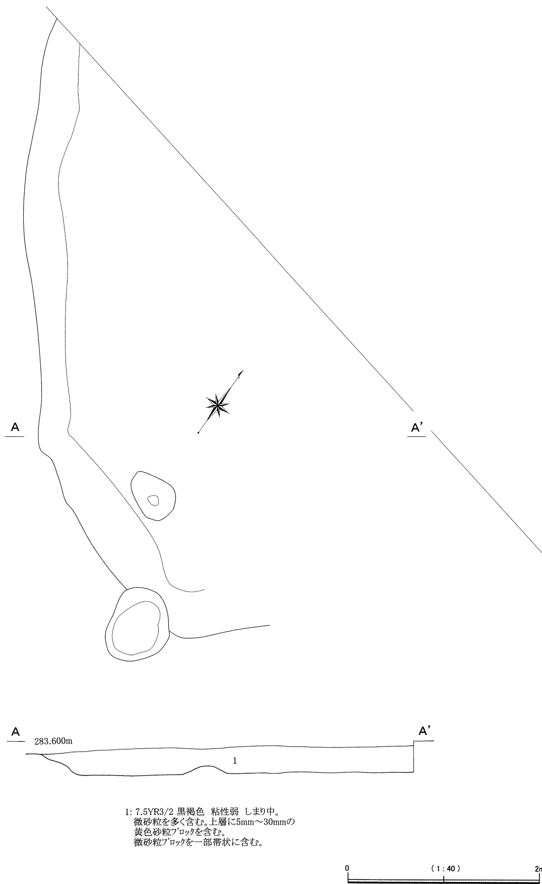
第6図 第5次2号住居跡
