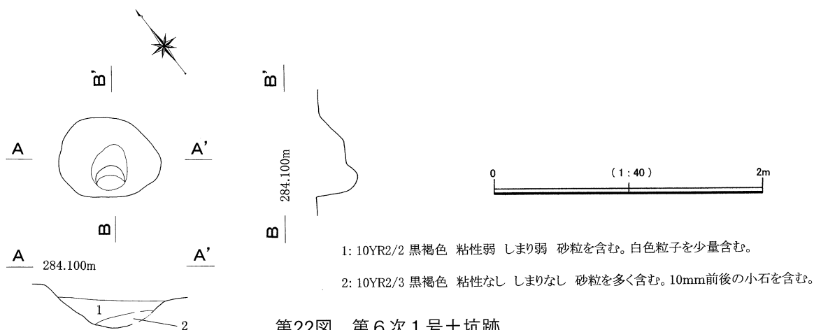
第22図 第6次1号土坑跡
