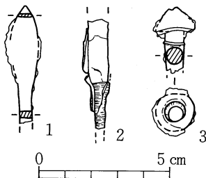
第55図 51号横穴墓出土鉄器 実測図 (1/2)
