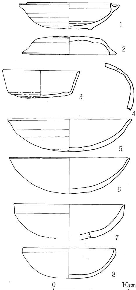
第8図 8号横穴墓出土土器実測図 (1/3)
