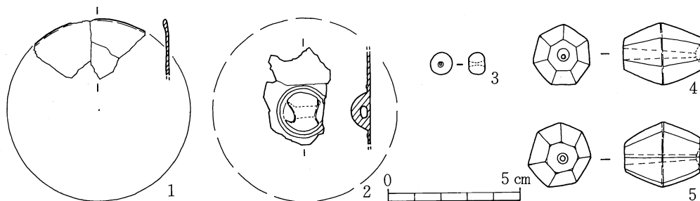
第58図 52号横穴墓出土鏡・玉類実測図 (1/2)
