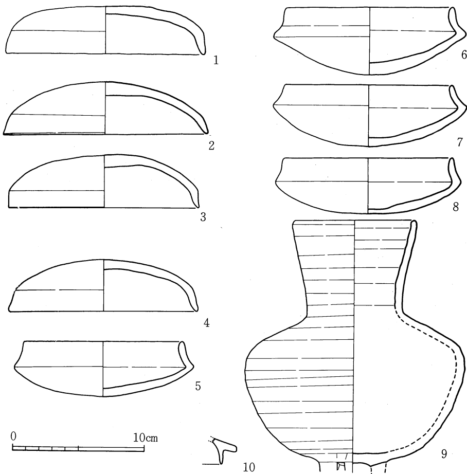
第38図 40号横穴墓出土土器実測図(1/3)
