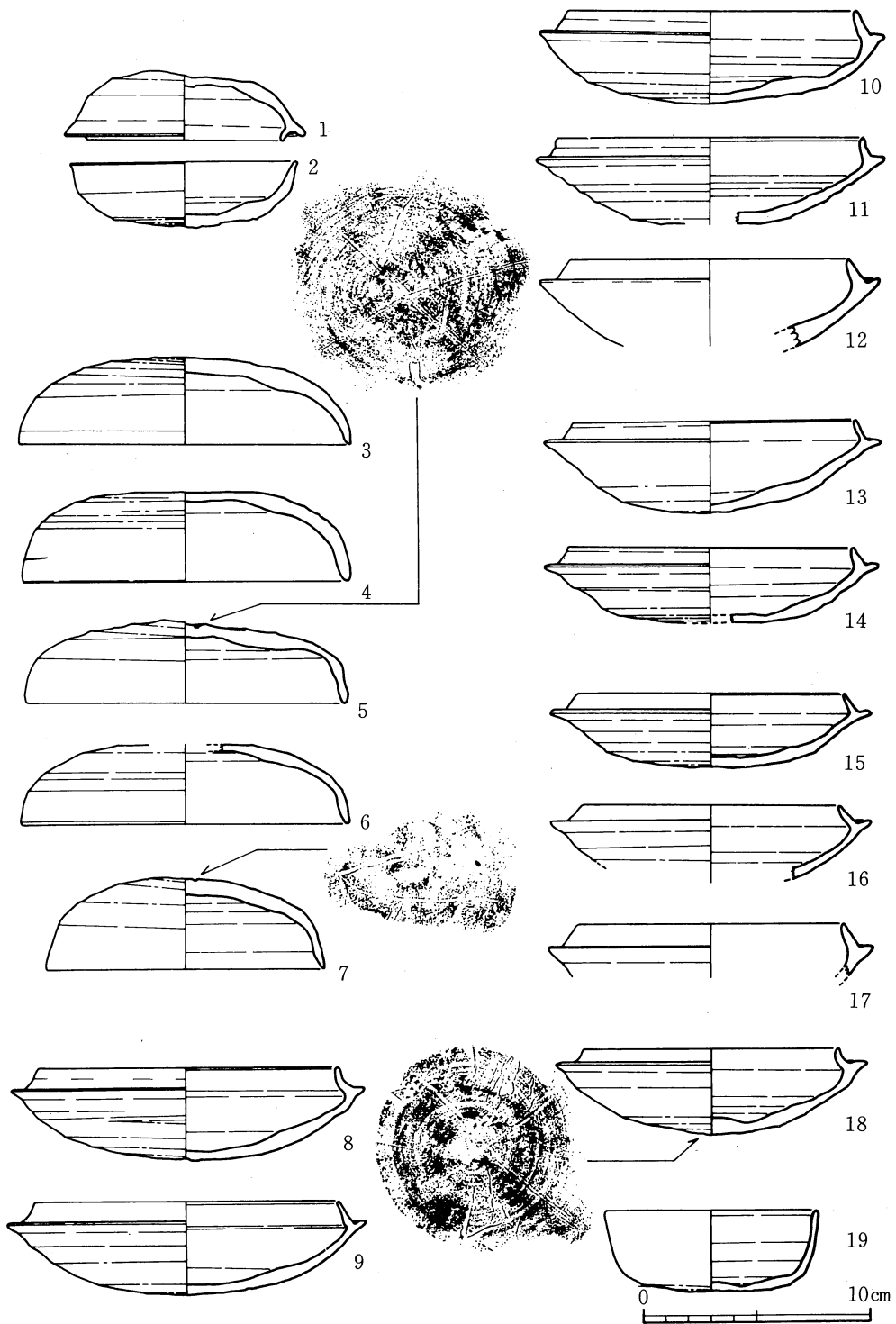
第16图 12号横穴墓出土土器实测图·拓影(3) (1/3)
