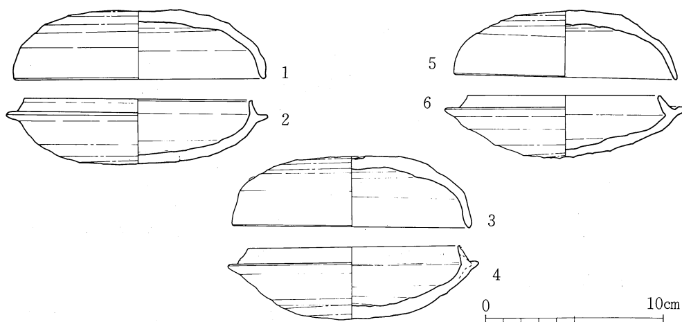
第14図 12号横穴墓出土土器実測図(1) (1/3)
