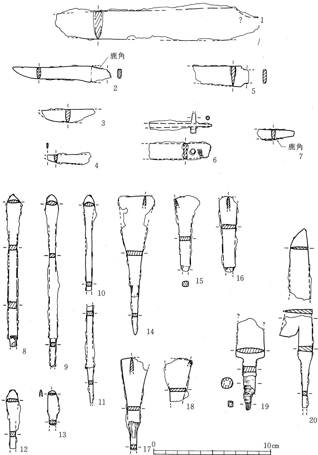
第51图 50号横穴墓出土铁器实测图(1) (1/2)
