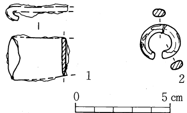
第9図 8号横穴墓出土鉄器 ・装身具実測図 (1/2)
