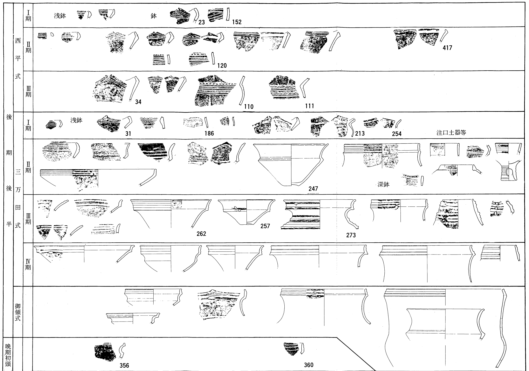
第4図 縄文後期後半土器編年図
