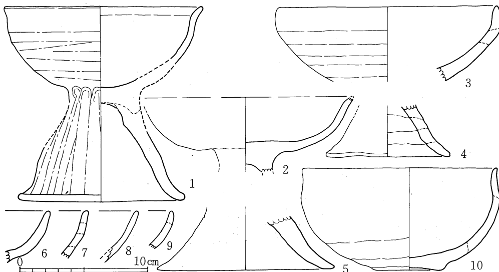
第17図 12号横穴墓出土土器実測図(4) (1/3)
