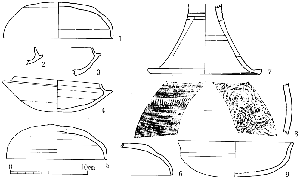
第56図 52号横穴墓出土土器実測図・拓影 (1/3)
