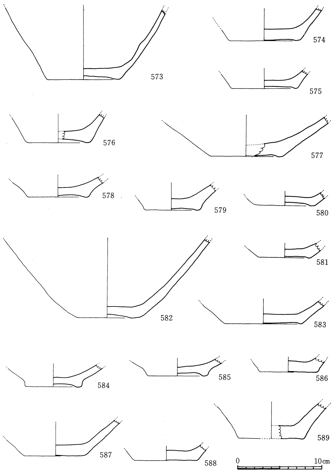
第39图 土器实测图(34)
