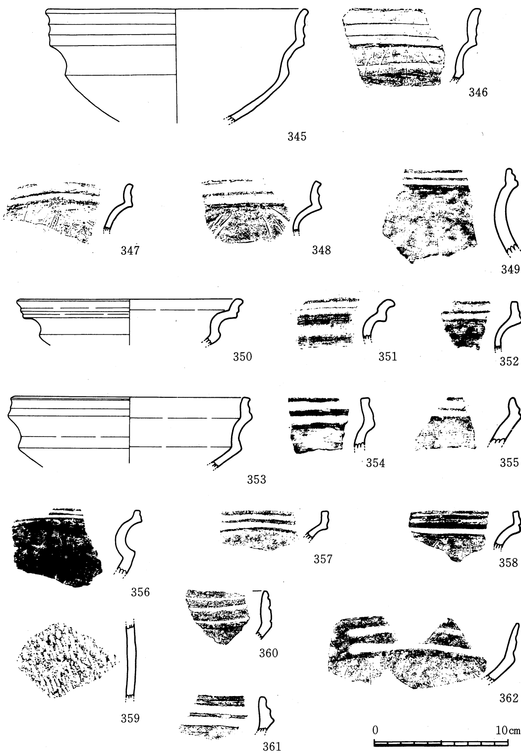
第21图 土器实测图(16)
