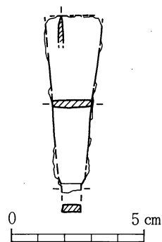
第30図 34号横穴墓 出土鉄器実測図 (1/2)
