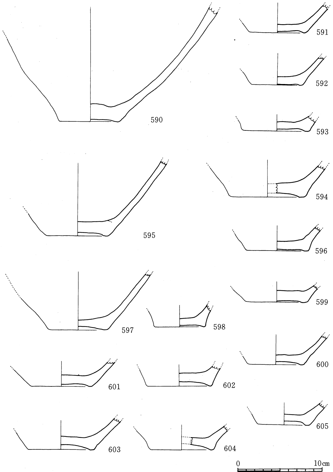
第40图 土器实测图(35)
