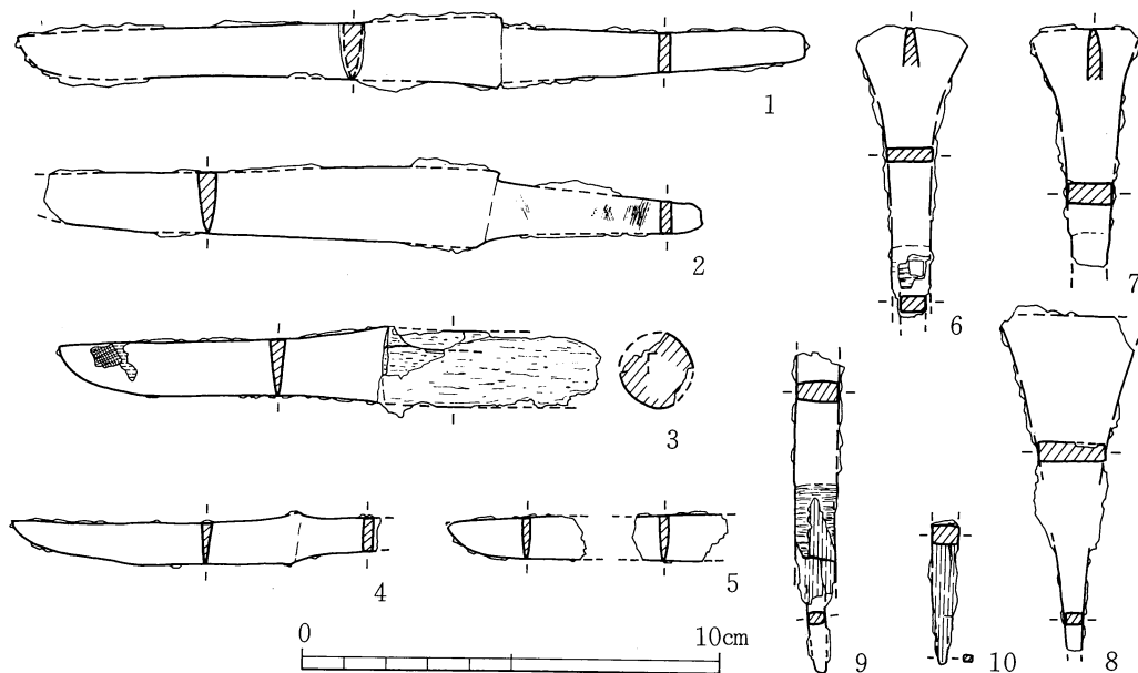
第6図 6号横穴墓出土鉄器実測図(1/2)
