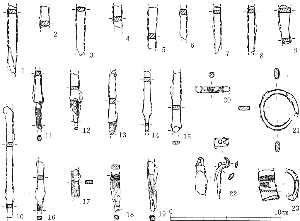
第52図 50号横穴墓出土鉄器実測図(2) (1/2)
