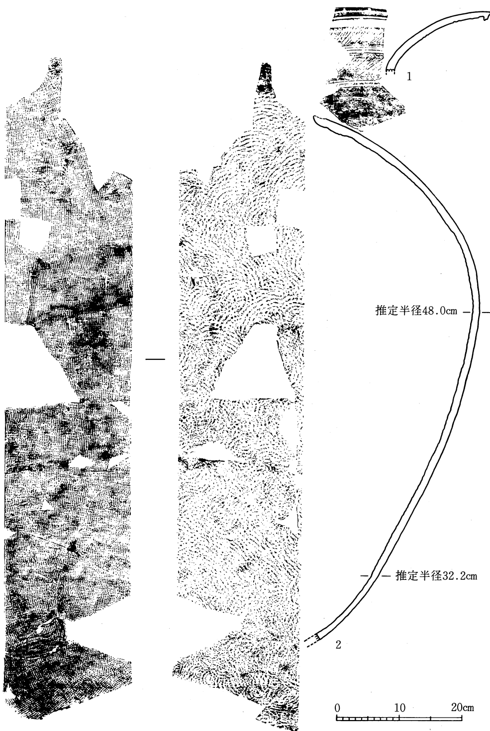
第45图 46号横穴墓出土土器实测图(4) (1/6)
