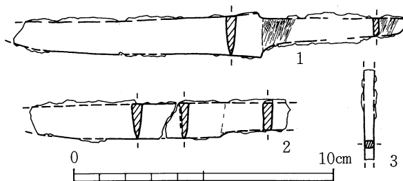
第39図 40号横穴墓出土鉄器実測図 (1/2)
