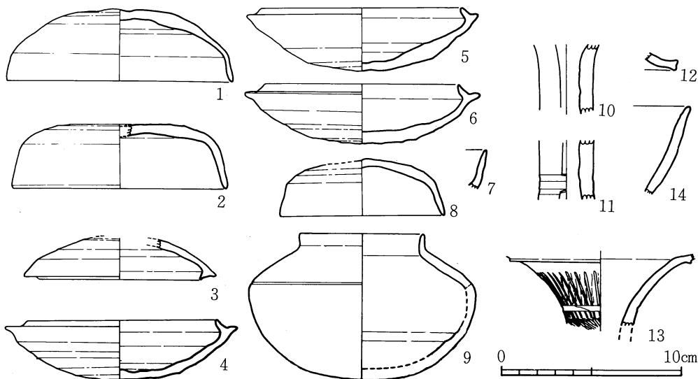
第42図 46号横穴墓出土土器実測図(1) (1/3)
