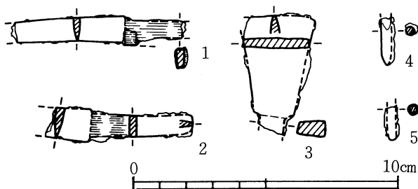
第21図 15号横穴墓出土鉄器実測図(1/2)
