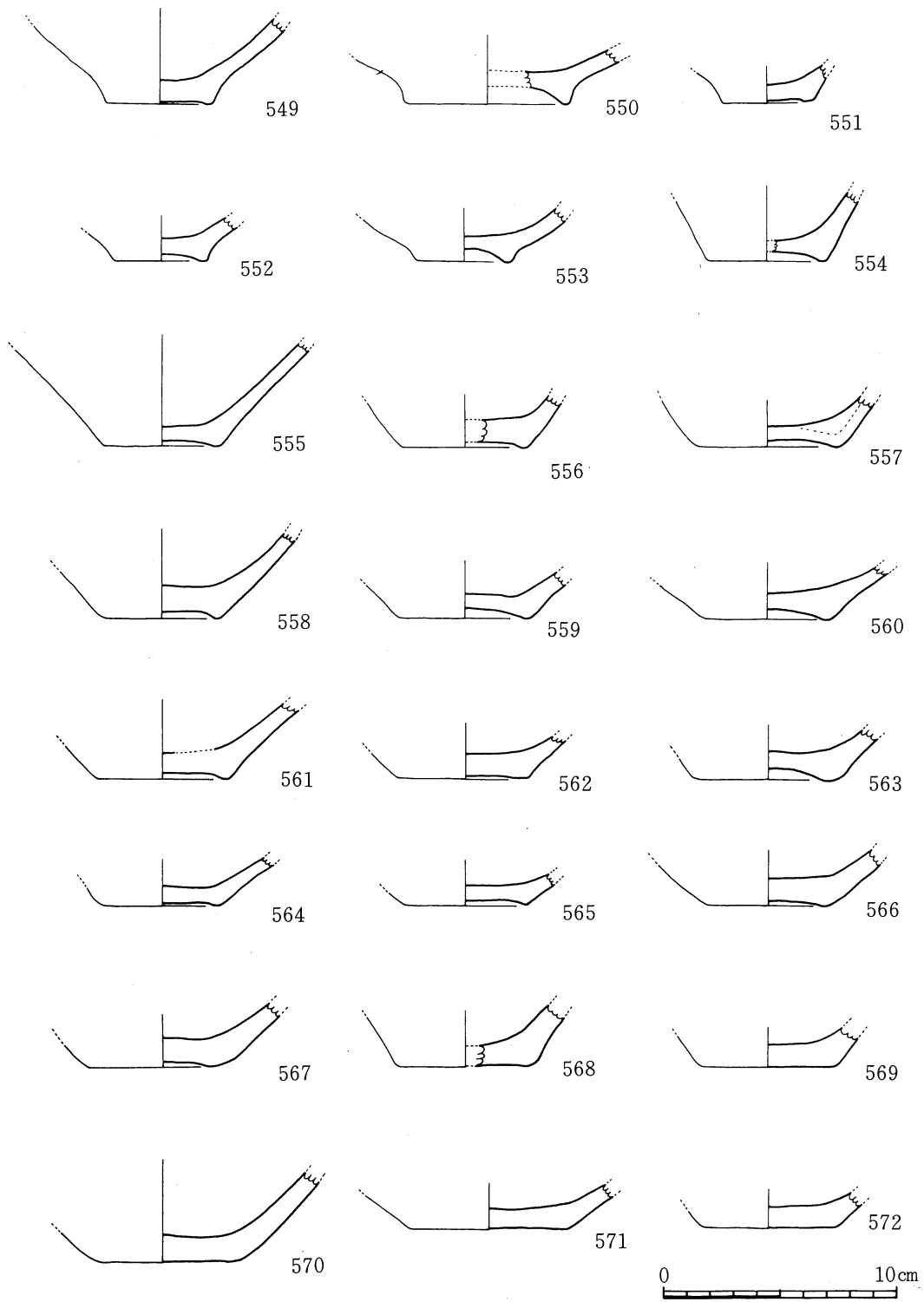
第38图 土器实测图(33)
