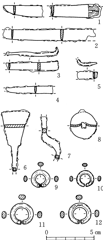
第26図 24号横穴墓出土鉄器 ・装身具実測図 (1/2)
