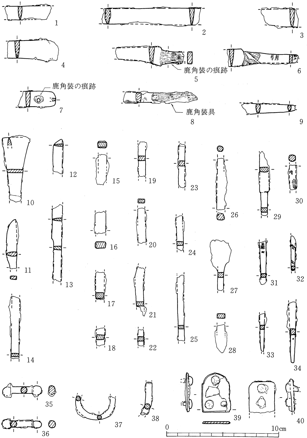
第57図 52号横穴墓出土鉄器実測図 (1/2)
