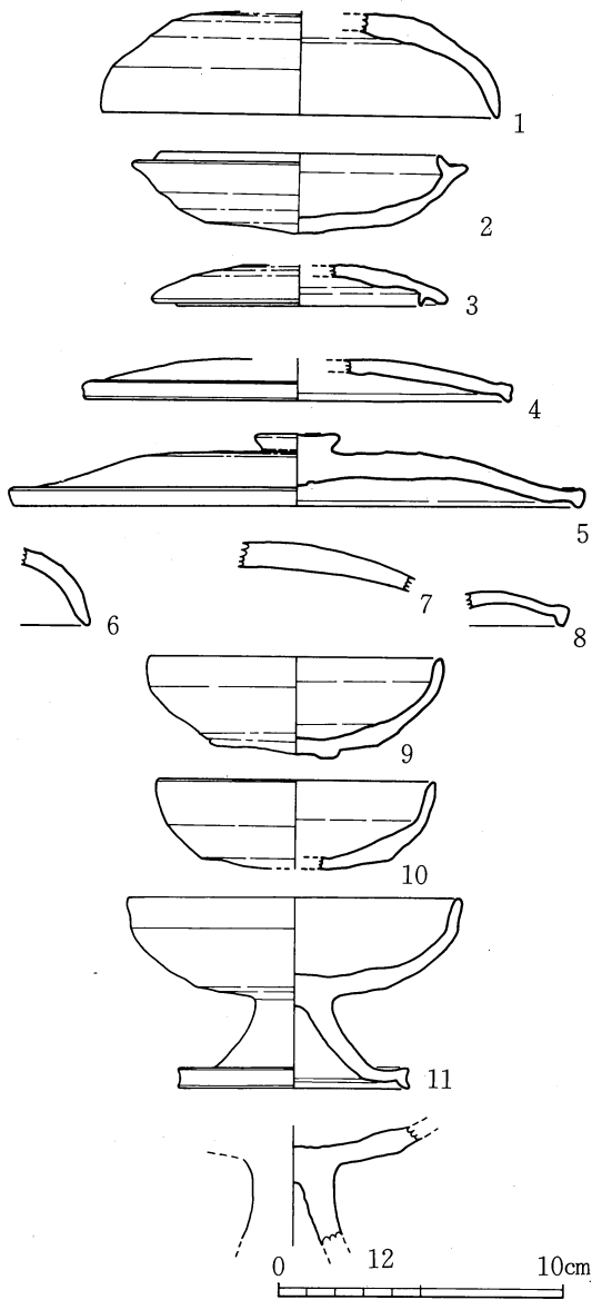
第34図 37号横穴墓出土土器実測図(1) (1/3)
