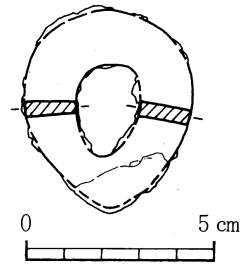
第19図 14号横穴墓出土鉄器実測図 (1/2)
