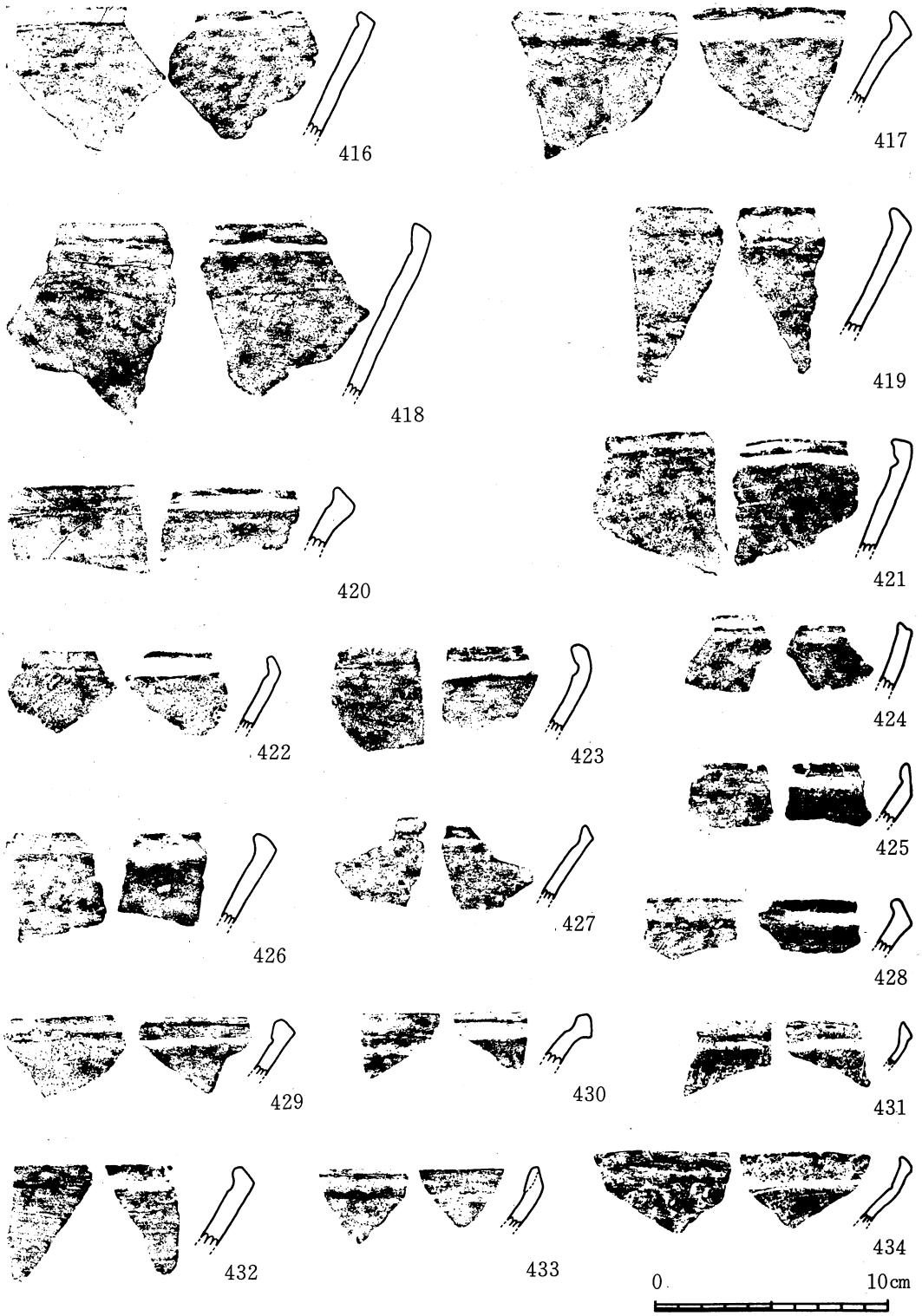
第27图 土器实测图(22)
