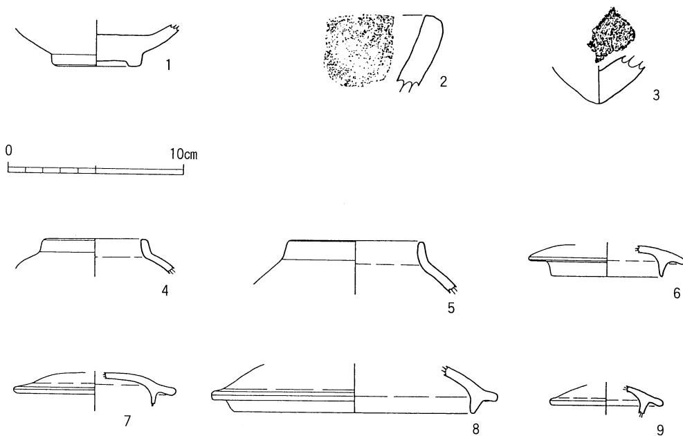
第20図 陶磁器実測図
