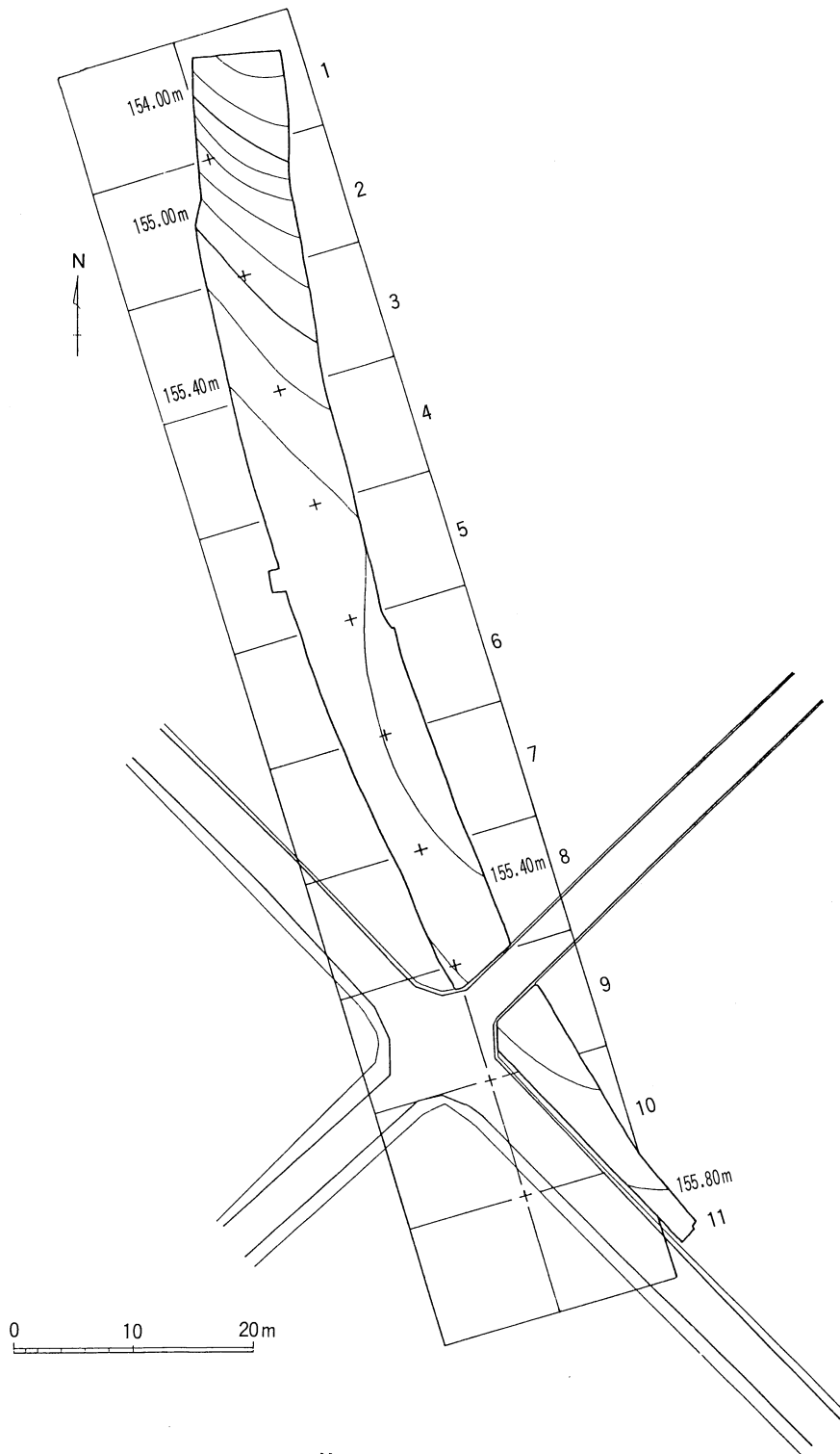
第4図 グリッド配置図
