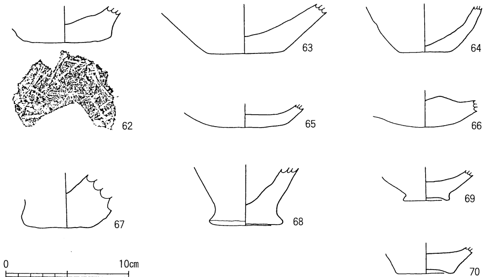
第14図 弥生土器実測図(3)
