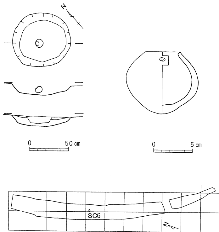
第11図 SC6遺構・遺物実測図
