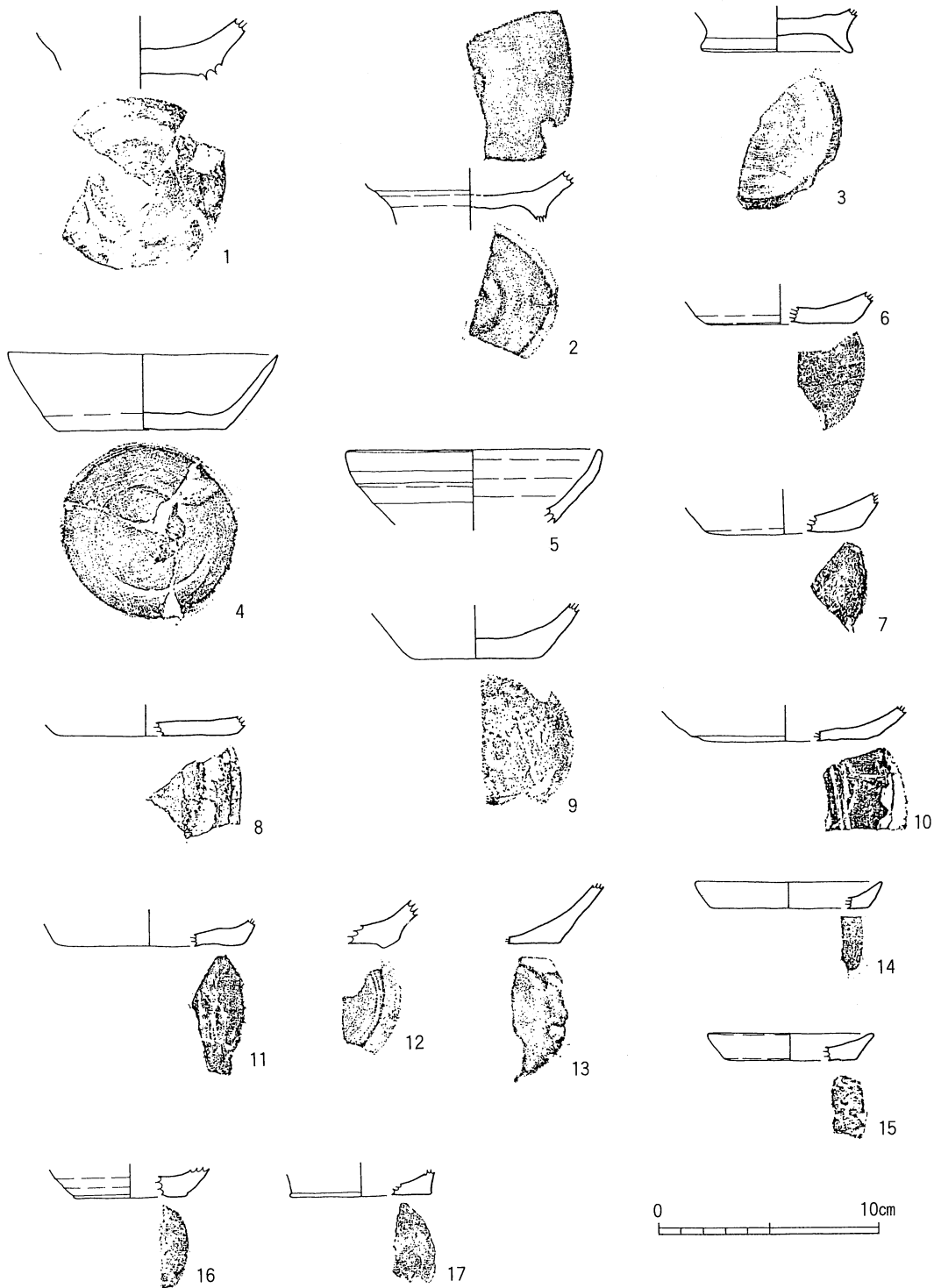
第19図 土師器実測図
