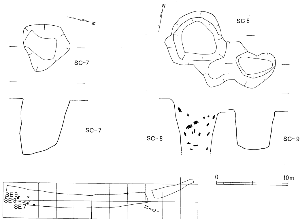
第6図 SC7・SC8・SC9 遺構実測図
