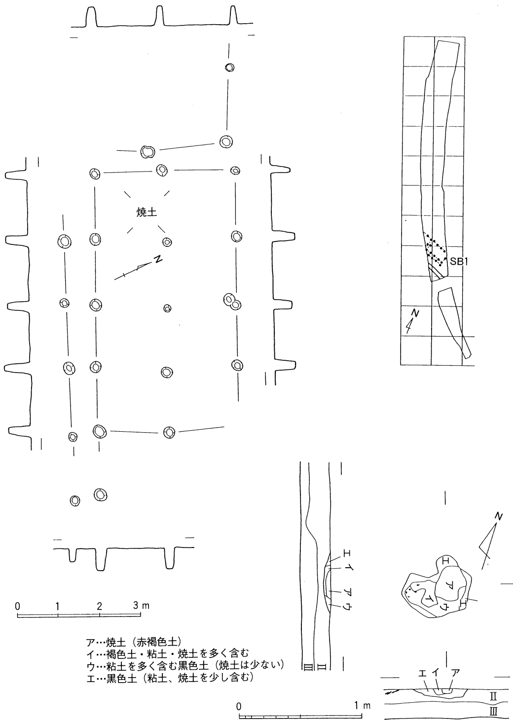
第17図 SB1遺構実測図
