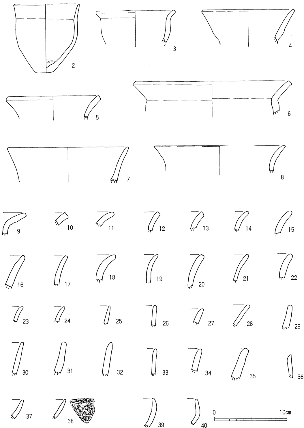
第12图 弥生土器实测图(1)
