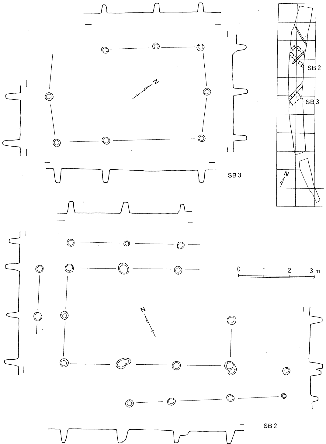
第18図 SB2・SB3遺構実測図
