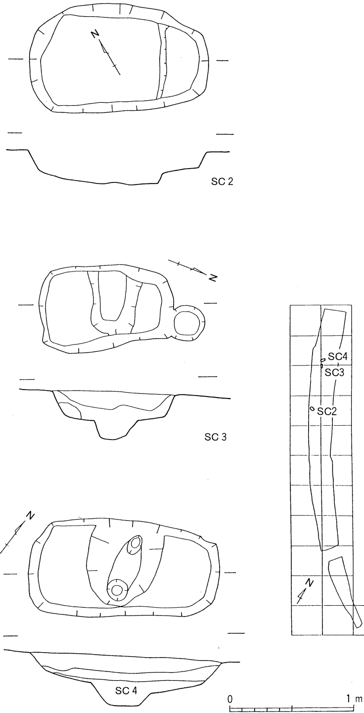
第22図 SC2・SC3・SC4遺構実測図
