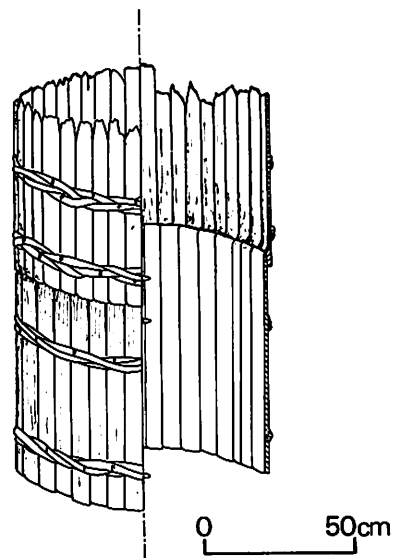
第9図 D2区第4号井戸復元図
