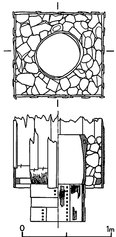
第3図 O O区第1号井戸復元図
