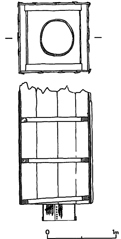
第5図 O4区第1号井戸復元図
