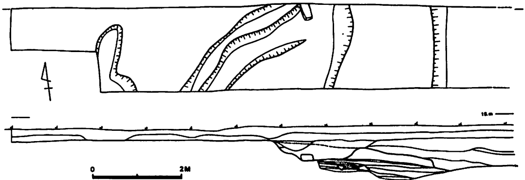
第3図 第5区東方建物基壇実測図
