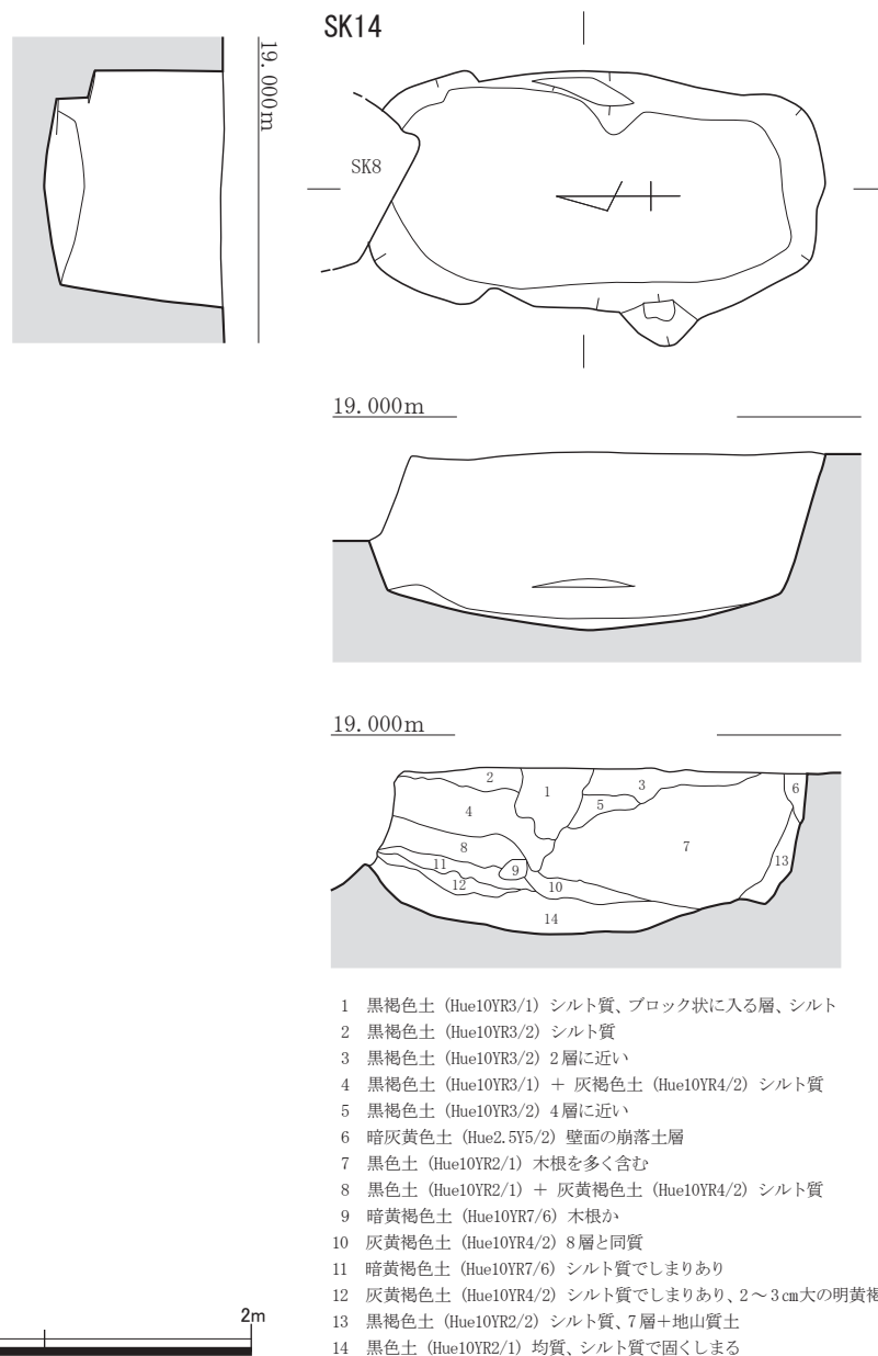
第13図 14号土坑実測図 (S=1/40)
