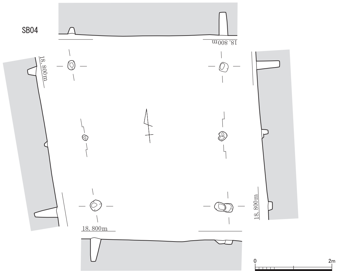
第5图 3·4号掘立柱建物实测图(S=1/60)
