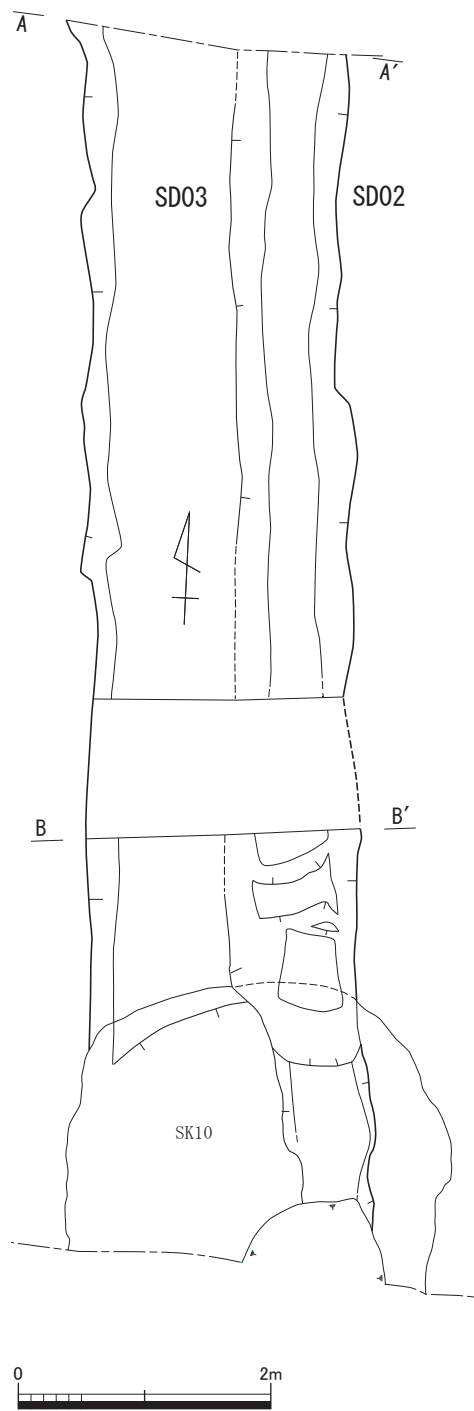
第16図 2・3号溝状遺構実測図 (S=1/60)
