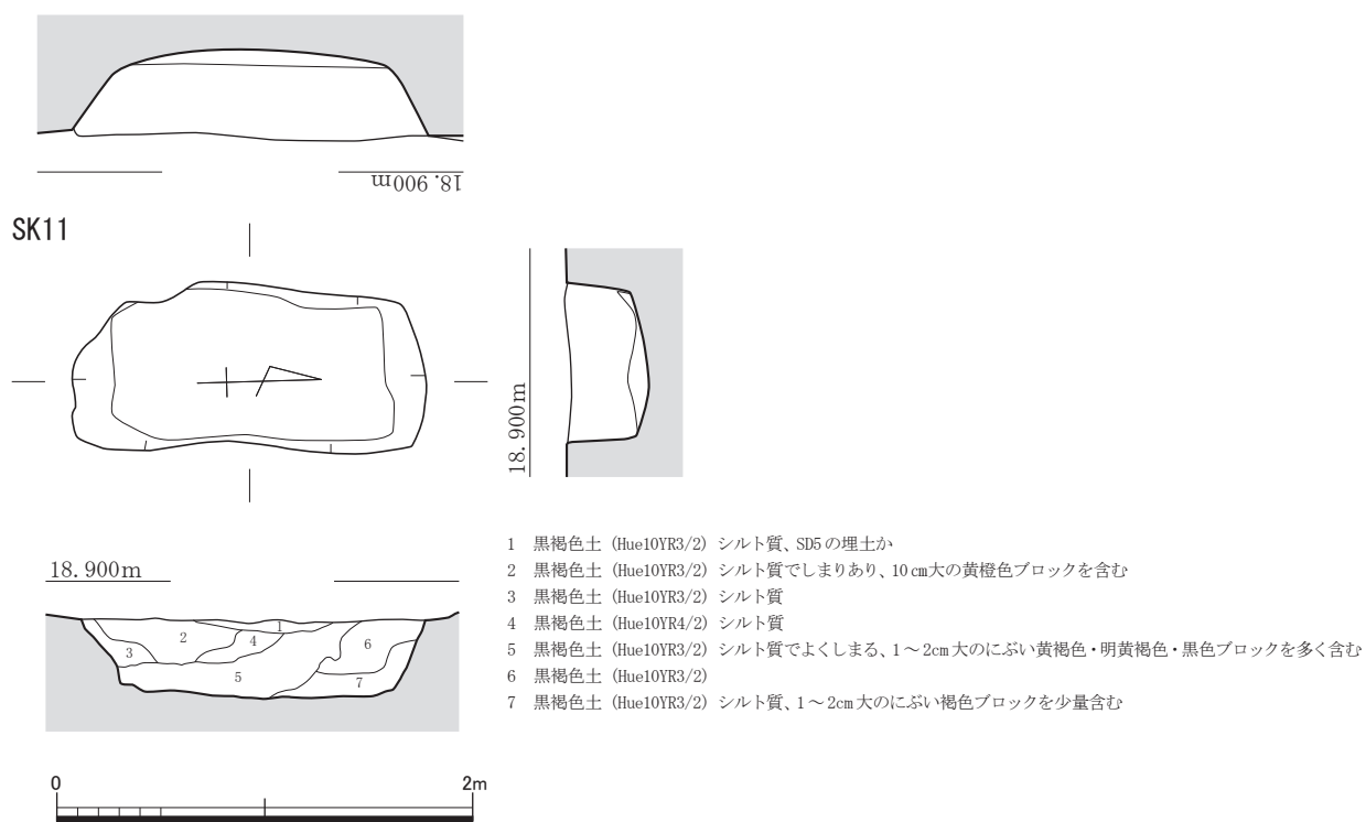
第12図 11号土坑実測図 (S=1/40)
