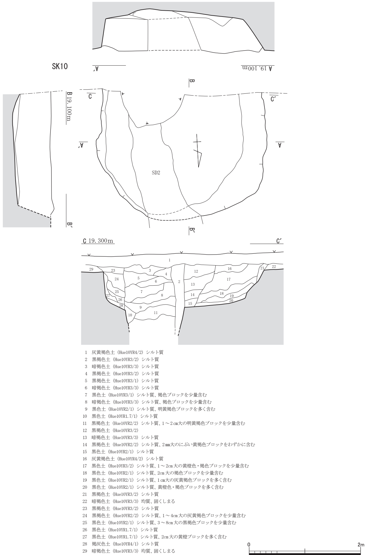
第 22 図 10 号土坑実測図 (S=1/40)
