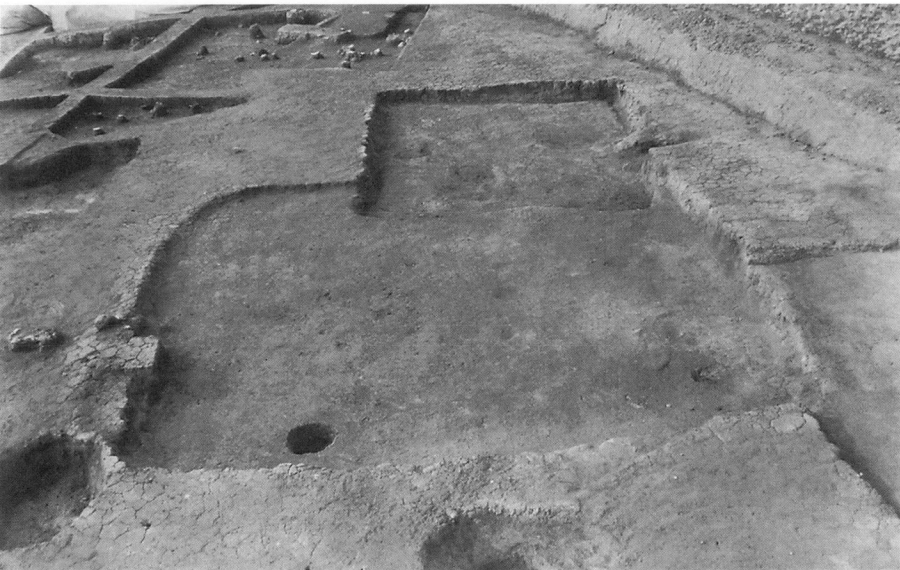
第32-A・B号住居跡 完掘状況
