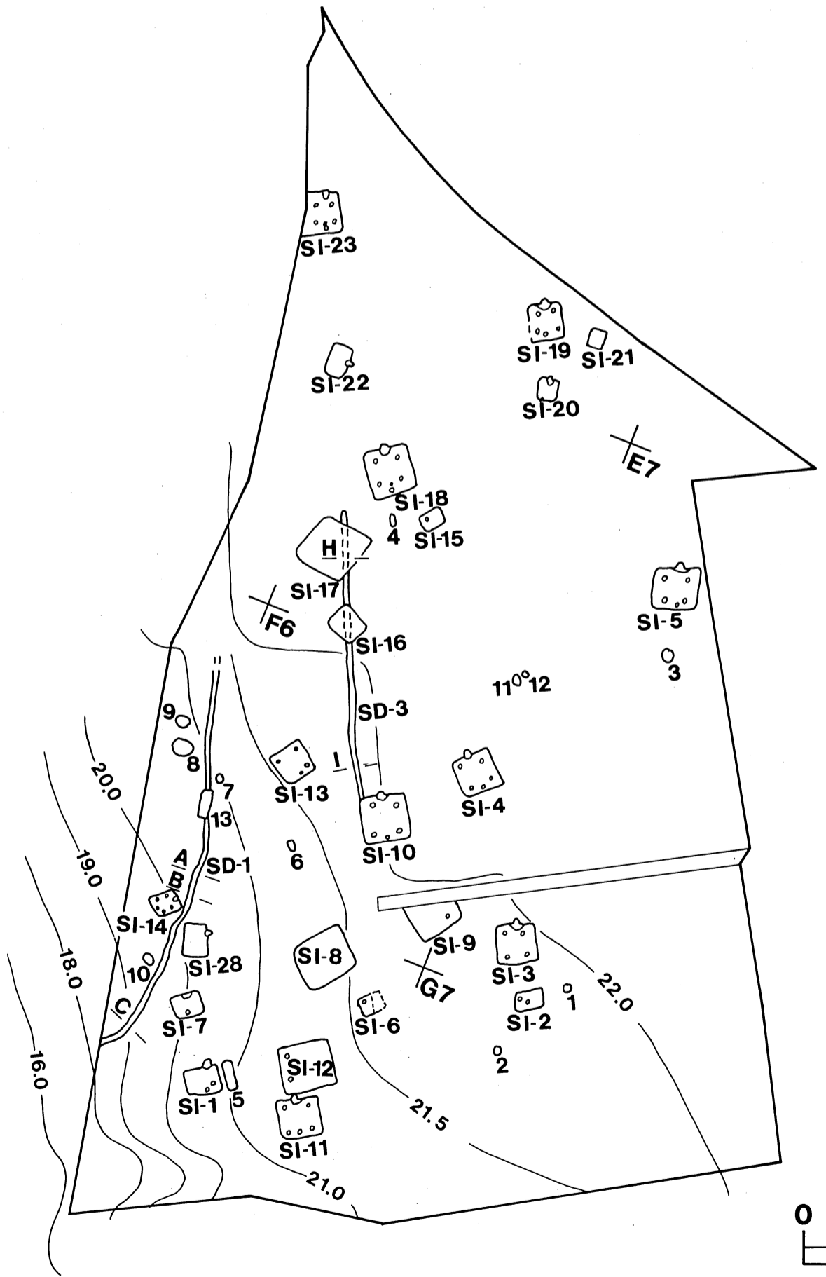
付図2 西栗山遺跡全体図
