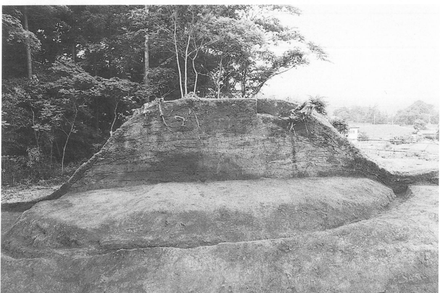
第3号塚土層断面（A-A'）
