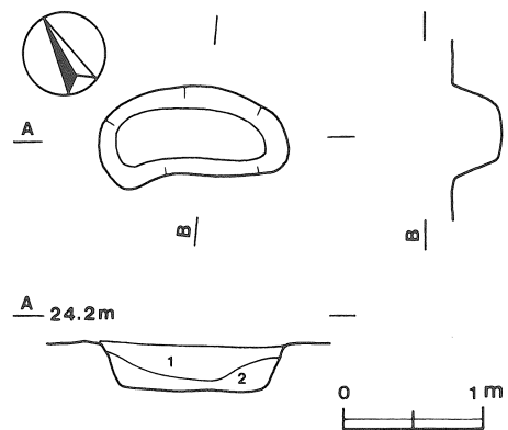
第25図 第1292号土坑実測図
