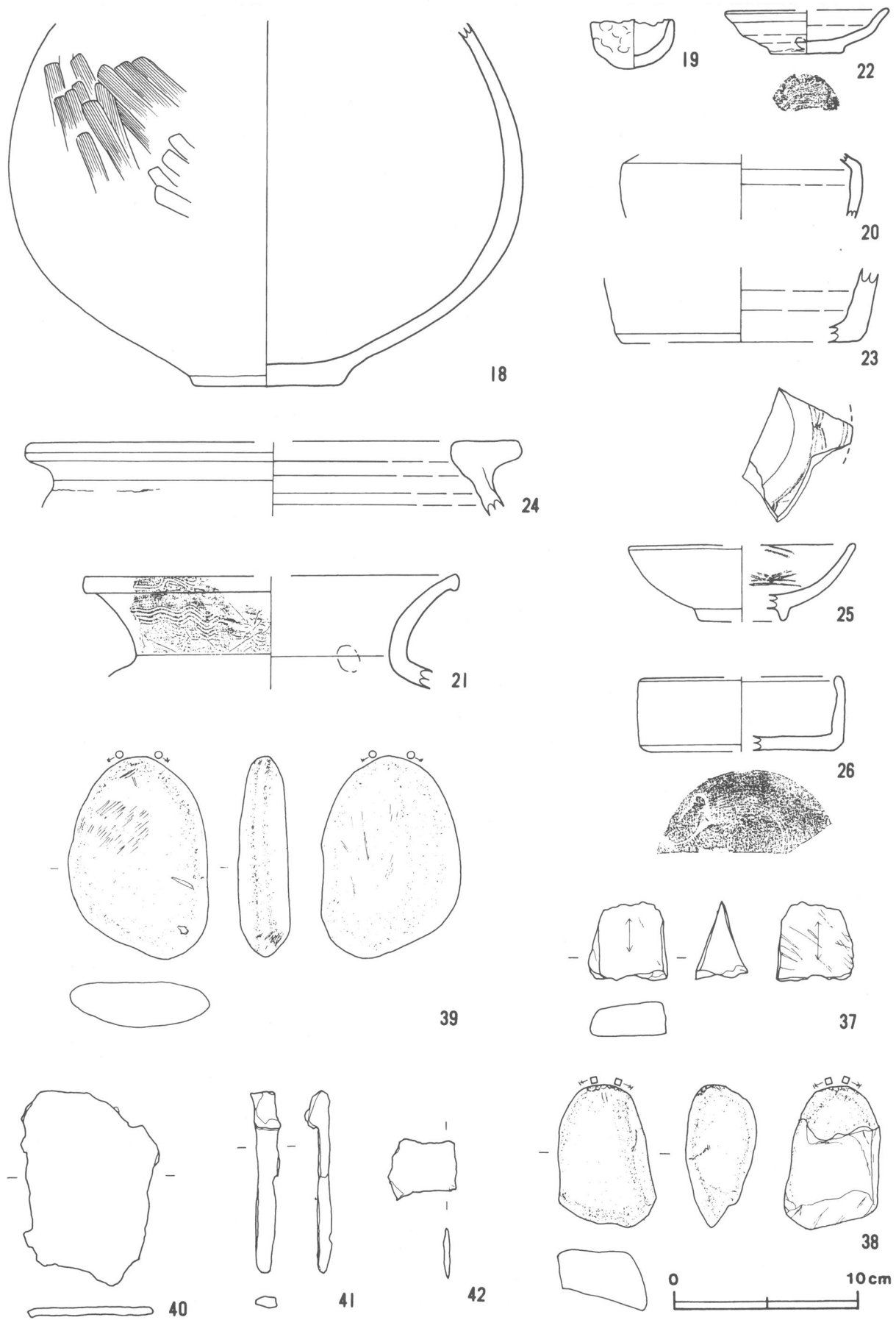
第19図 遺溝外出土遺物実測図(3)
