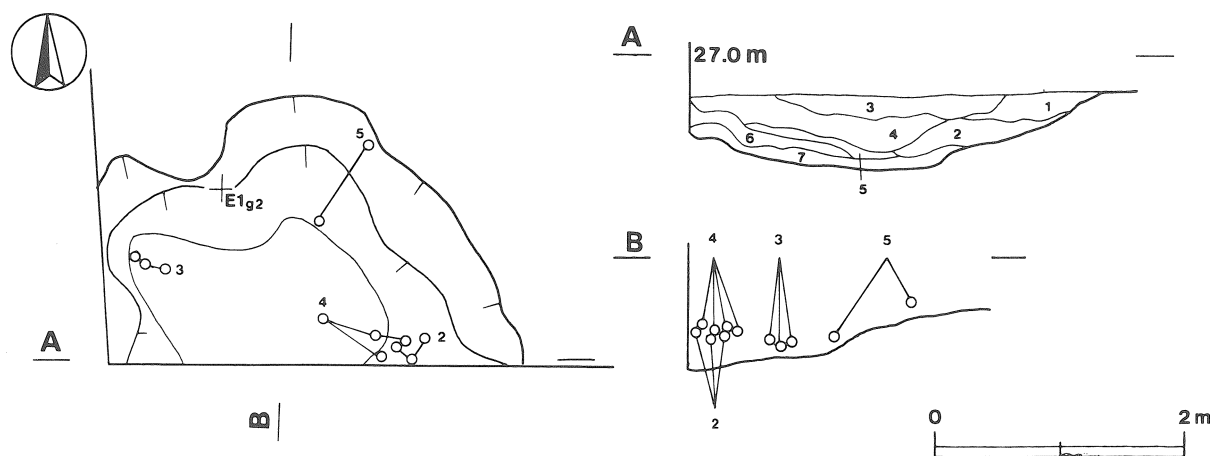
第4図 第37号墳実測図
