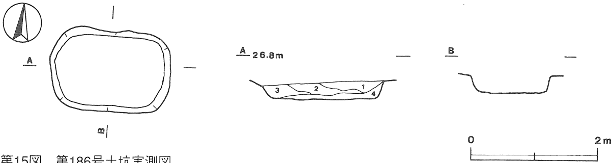
第15図 第186号土坑実測図
