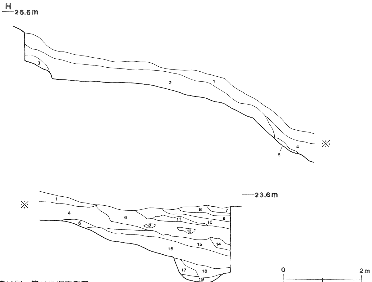
第13図 第42号堀実測図
