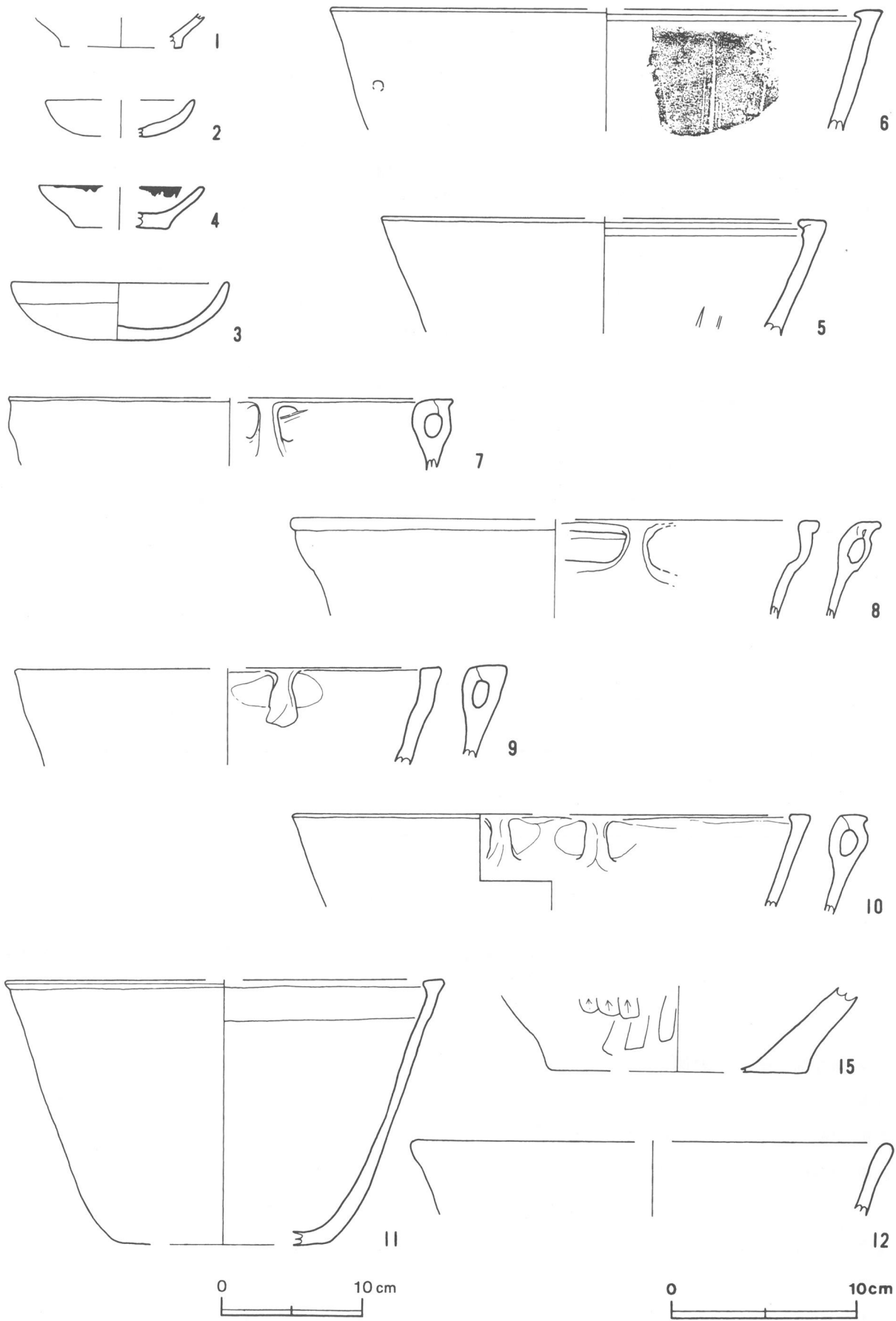
第23图 第3·4号土壘出土遺物実測図(1)
