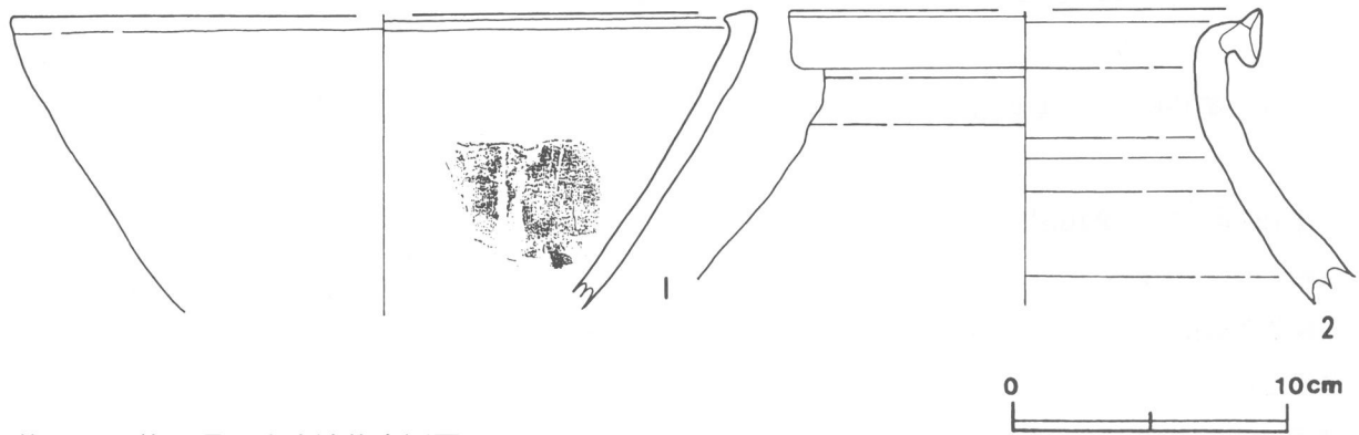
第14図 第42号堀出土遺物実測図
