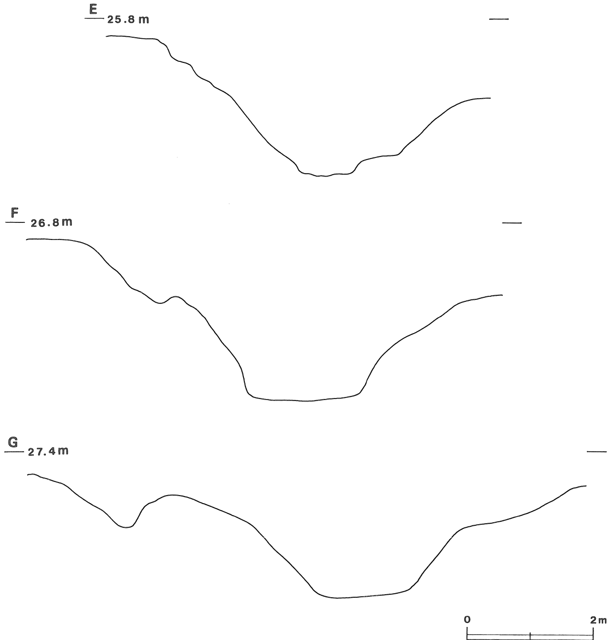
第11図 第37号堀実測図(2)
