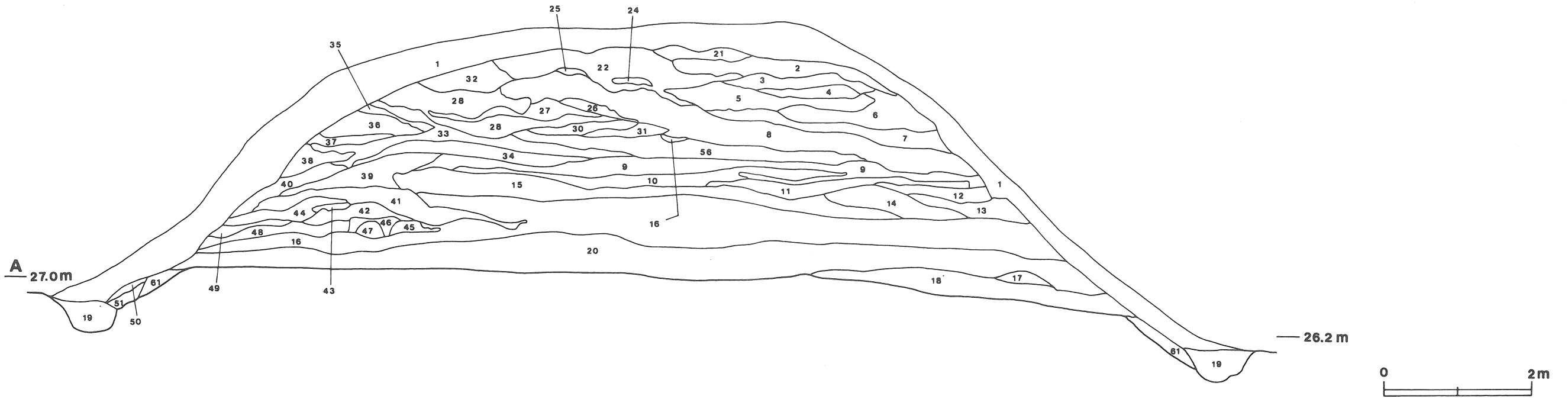
第8图 第3号塚实测图
