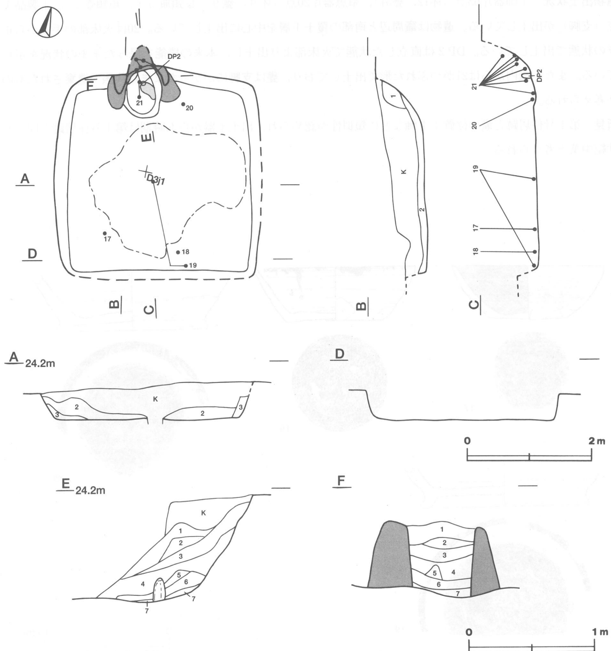
第7図 第3号住居跡実測図
