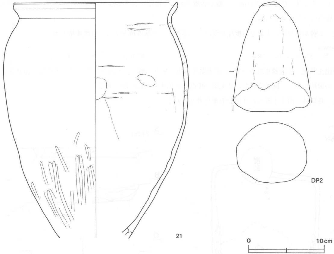
第9図 第3号住居跡出土遺物実測図(2)
