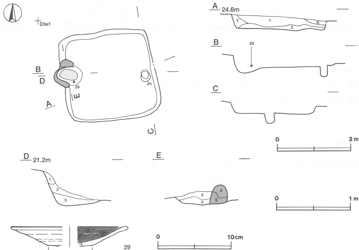
第13図 第7号住居跡・出土遺物実測図
