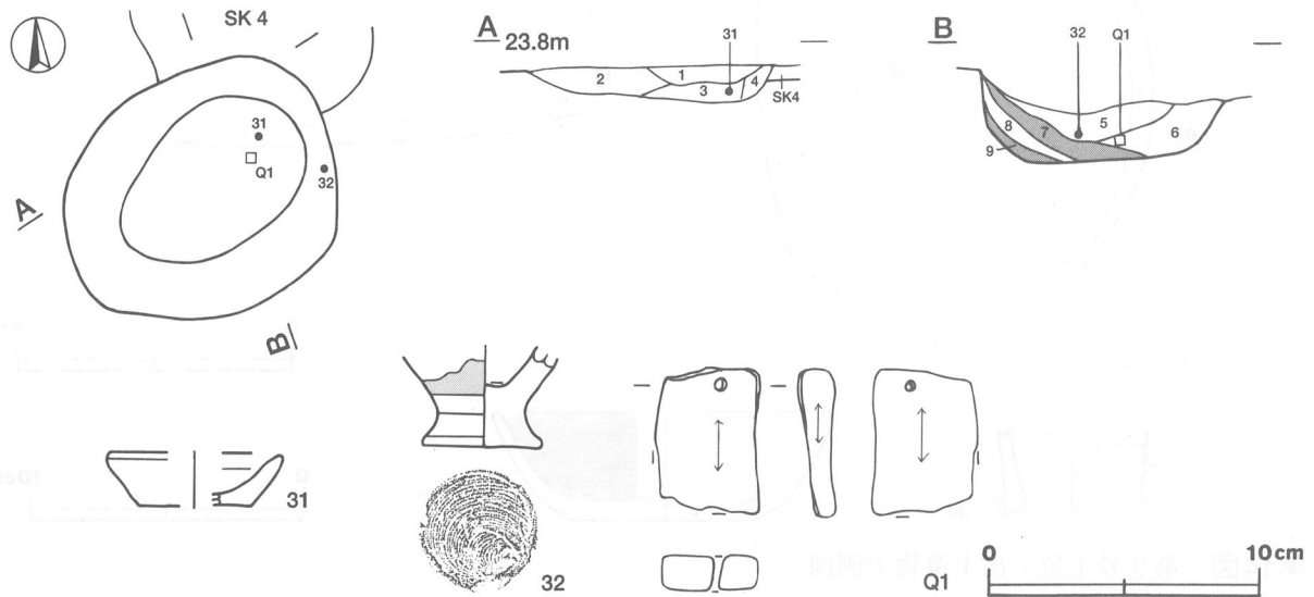
第15図 第3号土坑・出土遺物実測図
