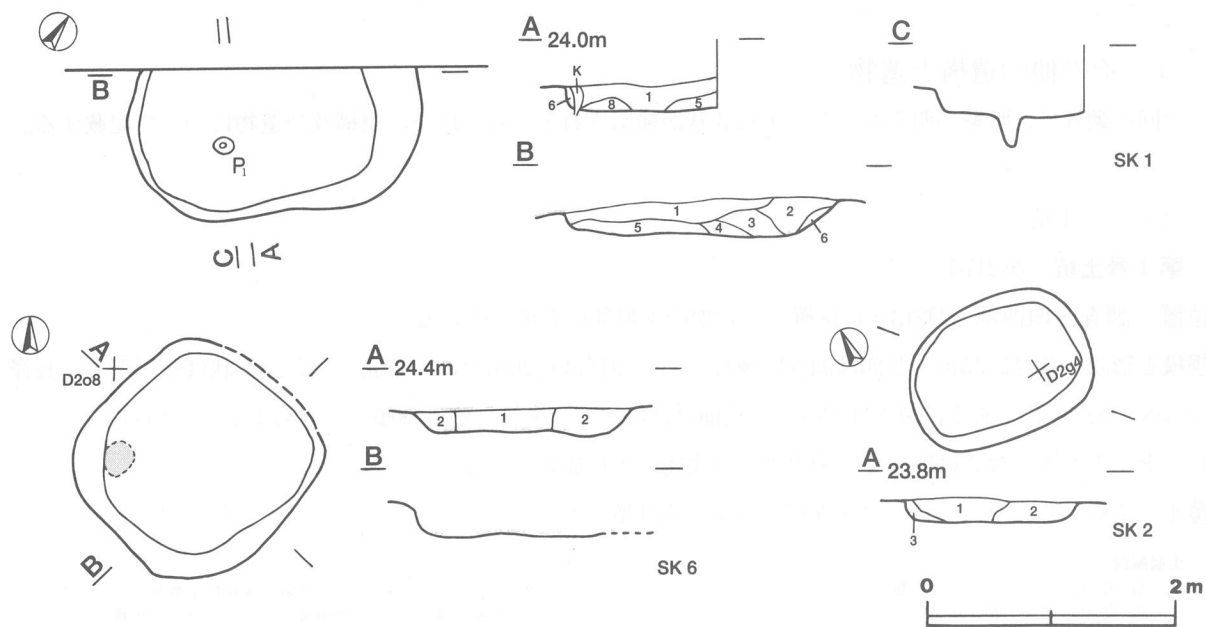
第21図 第1・2・6号土坑実測図
