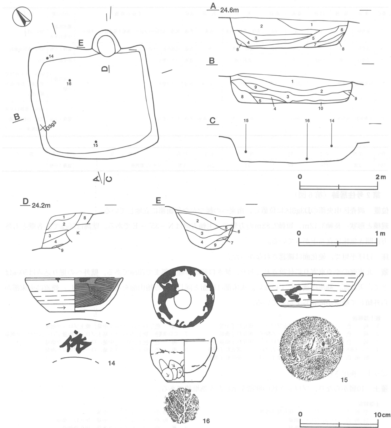
第6図 第2号住居跡・出土遺物実測図
