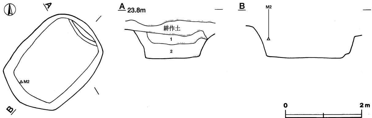
第19図 第10号土坑実測図
