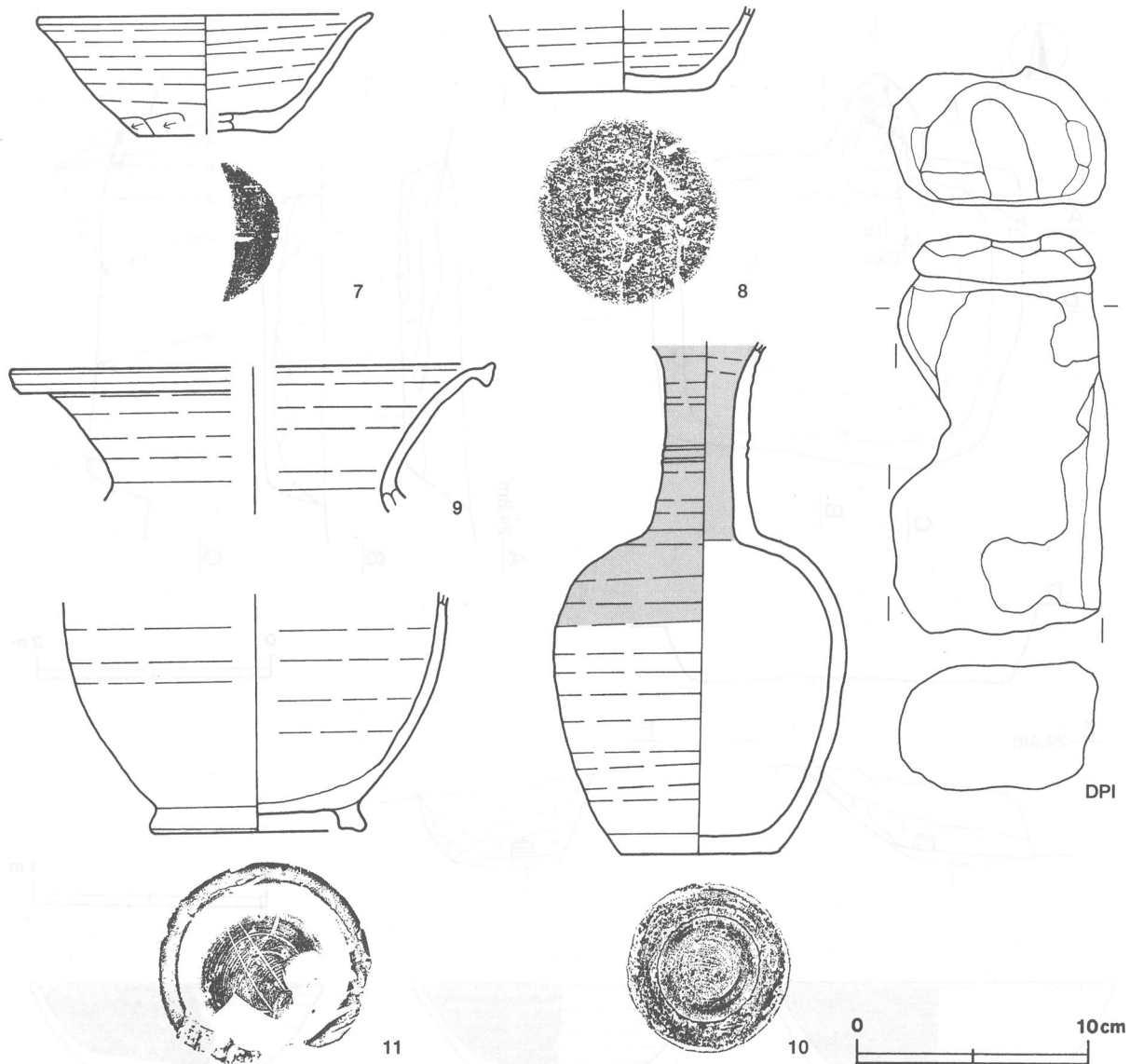
第5図 第1号住居跡出土遺物実測図
