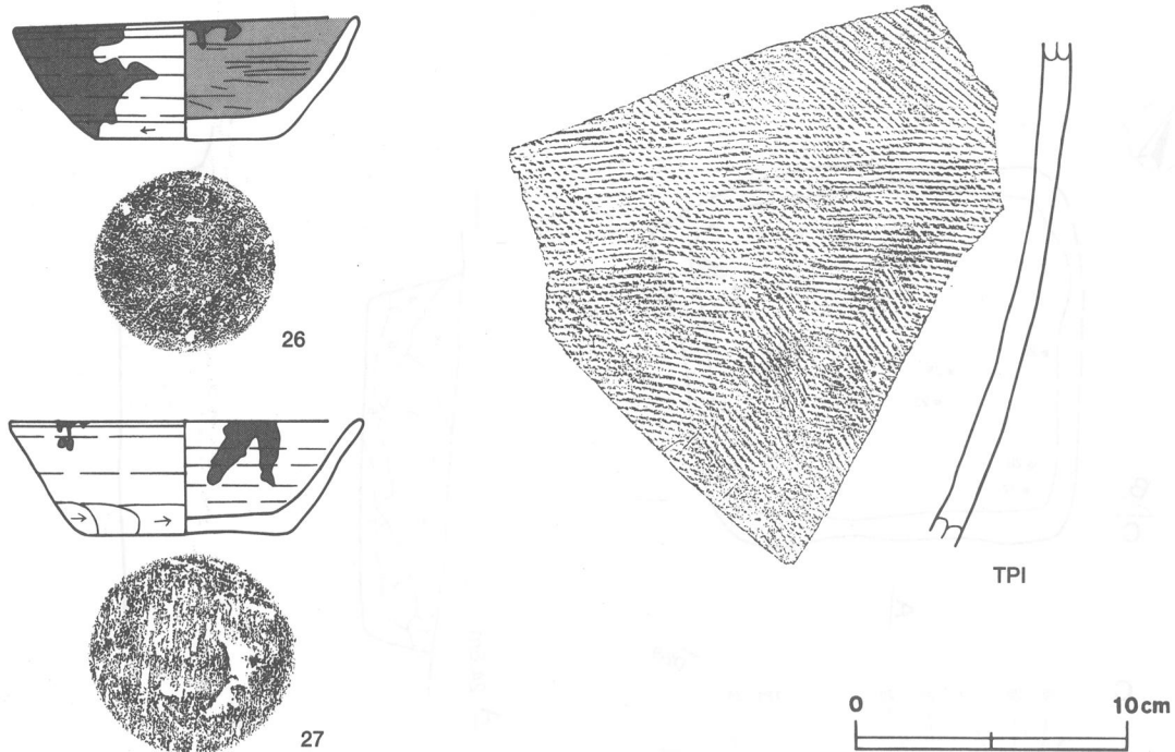
第12図 第6号住居跡出土遺物実測図
