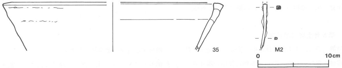
第20図 第10号土坑出土遺物実測図
