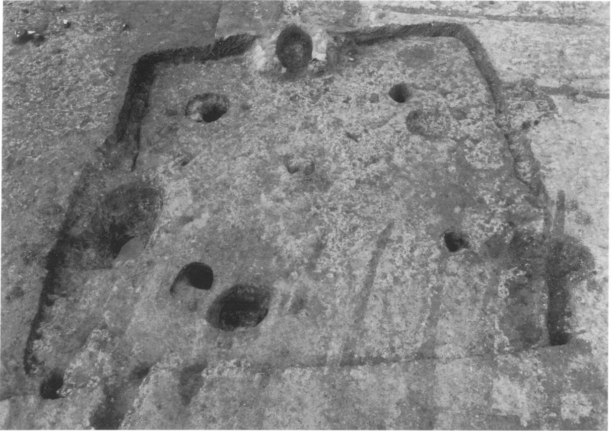
第56号住居跡完掘状況
