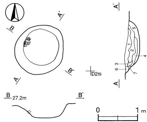
第12図 第30号土坑実測図
