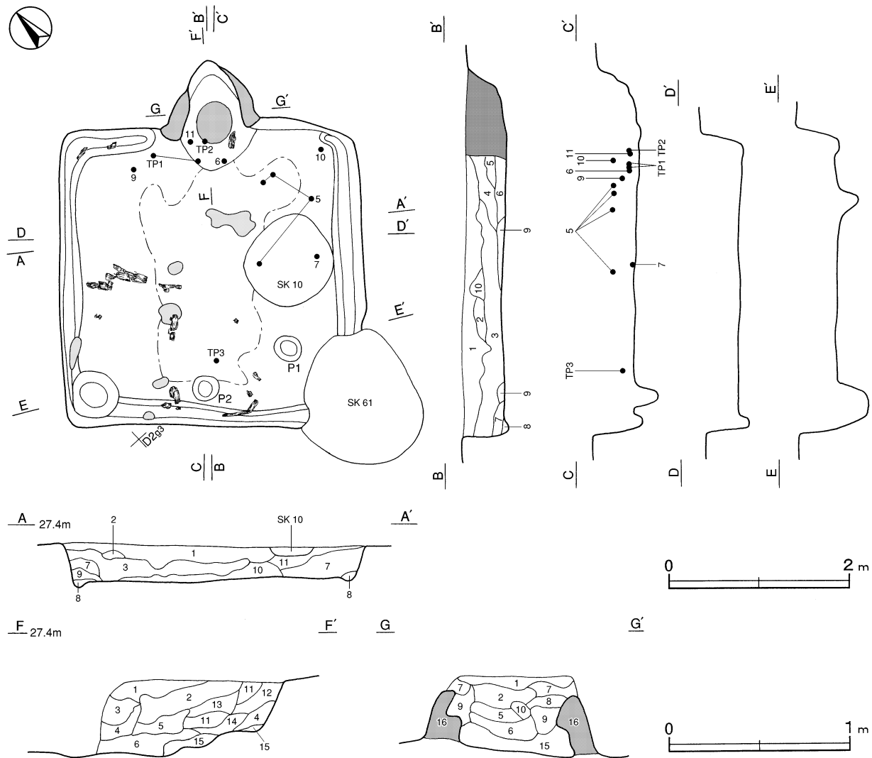
第6図 第2号住居跡実測図
