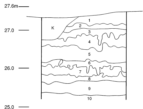
第3図 基本土層図
