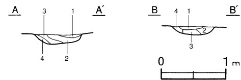
第13図 第1号溝跡実測図
