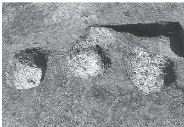
第3～5号墓坑完掘状况
