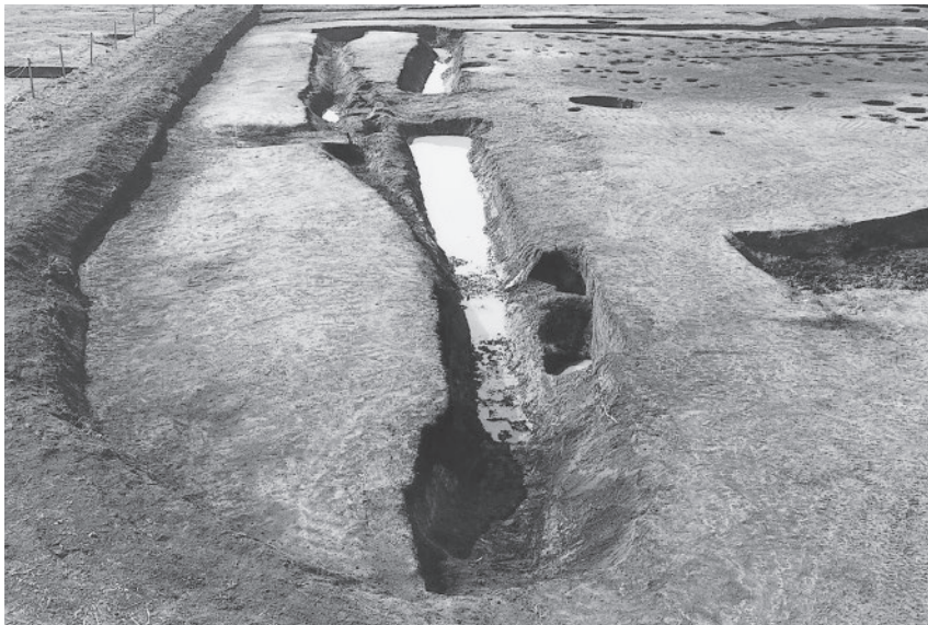
第28A・28B・29号溝跡 完掘状況(北から)
