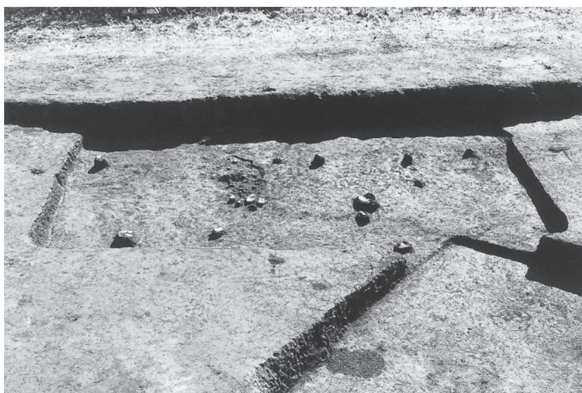
第 126 号 住居 跡 遺 物 出 土 状 況 (西 から)
