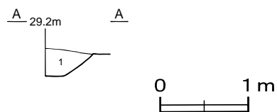
第18図 第6号溝跡実測図
