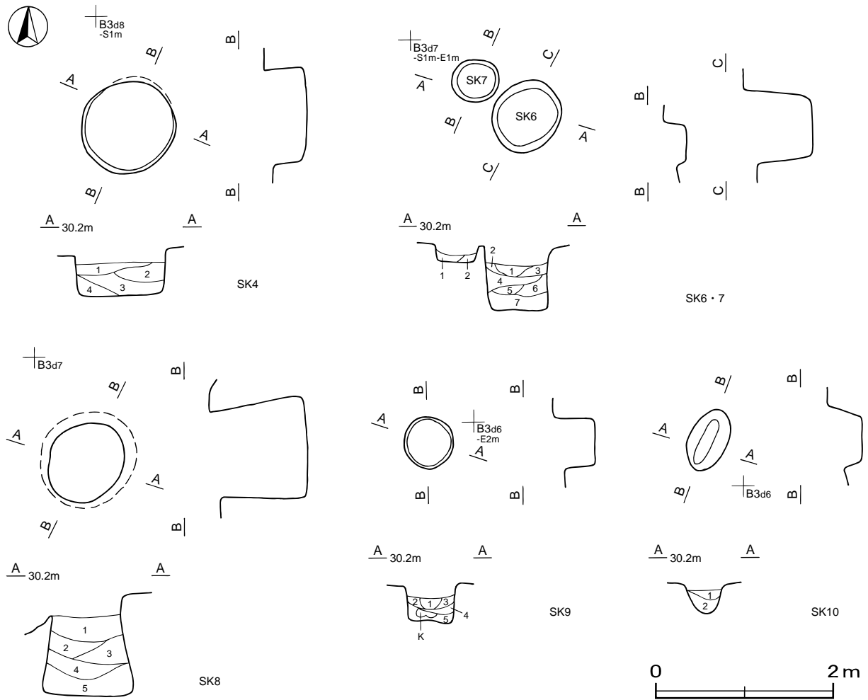
第30図 その他の土坑実測図
