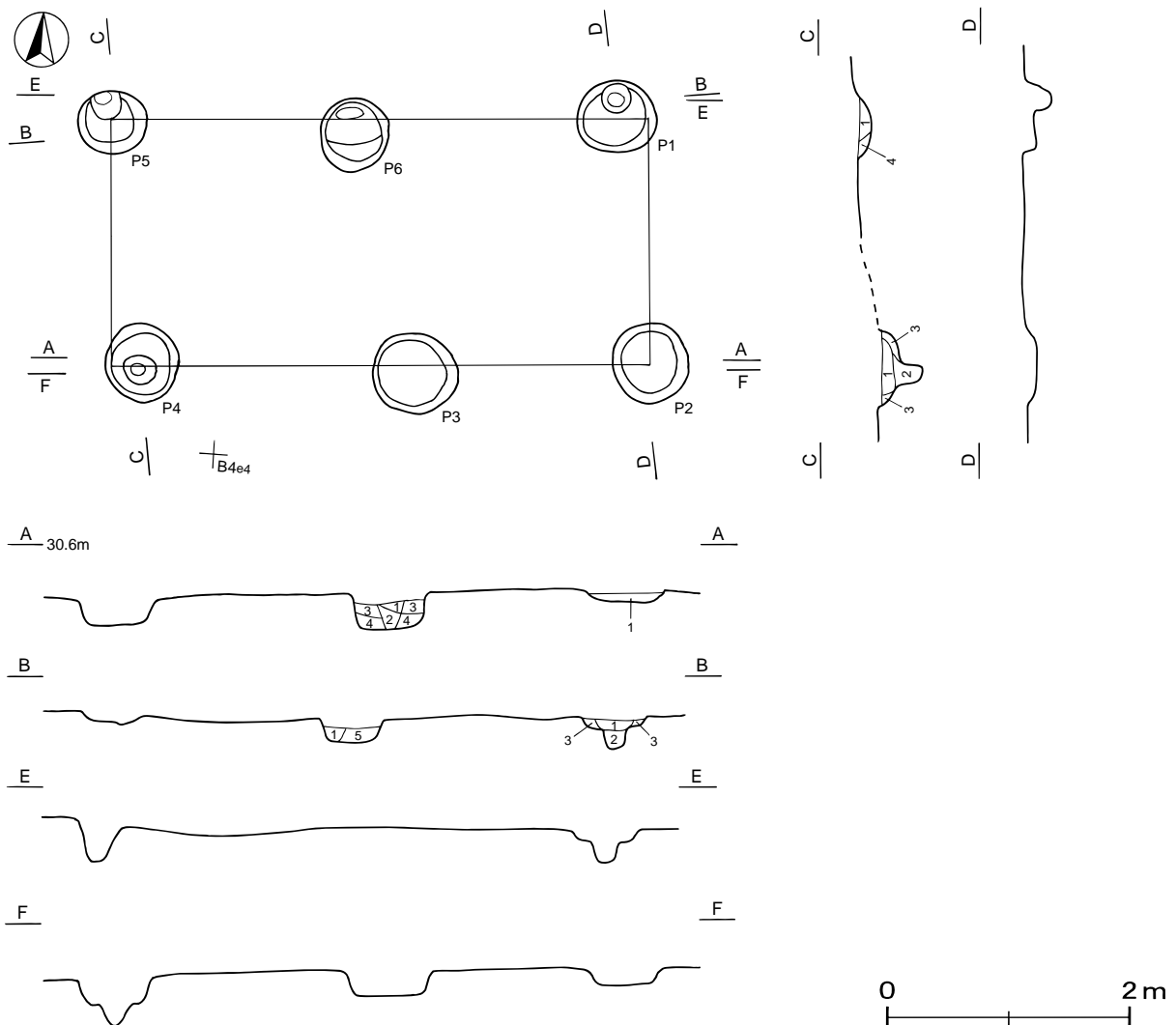
第25図 第2号掘立柱建物跡実測図
