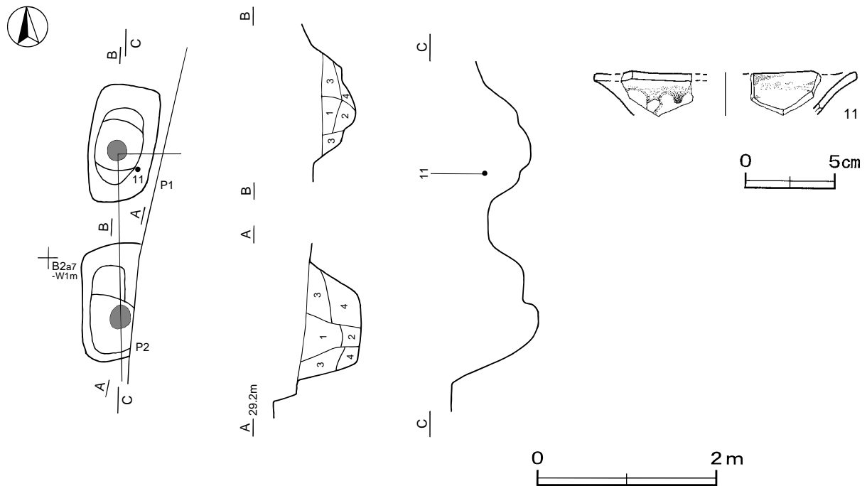
第 9 図 第 4 号掘立柱建物跡・出土遺物実測図
