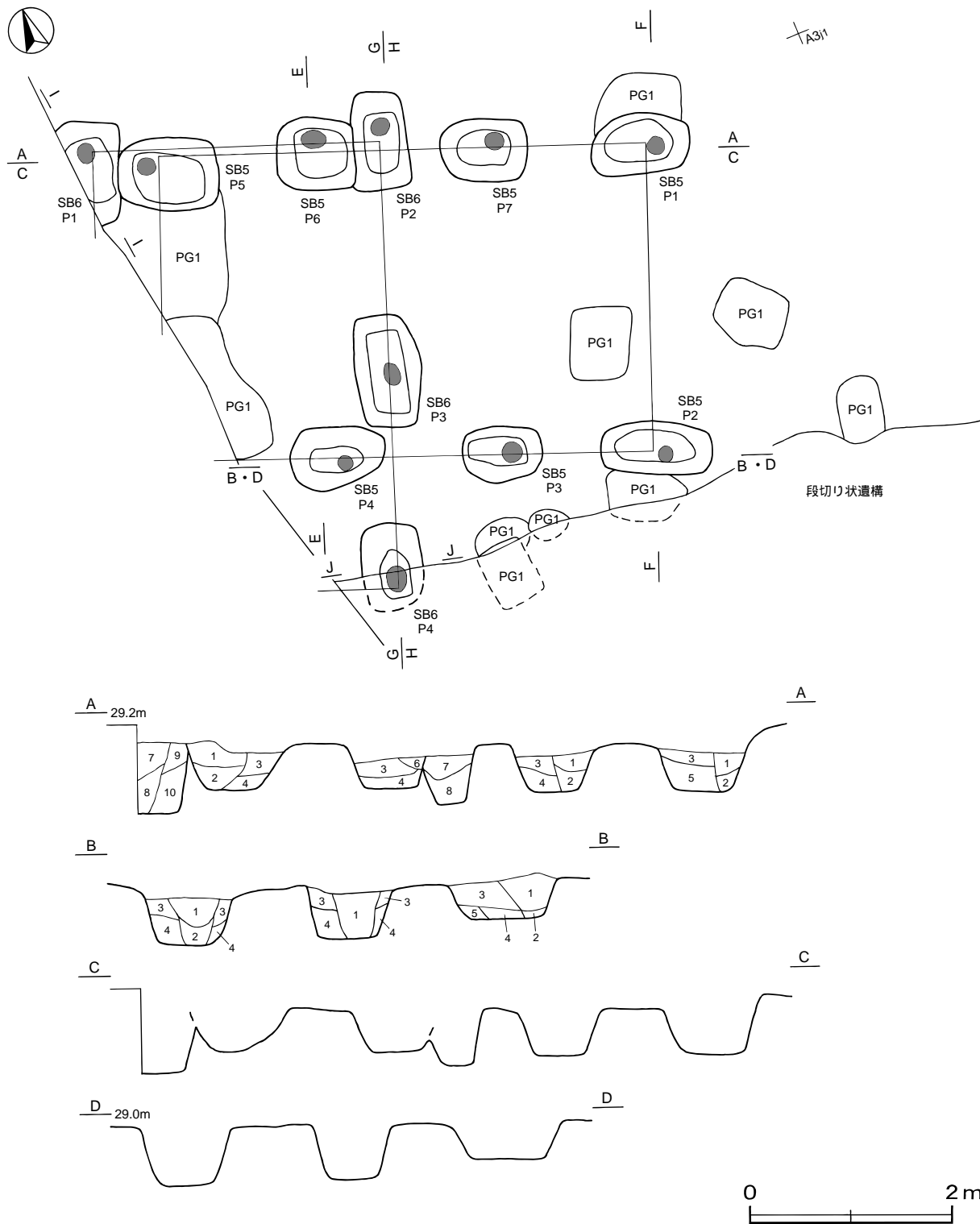
第10図 第5・6号掘立柱建物跡実測図
