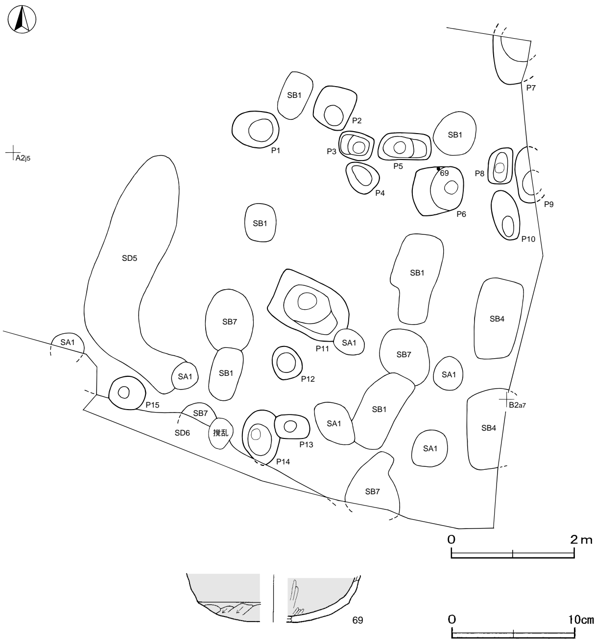
第32図 第2号ピット群・出土遺物実測図
