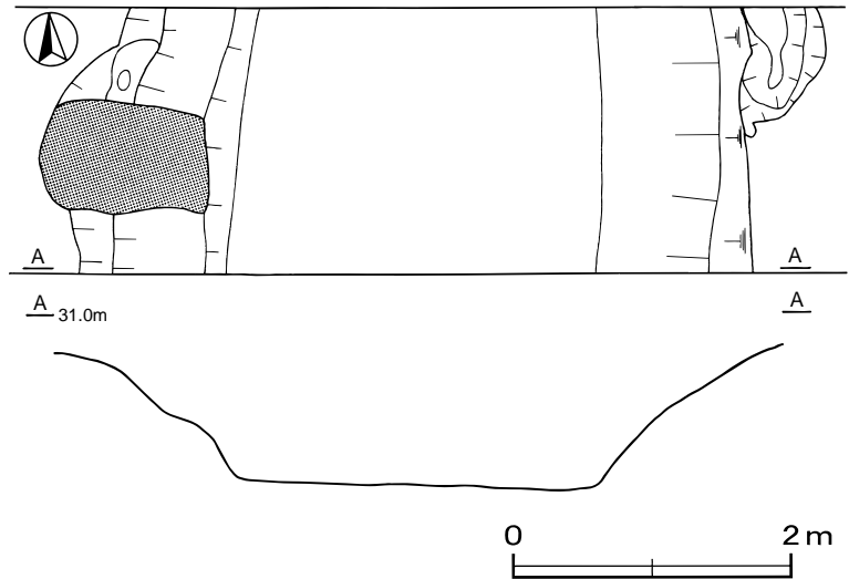
第35図 KT20遺跡大溝実測図（「鹿島町内遺跡発掘調査報告書」より抜粋 一部改変再トレース）
