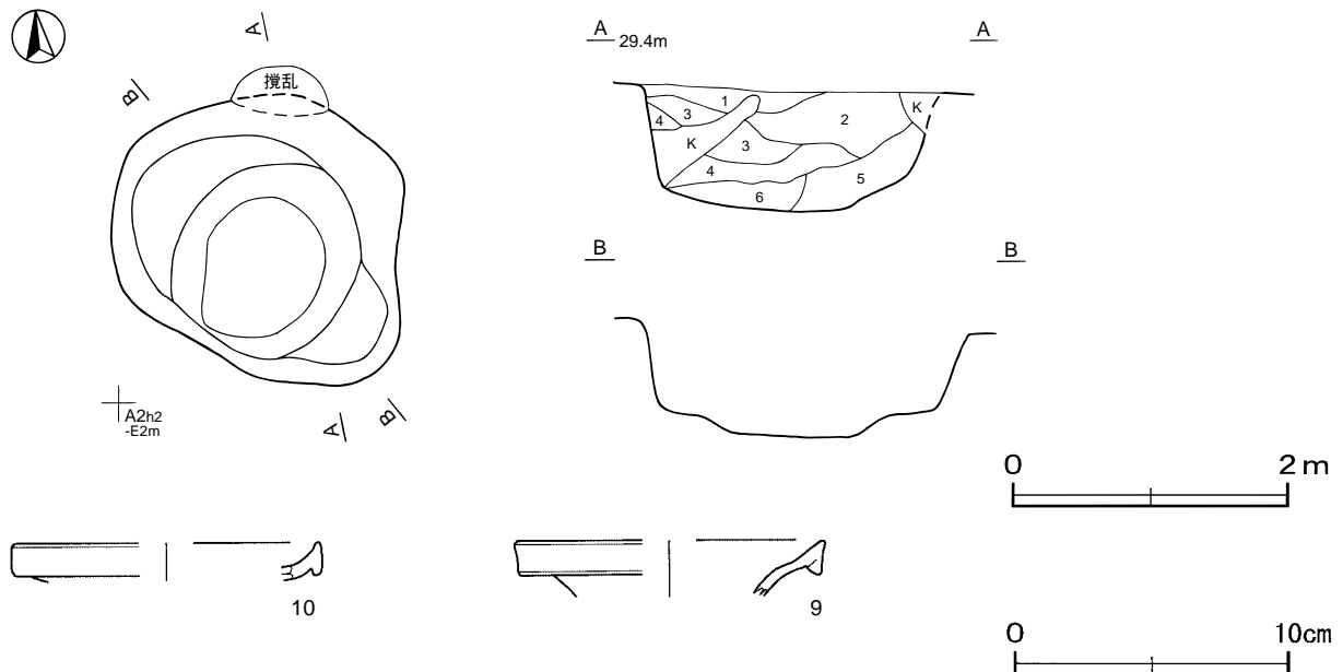
第7図 第2号土坑・出土遺物実測図
