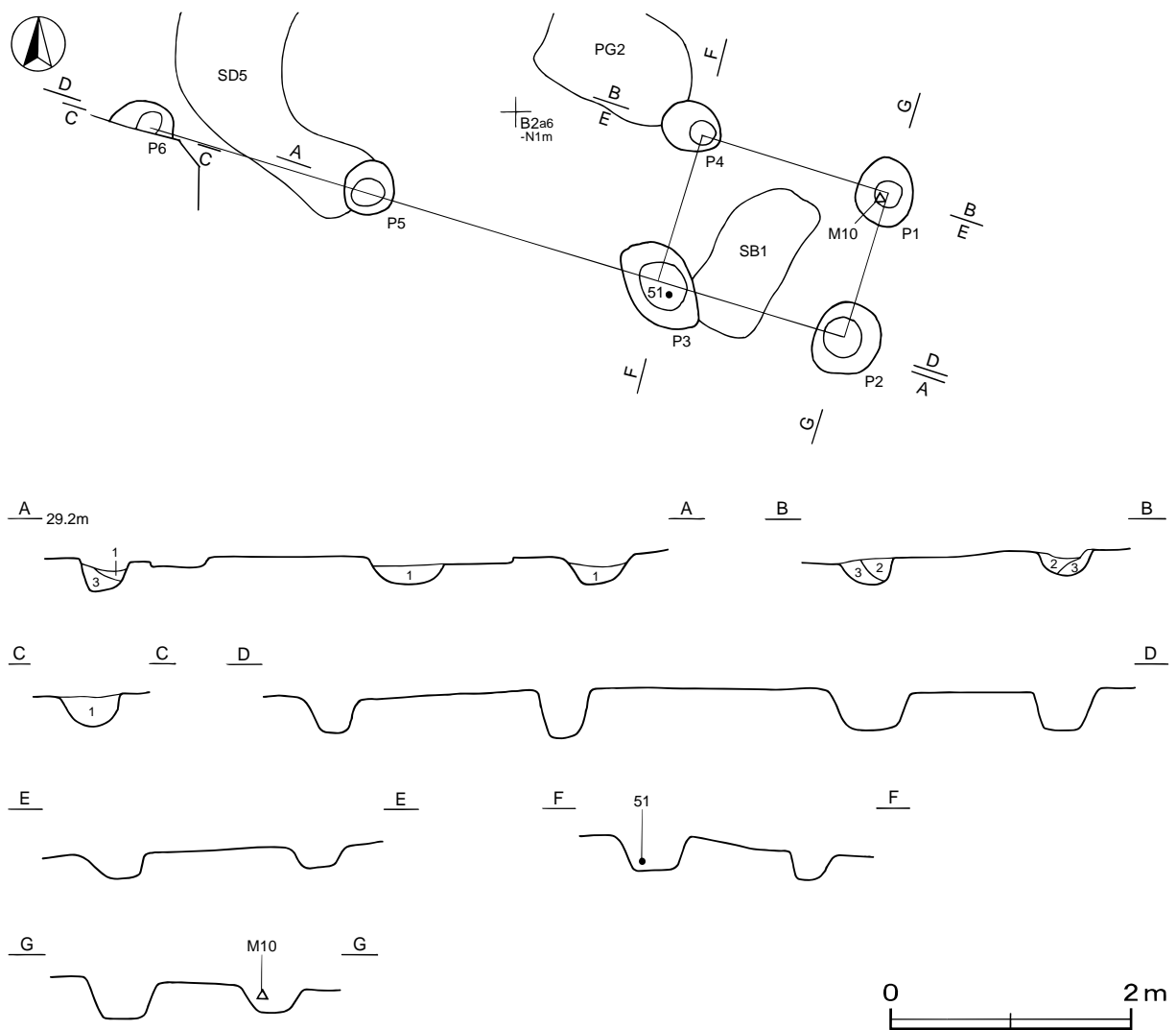
第20図 第1号柵跡実測図
