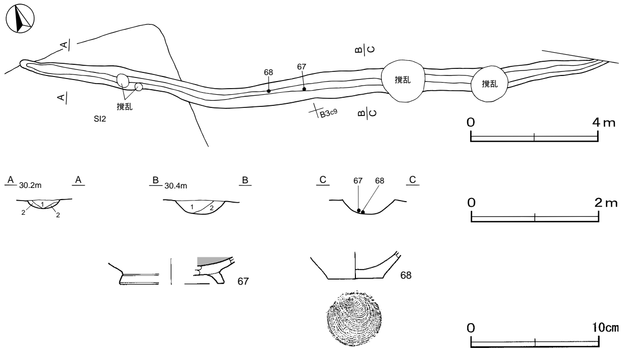
第28図 第4号溝跡・出土遺物実測図
