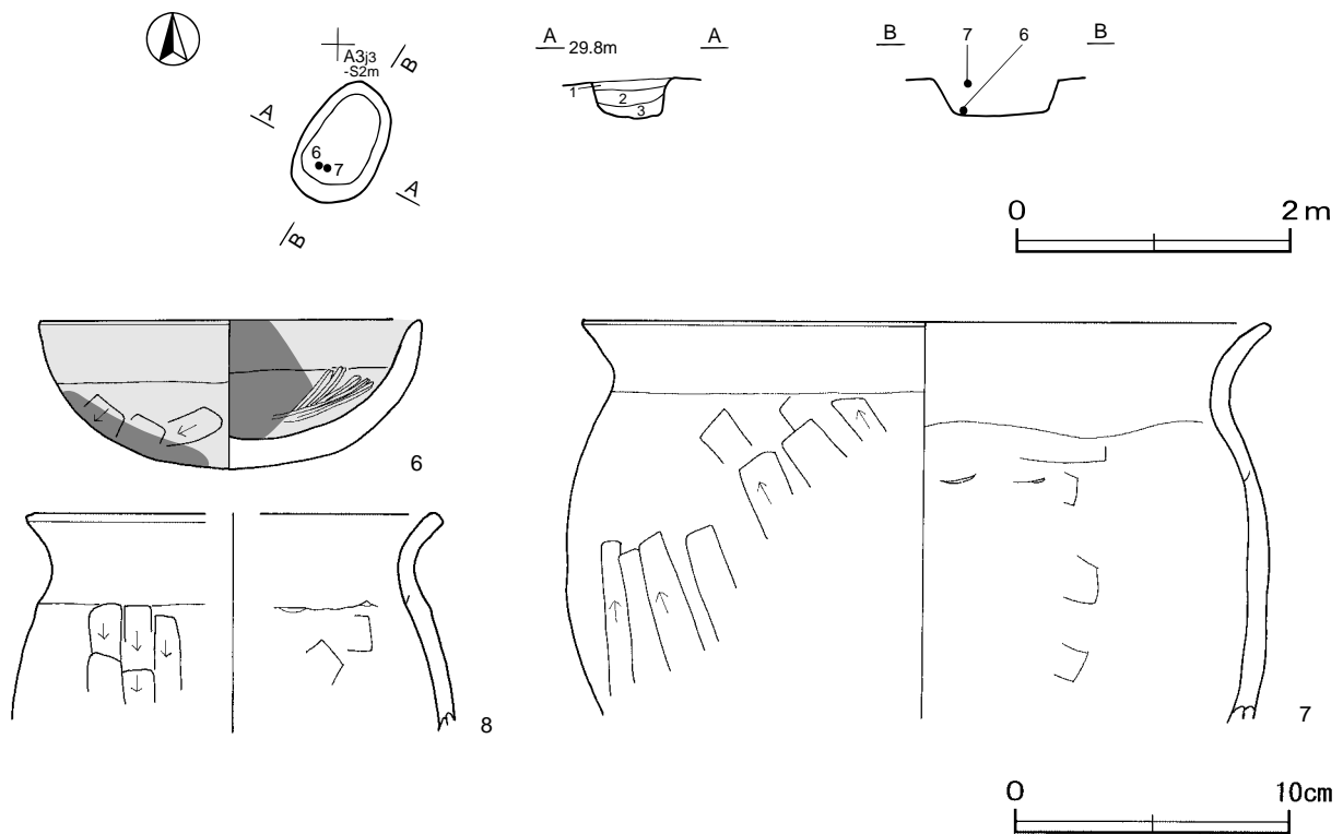
第6図 第1号土坑・出土遺物実測図
