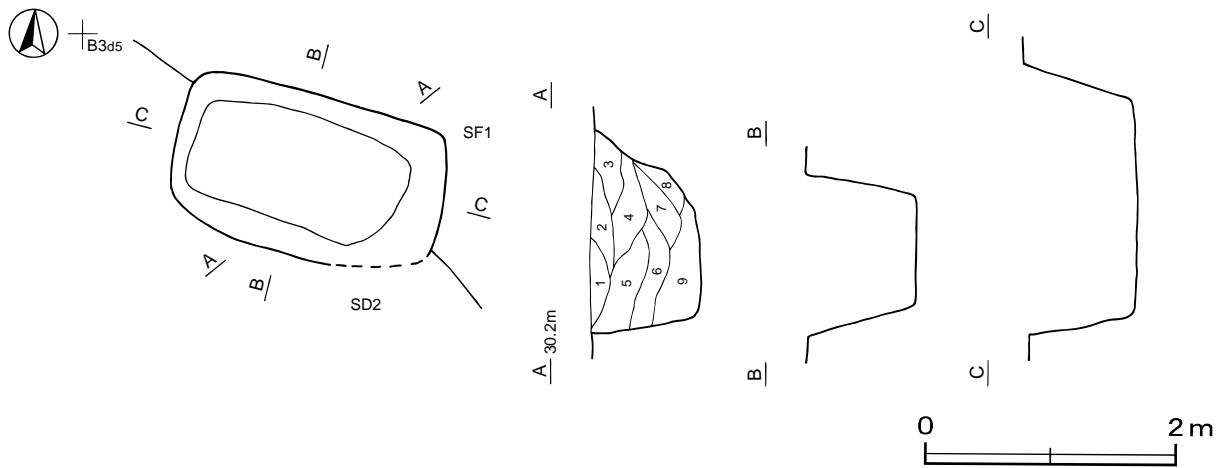
第29図 第5号土坑実測図
