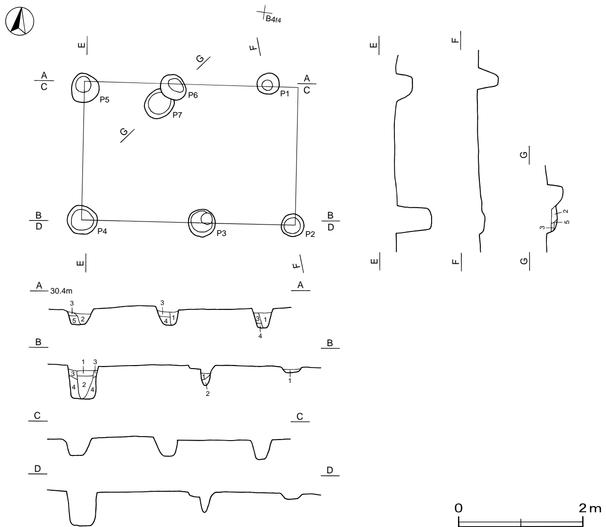
第26図 第3号掘立柱建物跡実測図
