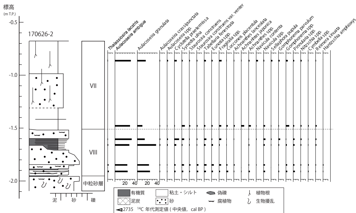
図6 南壁面の地点170626-2における地質柱状図および珪藻分析結果
