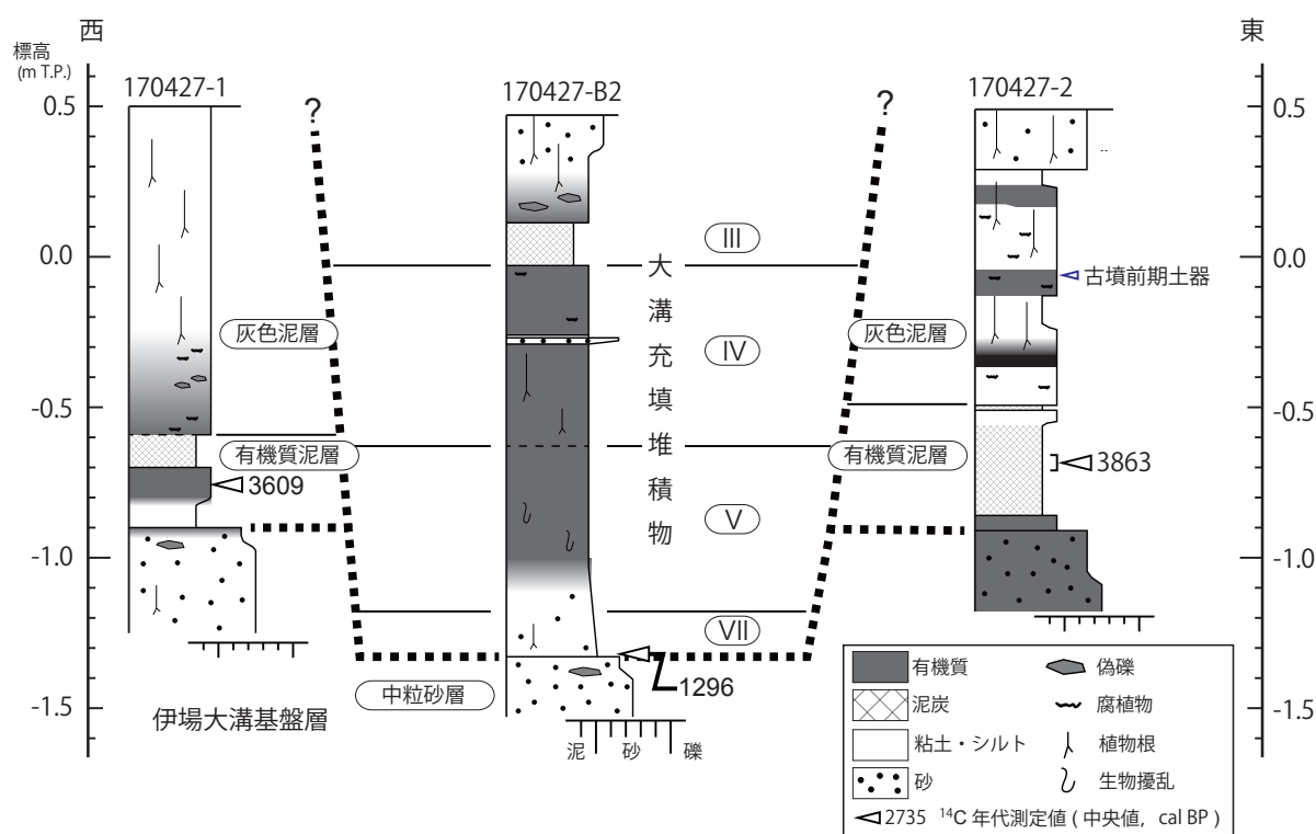
図 3 ベルト II における地質柱状図
