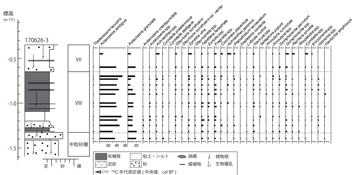
図 7 西壁面（地点 170626-3）における地質柱状図および珪藻分析結果
