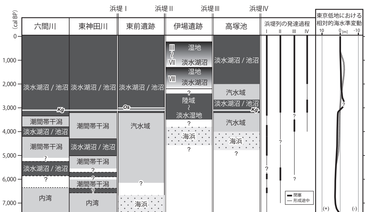
図 9 梶子遺跡周辺における伊場大溝の堆積環境変遷と浜松平野西部における浜堤列の地形発達過程
