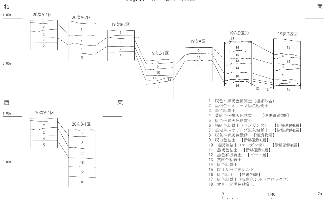
Fig. 18 土層柱状図
