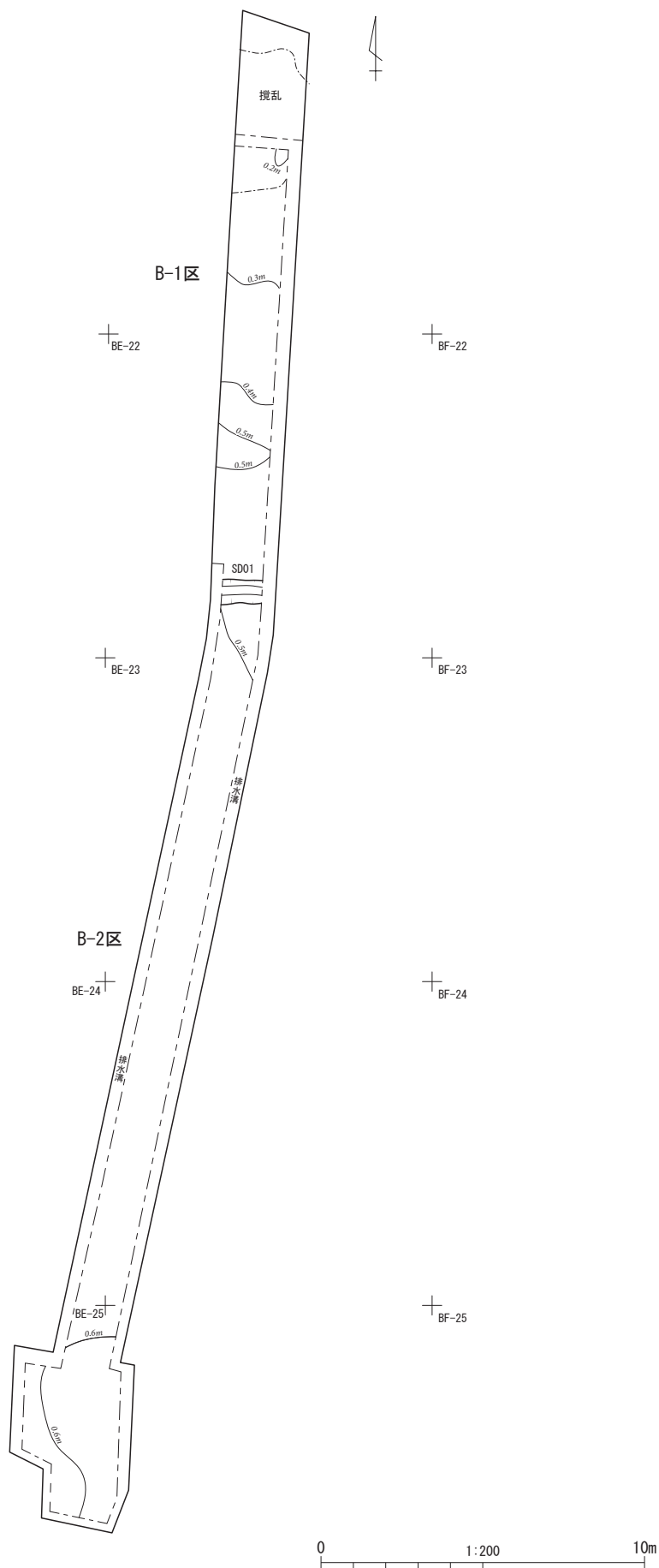
Fig. 33 B区 上層遺構全体図
