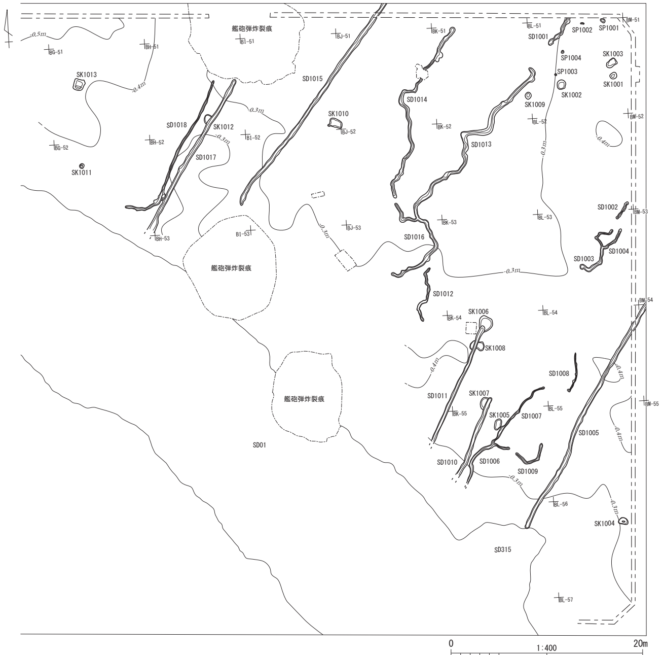
Fig. 43 D区 下層 遺構全体図
