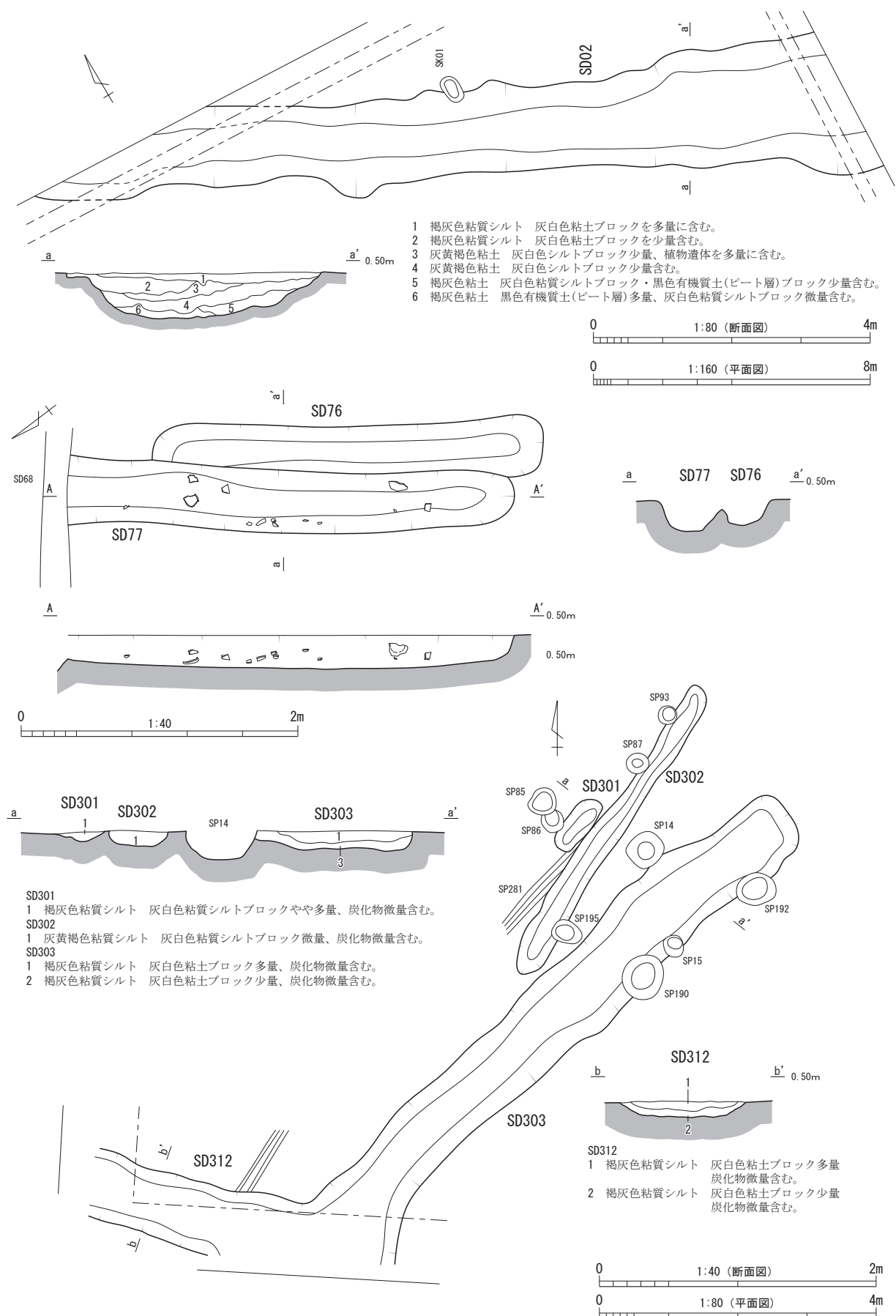
Fig. 55 SD02・76・77・301～303・312 実測図
