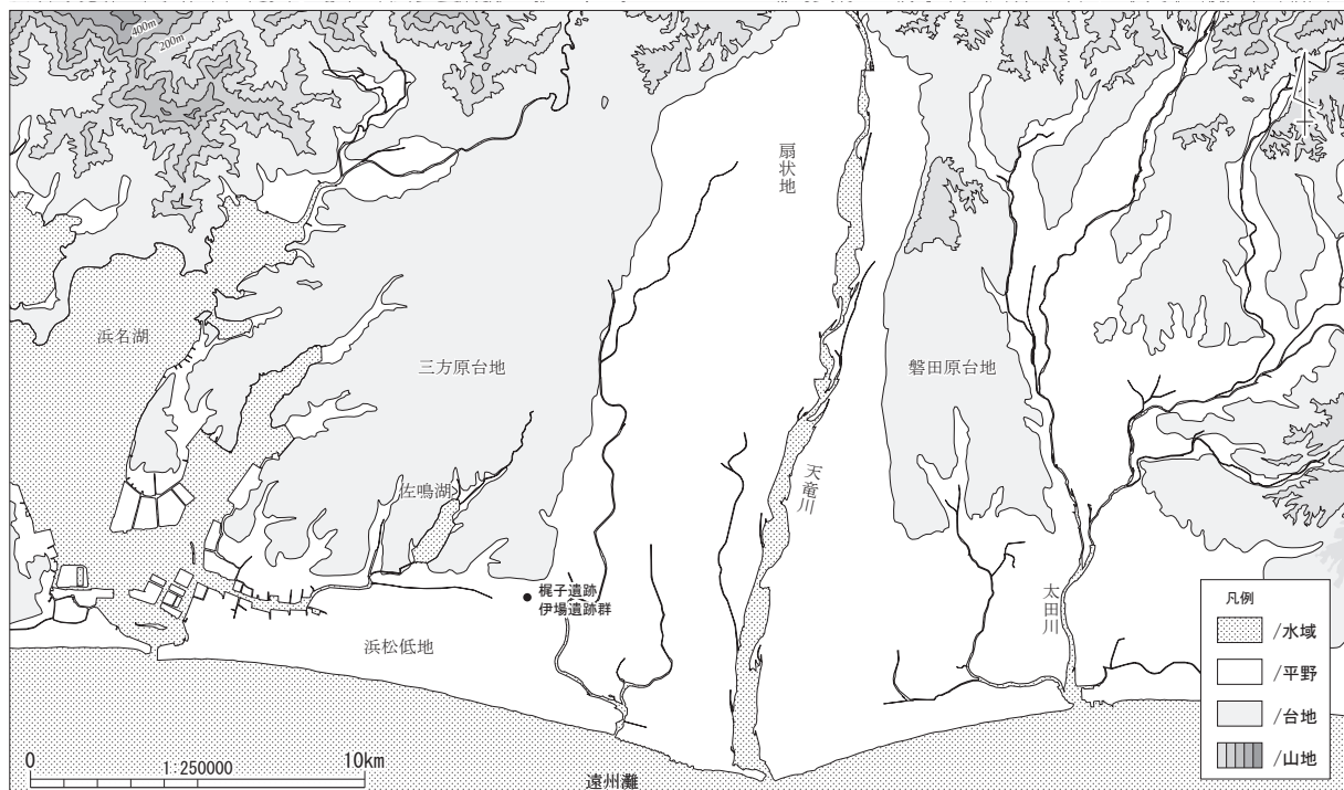
Fig. 5 浜松市南部の地形模式図
