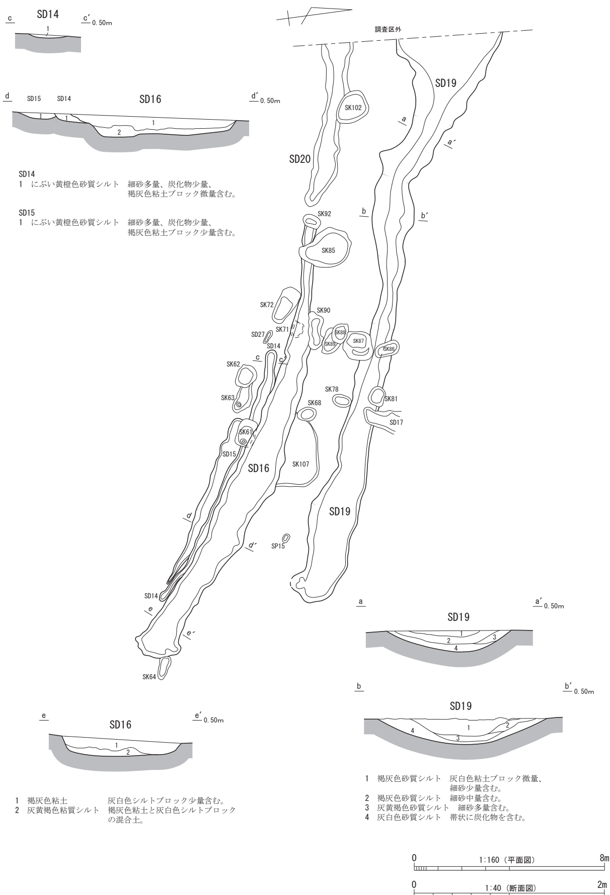
Fig. 21 A区 SD14～16・19 実測図
