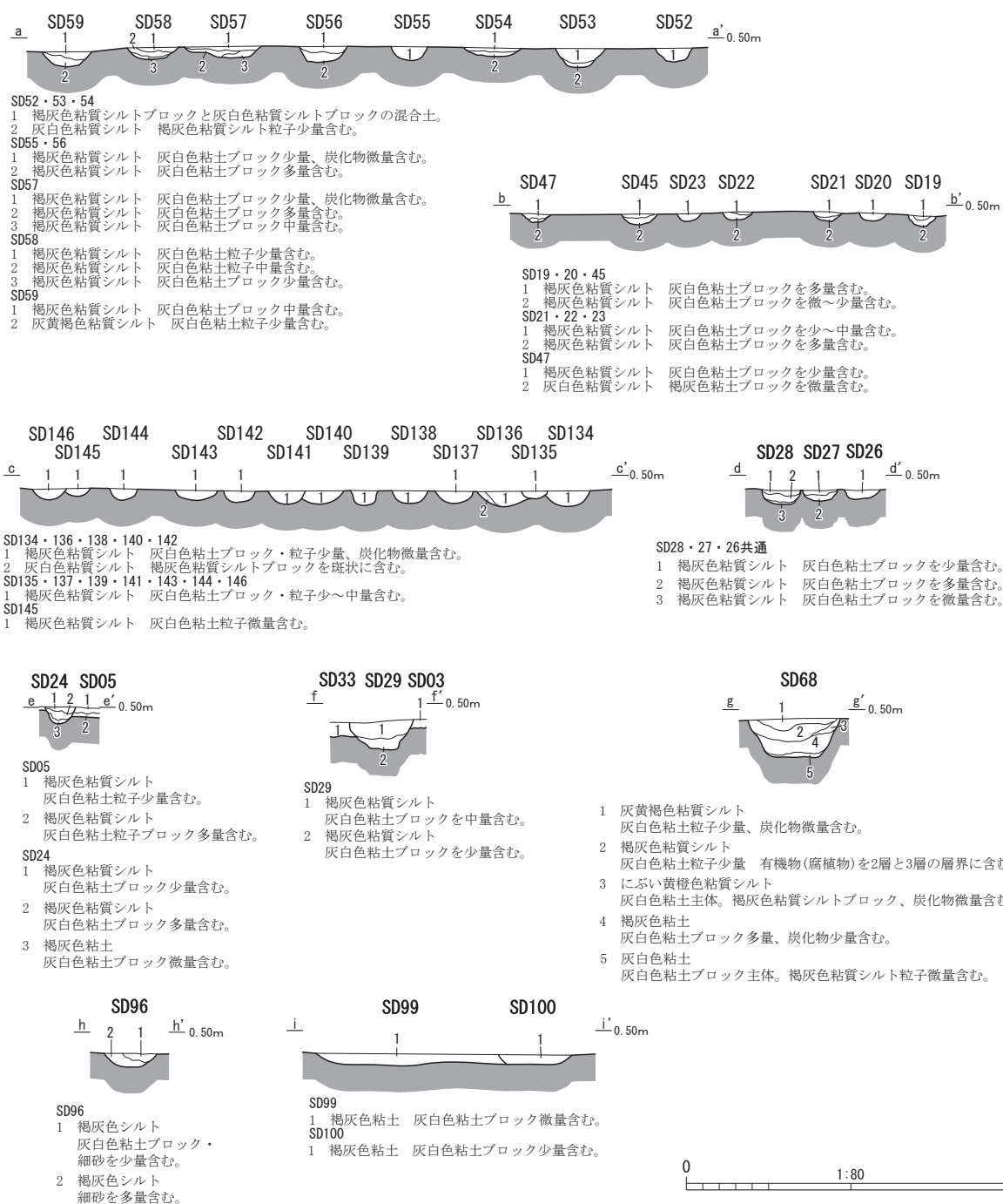
Fig. 57 SD03・05・19～24・26～29・33・45・47・52～59・68・96・99・100・134～146 実測図
