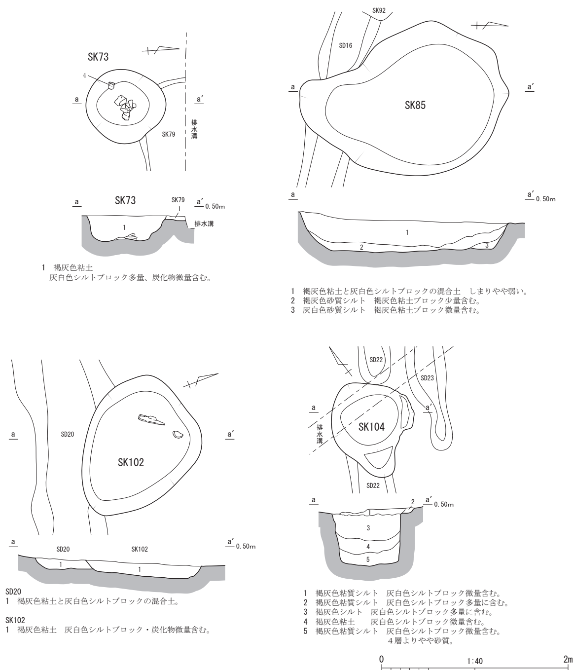
Fig. 25 A区 SK73・85・102・104 実測図
