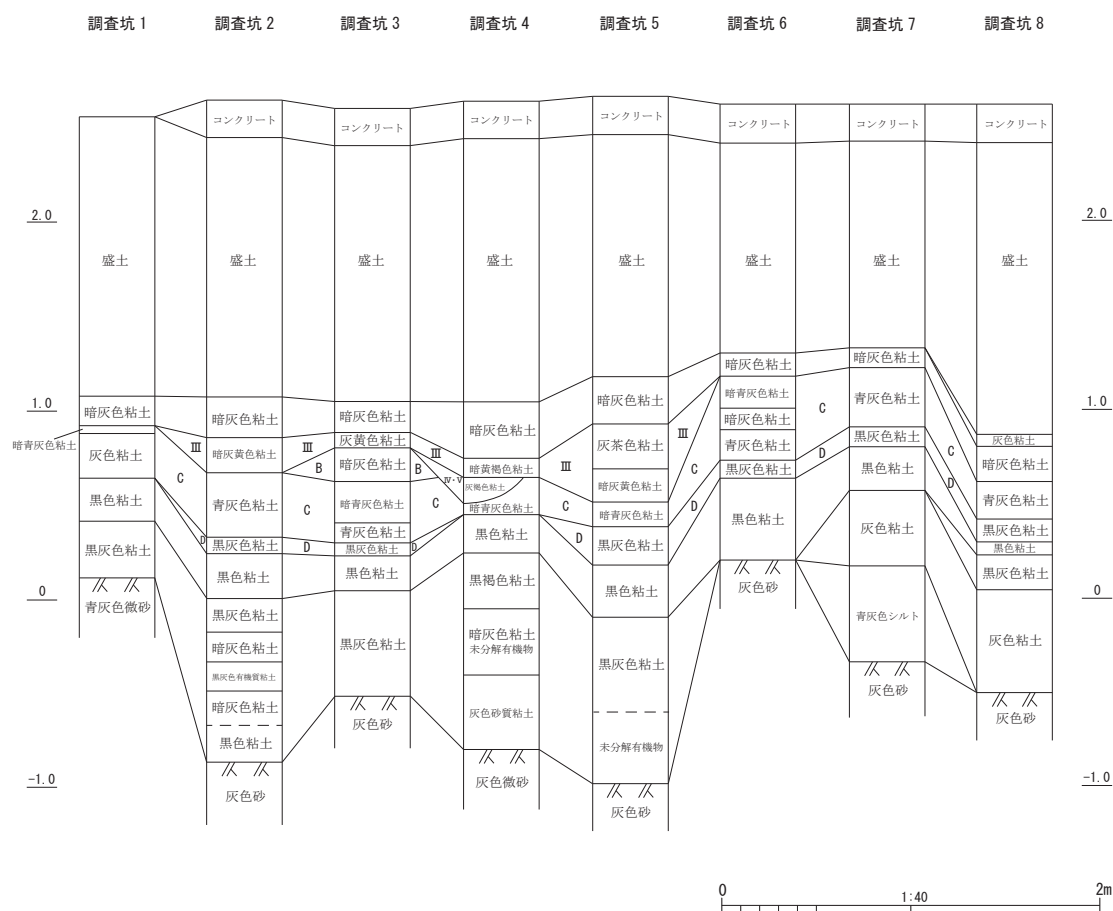
Fig. 13 確認調査土層柱状図
