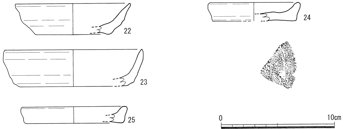
第17図 S01 出土遺物実測図 S=1/2
