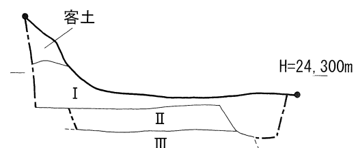
第5図 基本土層図（下段） S=1/40
