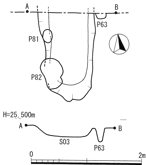
第10図 S03 実測図 S=1/40
