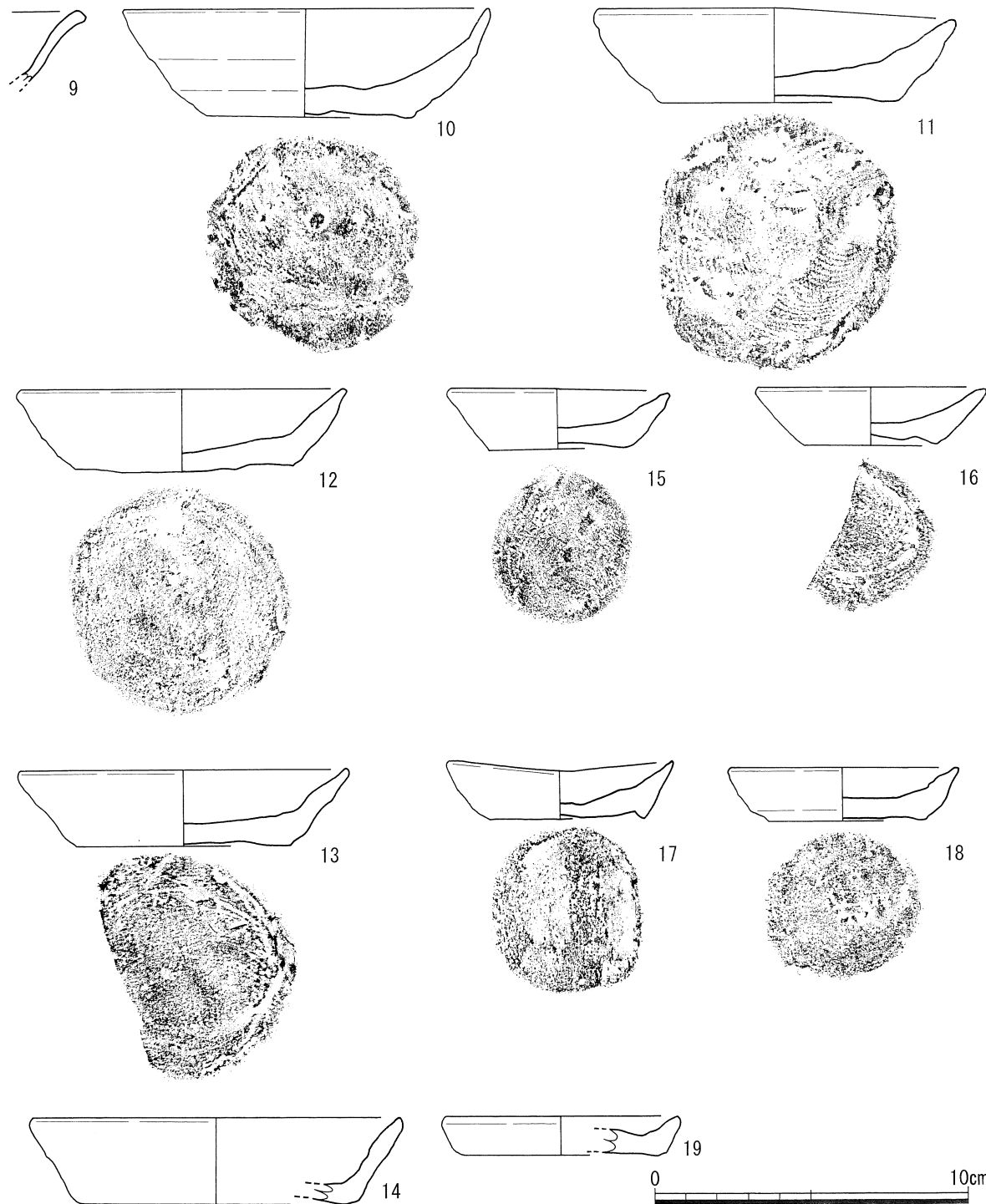
第 13 図 S07 出土遺物実測図 1 S=1/2
