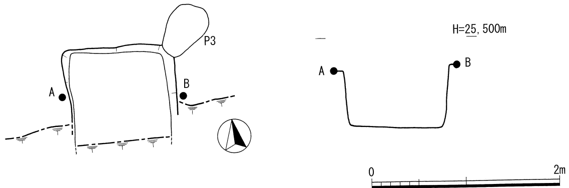
第8図 S02 実測図 S=1/40
