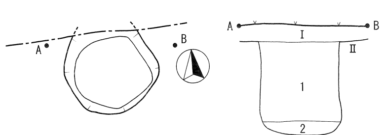
第 12 図 S07 実測図 S=1/40
