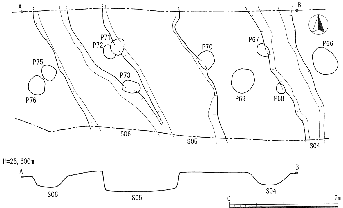
第18図 S04・S05・S06 実測図 S=1/40
