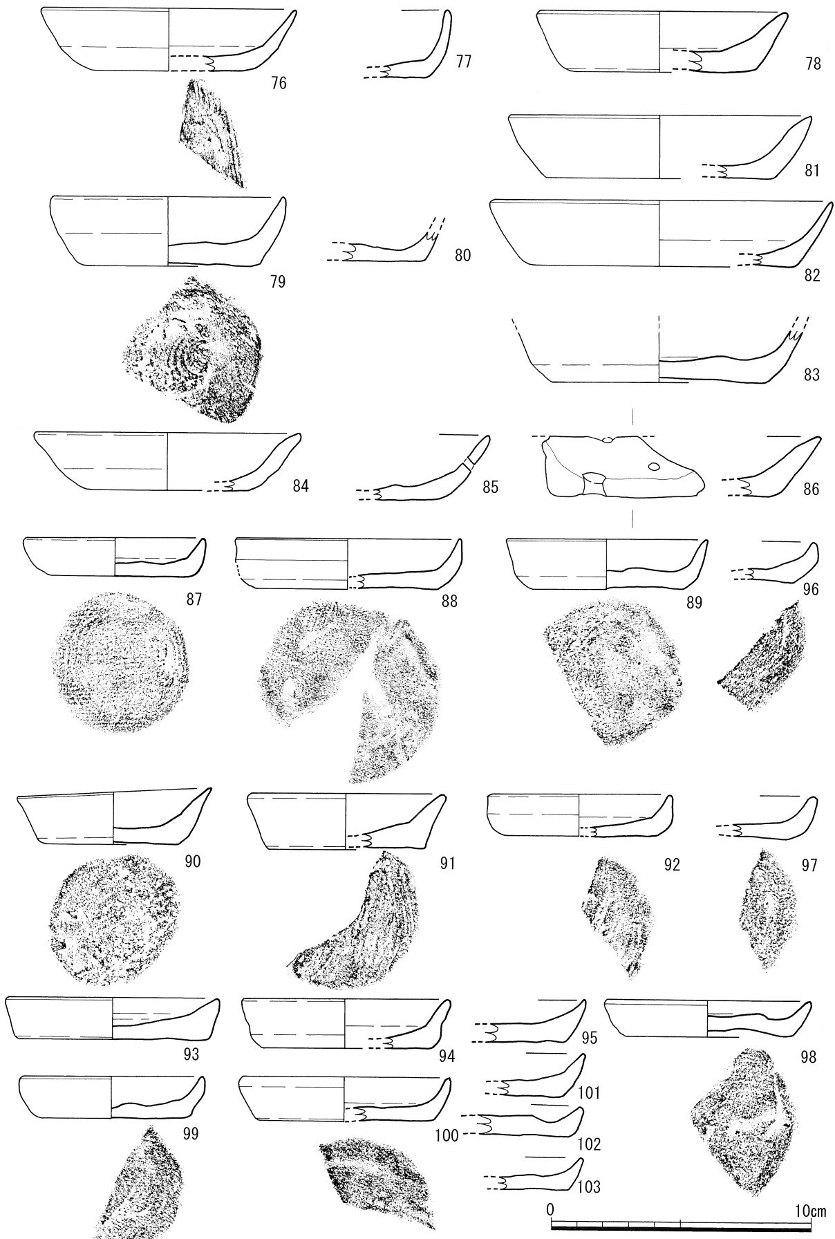
第 25 図 遺構外出土遺物実測図 2 S=1/2
