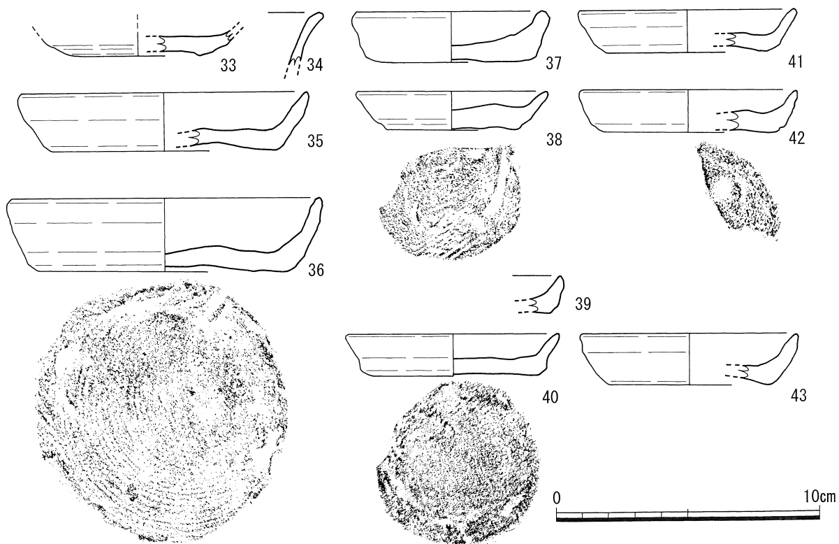
第 22 図 小穴内出土遺物実測図 1 S=1/2
