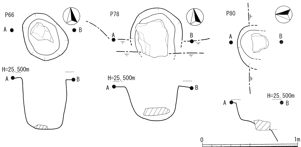
第 21 図 P66・P78・P80 実測図 S=1/20
