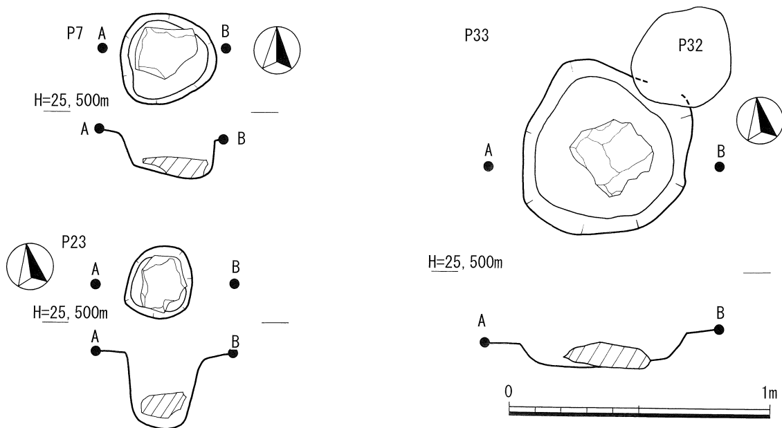
第 20 図 P7・P23・P33 実測図 S=1/20
