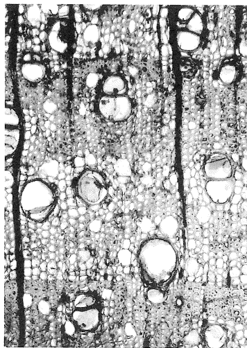
横断面 ————— : 0.5mm
