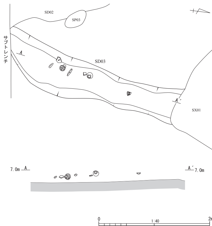
Fig. 15 SD03 詳細図
