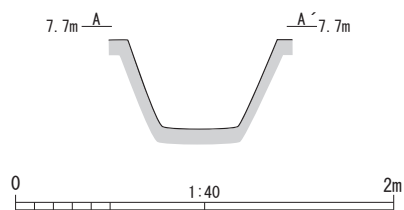
Fig. 22 SX03 詳細図
