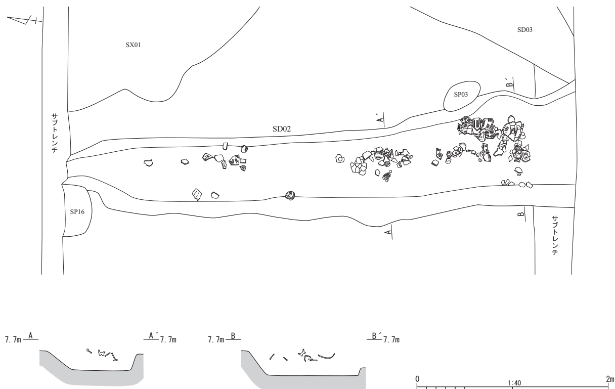
Fig. 12 SD02 詳細図
