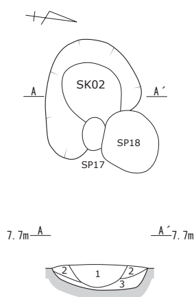
SK02 土層断面図
