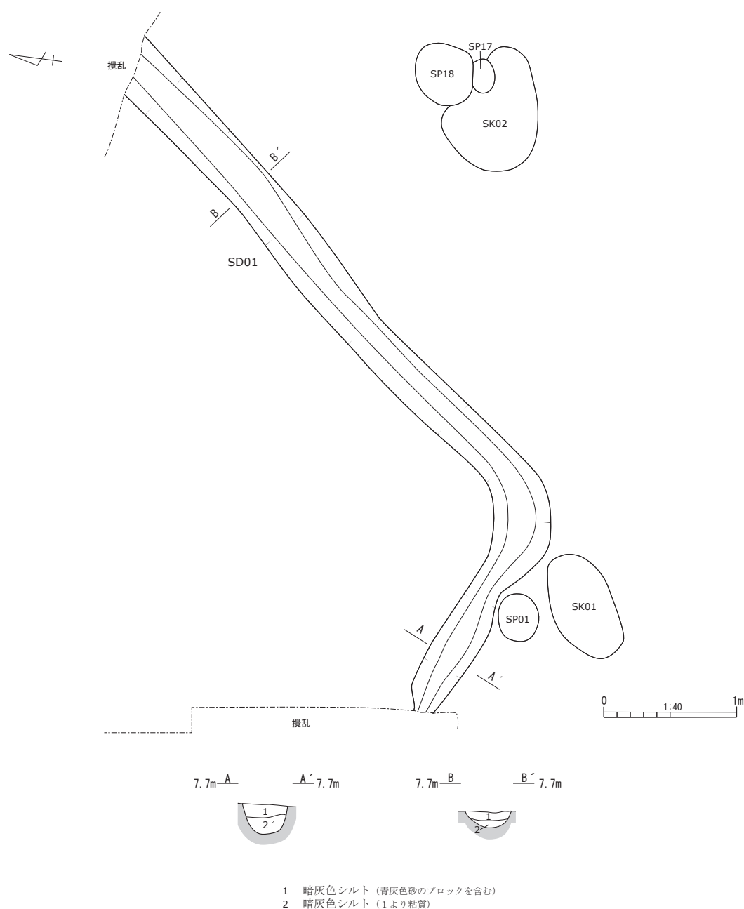
Fig. 11 SD01 詳細図
