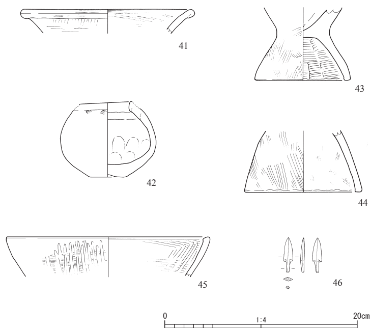
Fig. 15 SD03 詳細図
