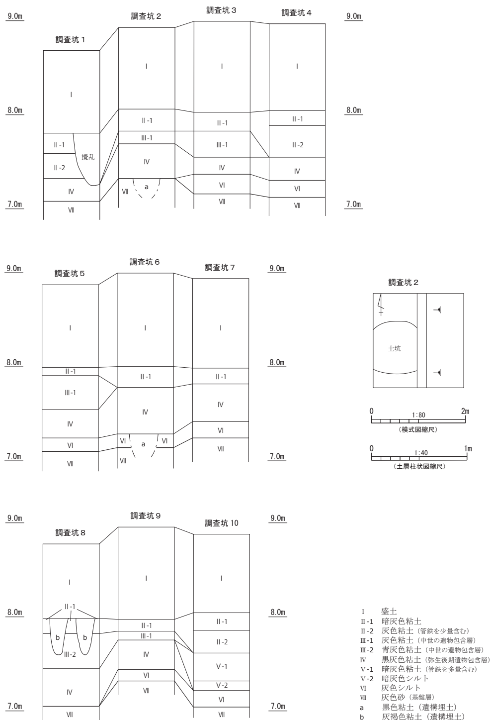
Fig. 6 確認調査 (3 次調査) における土層柱状図及び調査坑 2 平面模式図
