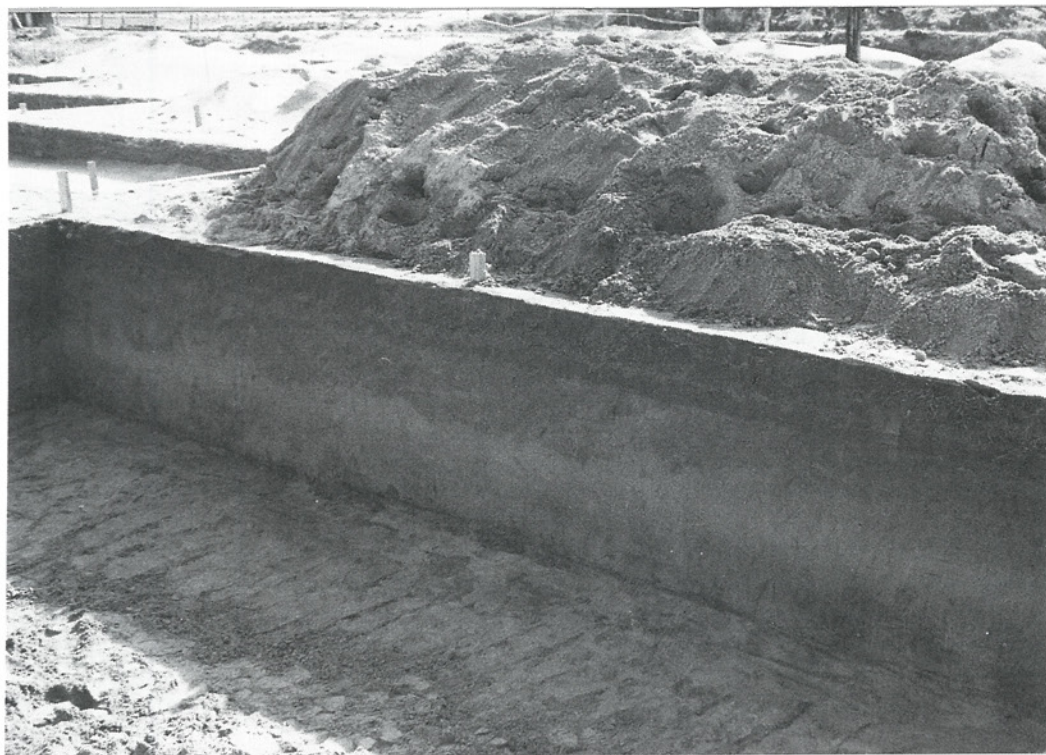
第16区層序
