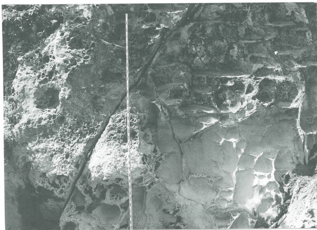
第16区海蝕痕
