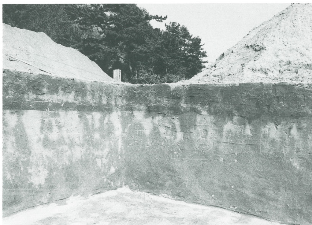
第16区層序
