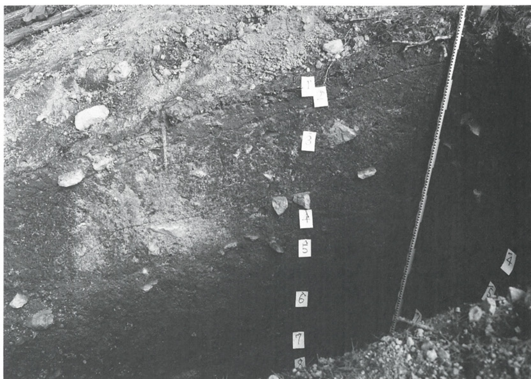
第28区層序
