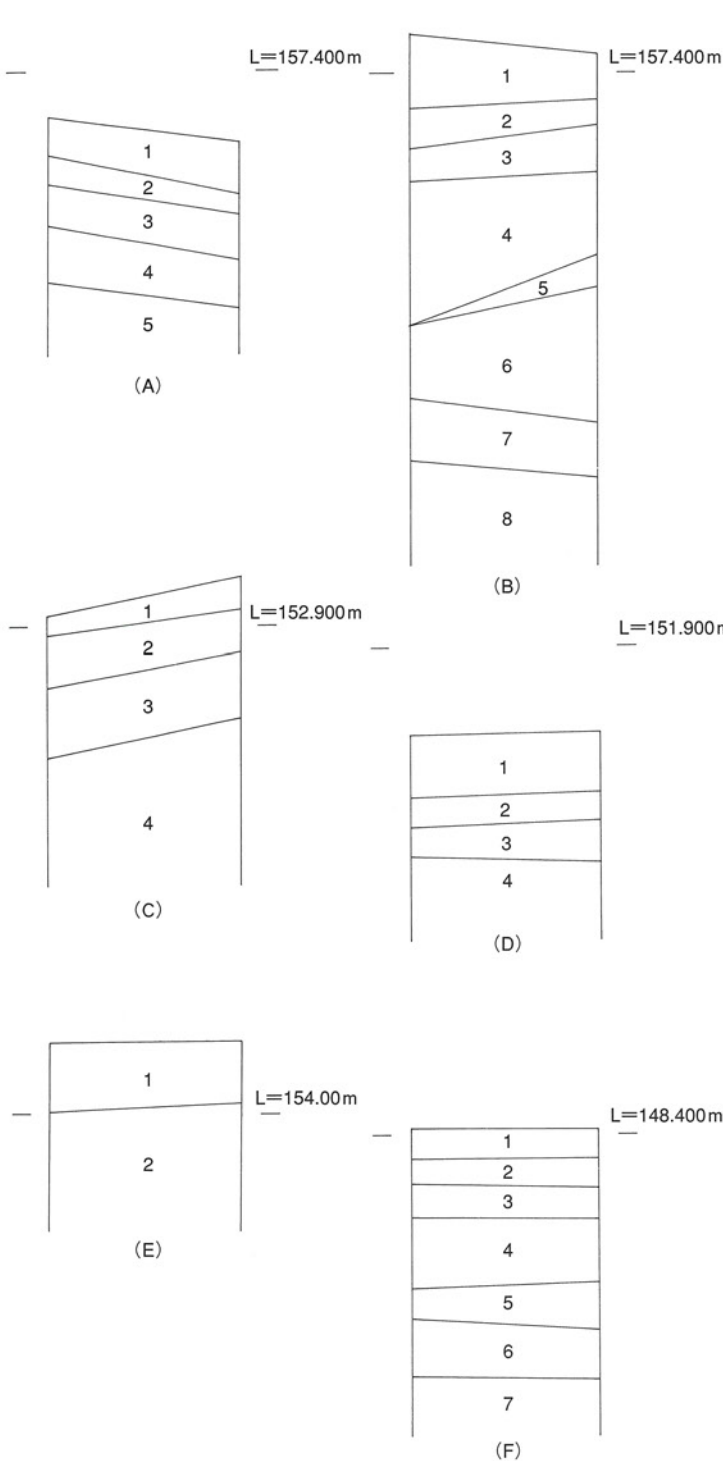
第4図 基本土層柱状図
