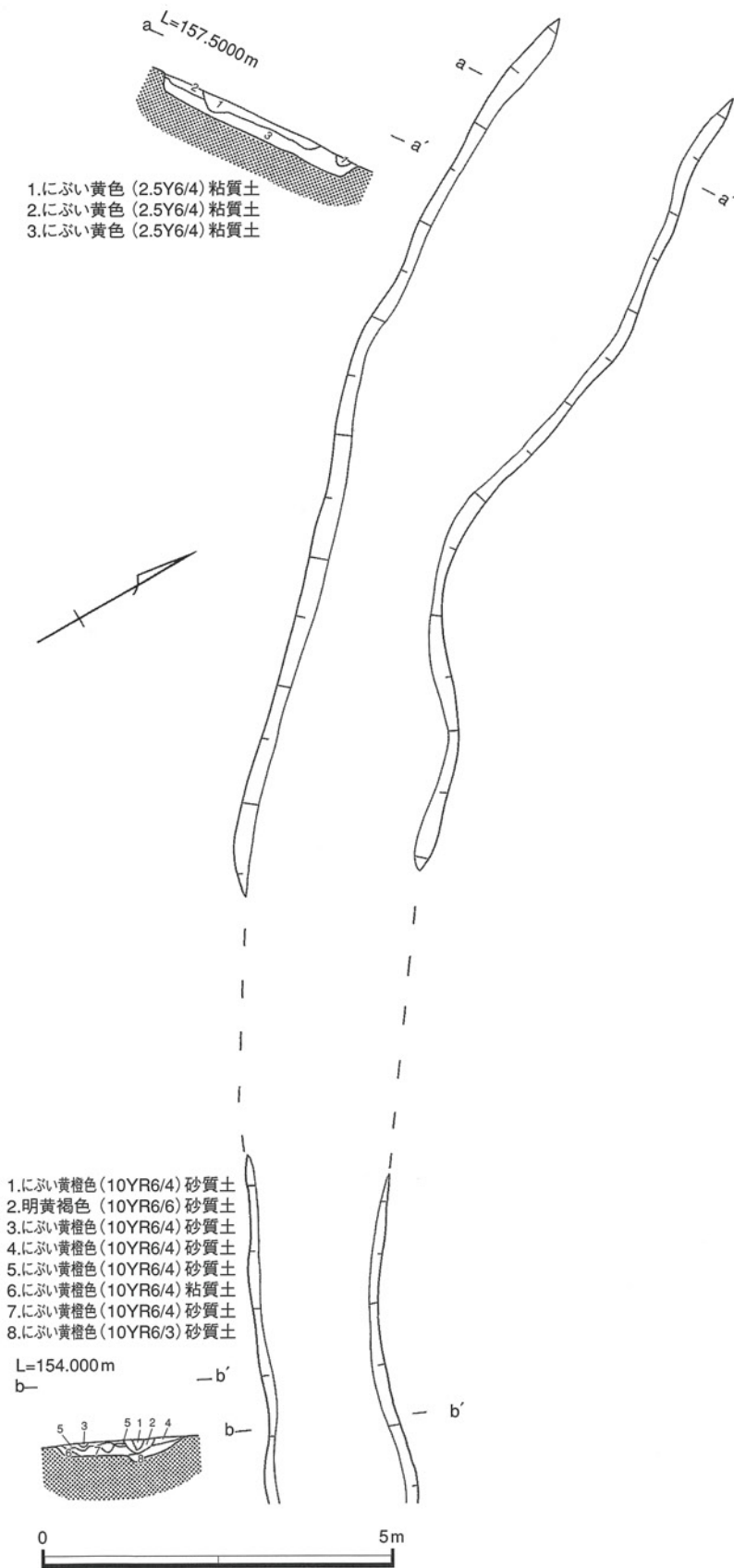
第18図 SD1013 遺構図
