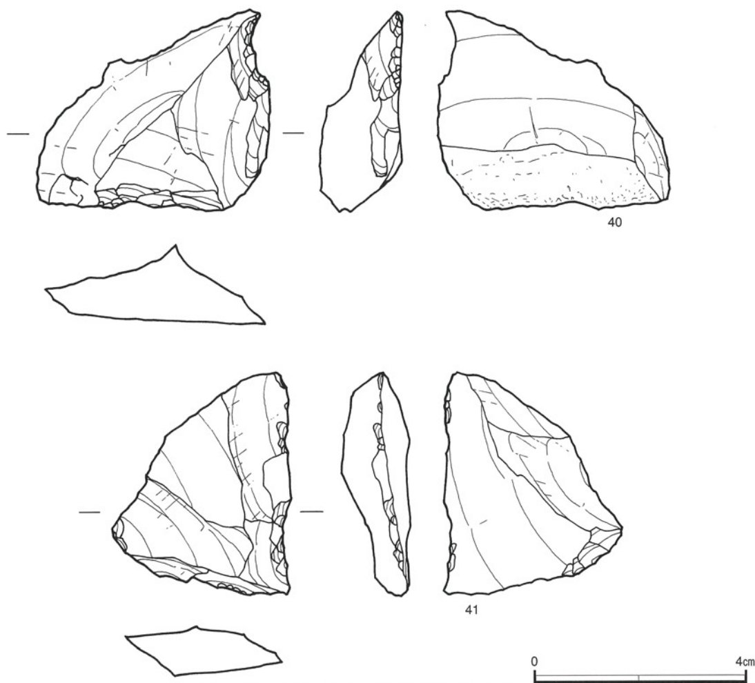
第58図 第3ブロック出土石器 (4)
