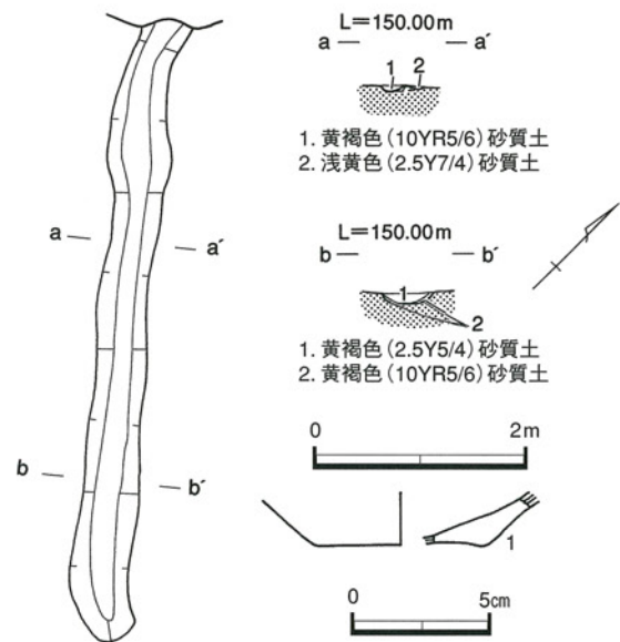
第8図 SD1001 遺構図・出土遺物
