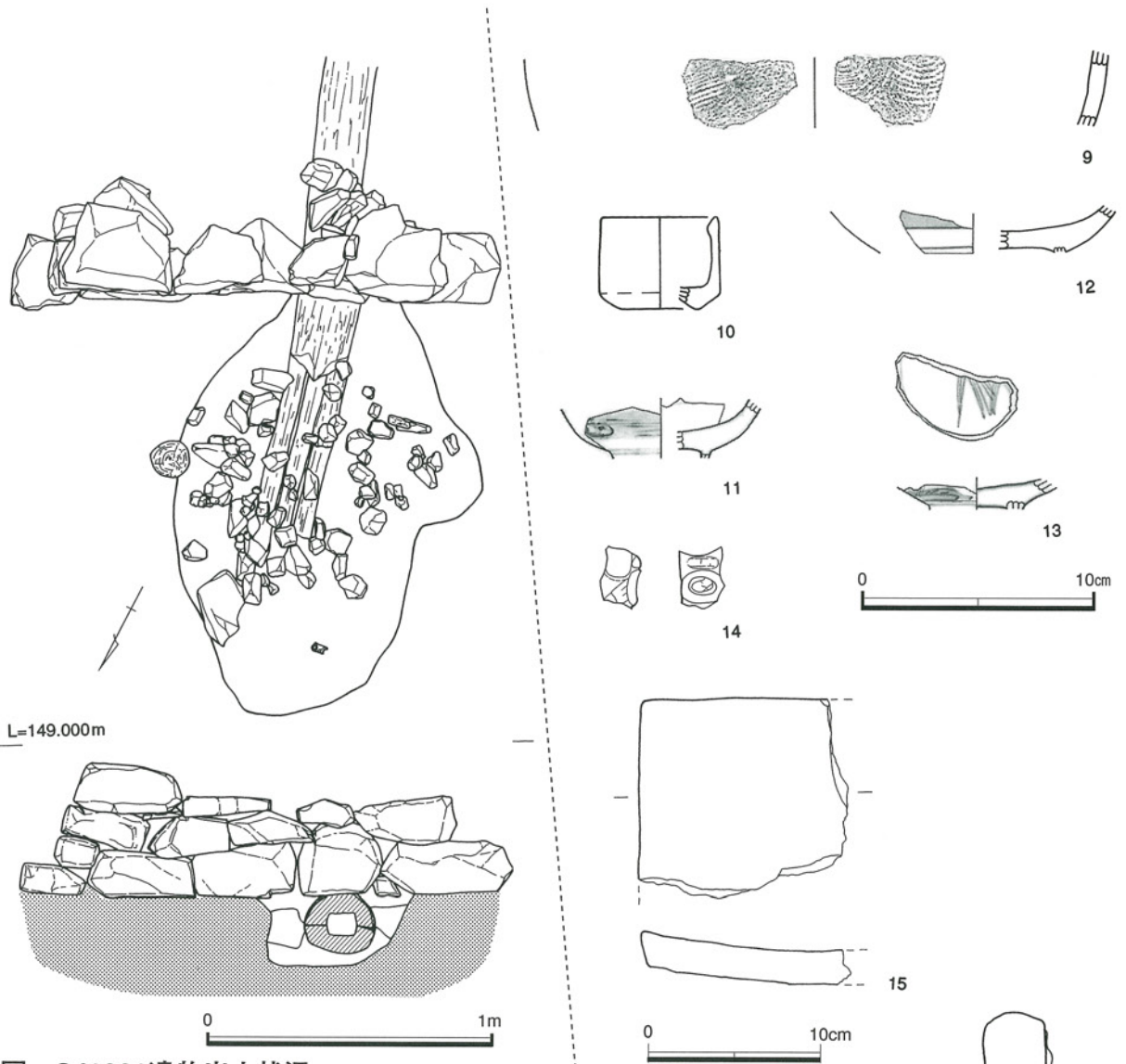
第33図 SJ1001遺物出土状況
