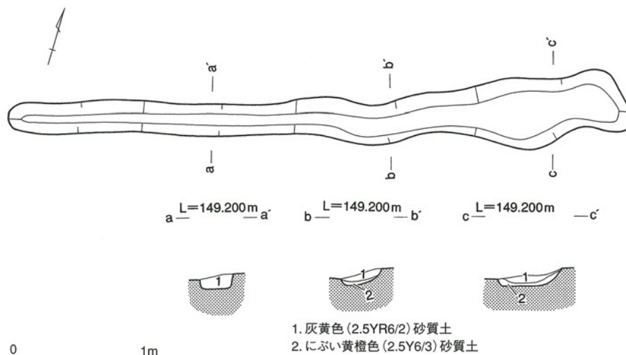
第9図 SD1002 遺構図
