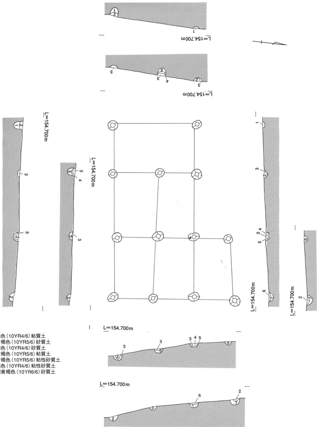
第6図 SA1002 遺構図
