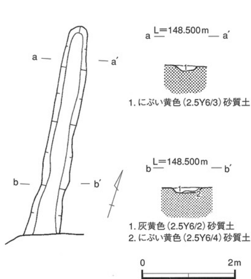
第10図 SD1003 遺構図
