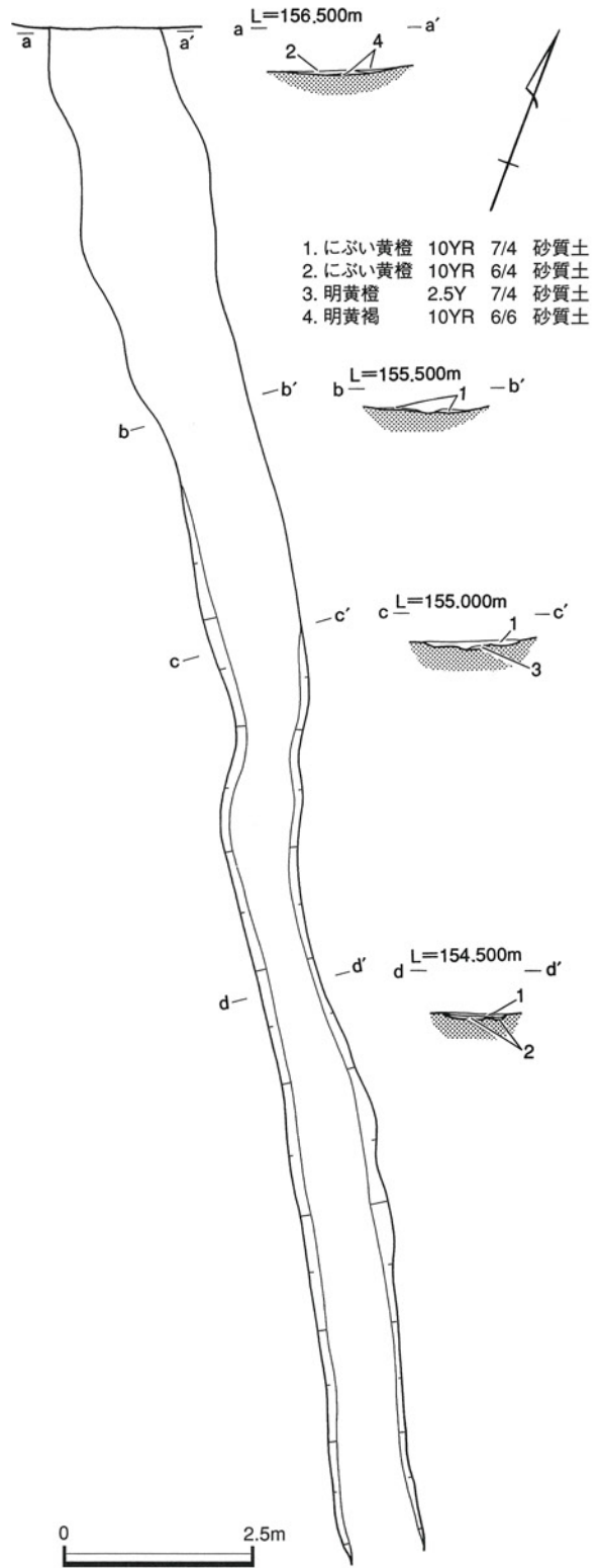
第14図 SD1008 遺構図
