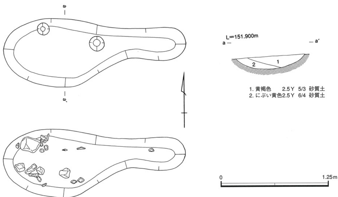
第26図 SK1012 遺構図
