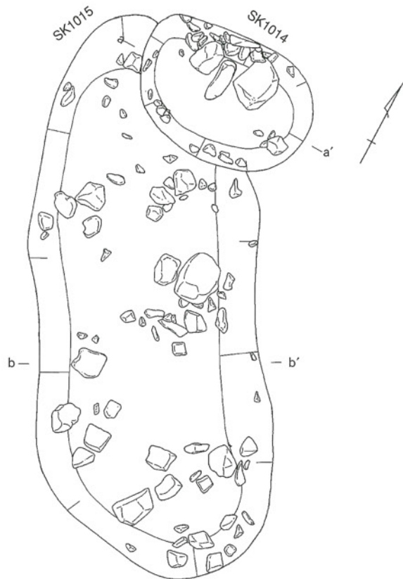
第28図 SK1014.1015 遺構図
