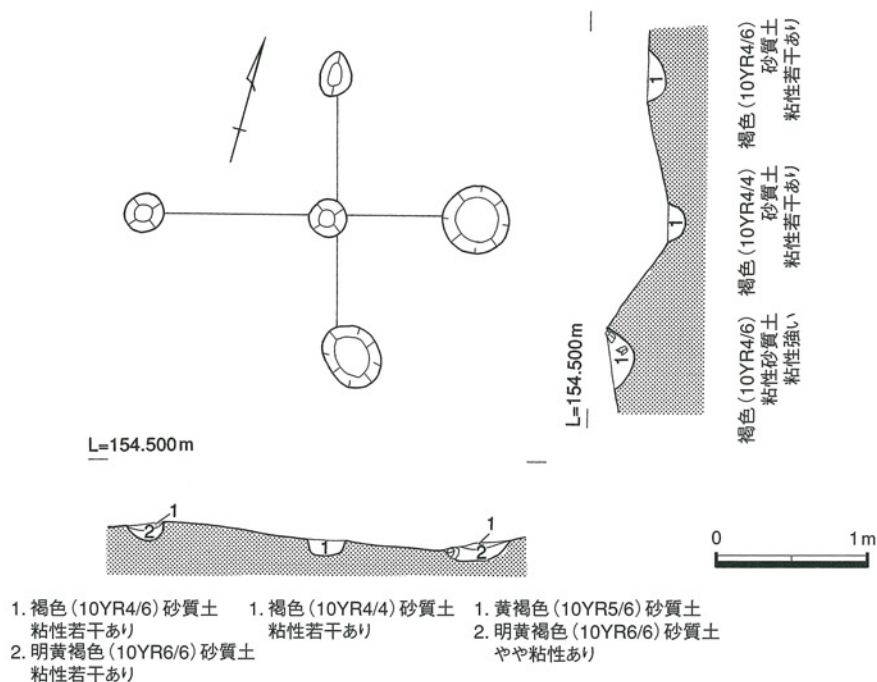
第5図 SA1001 遺構図
