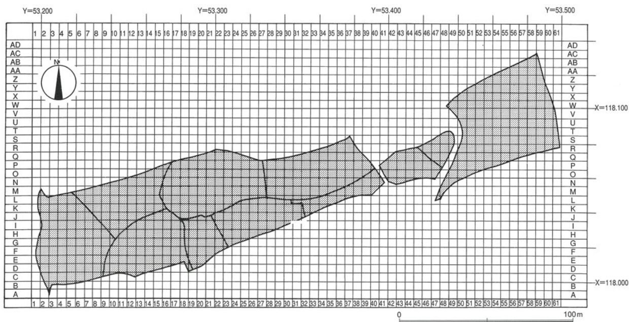
第2図 坊僧地区グリッド配置図
