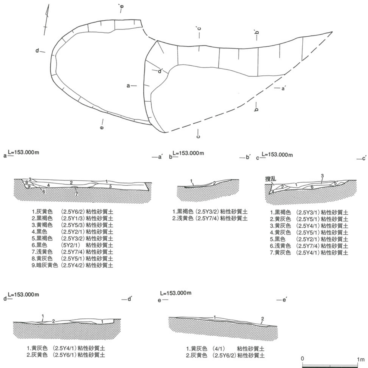
第36図 SO1003. 1004 遺構図
