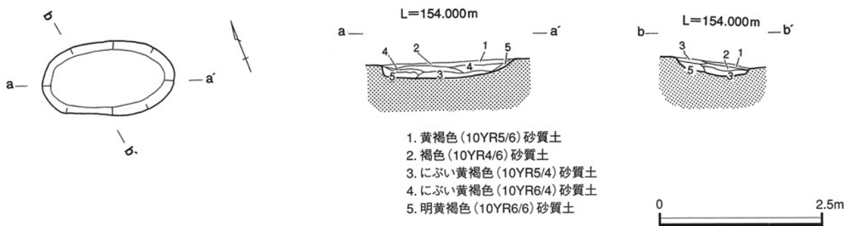
第25図 SK1010 遺構図
