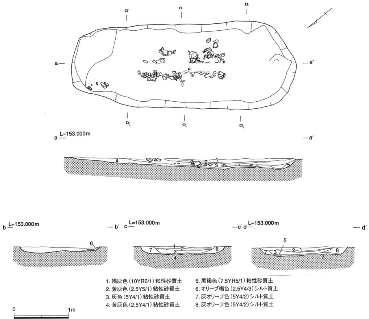
第35図 SO1002 遺構図
