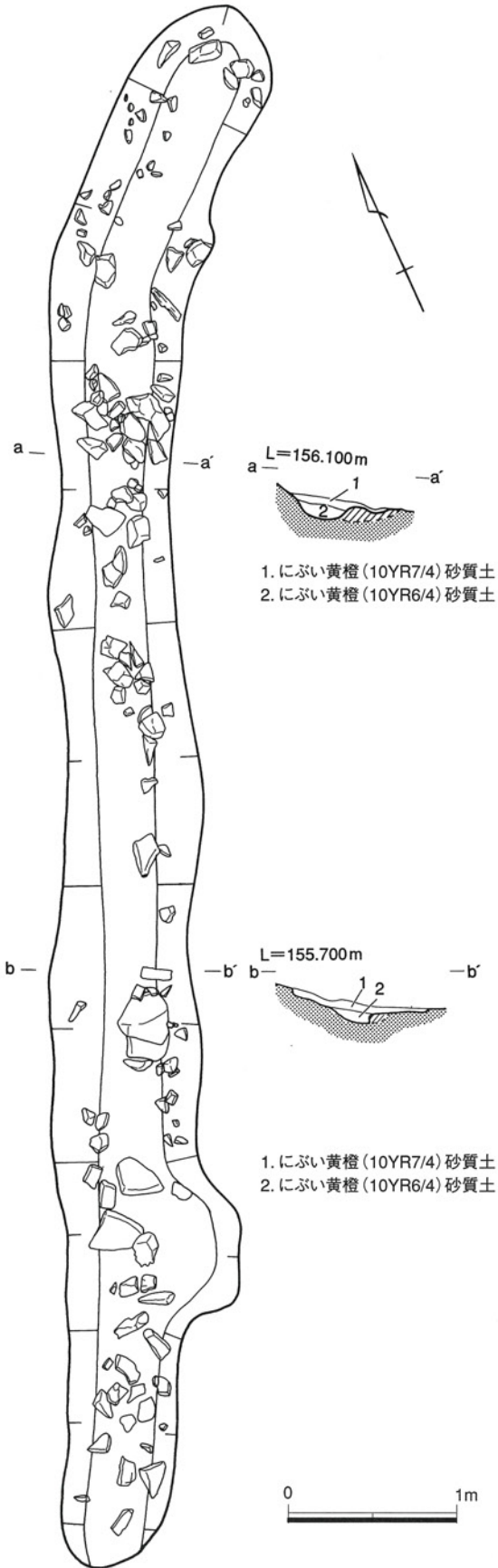
第13図 SD1007 遺構図
