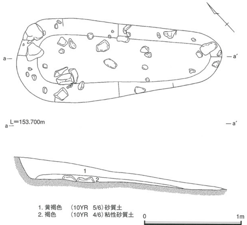
第27図 SK1013 遺構図
