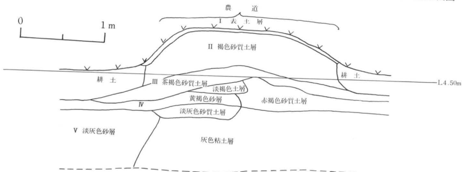
第6トレンチ南壁断面図
