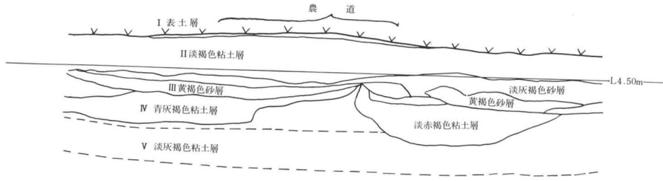
第1トレンチ北壁断面図
