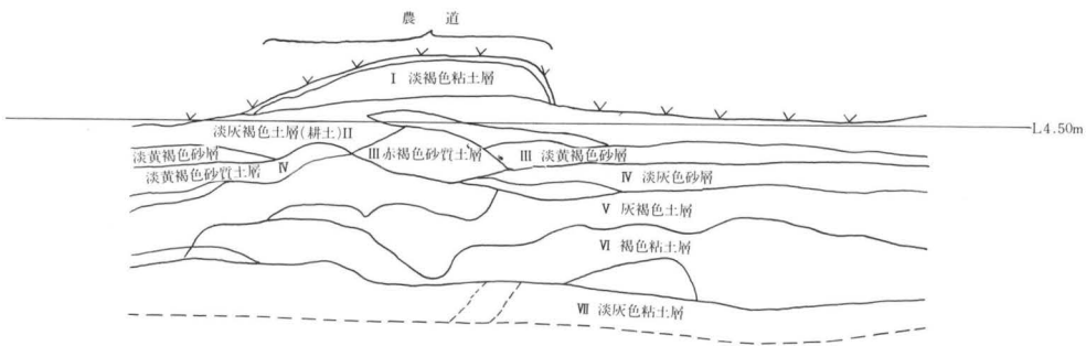
第5トレンチ北壁断面図
