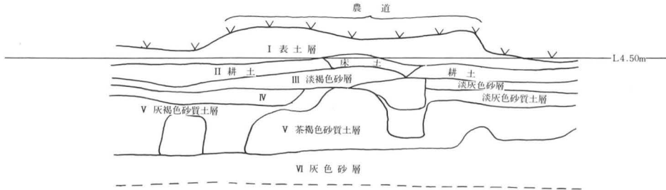
第2トレンチ東壁断面図
