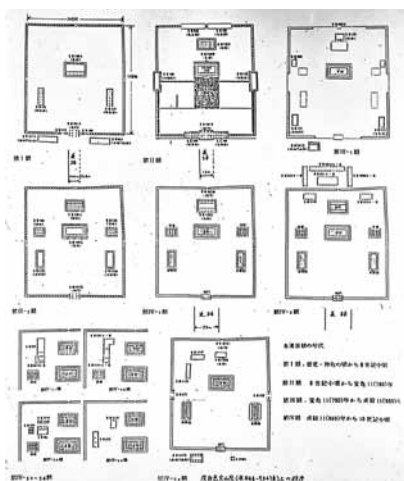
図4 多賀城跡・政庁第I～IV期変遷図
