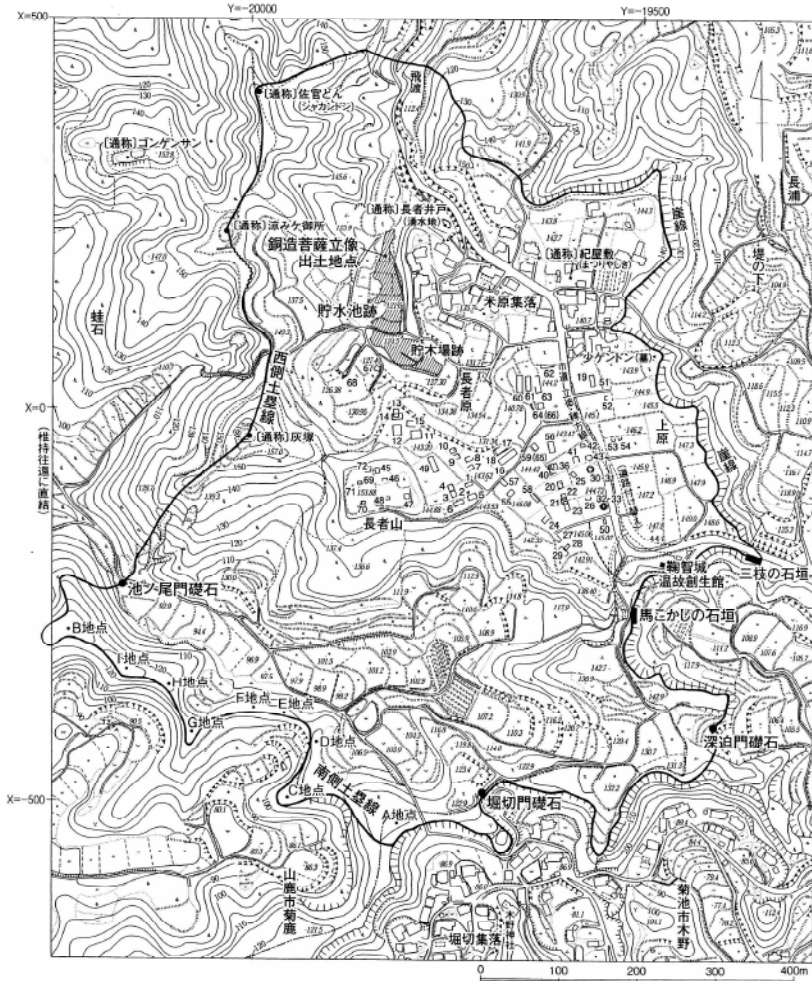
第1図 鞠智城跡
